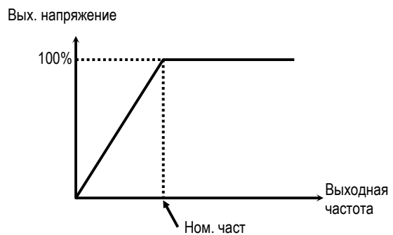
[Линейная U/F-характеристика]
