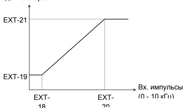
[Зависимость задания скорости от частоты входных импульсов]
