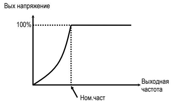
[Квадратичная U/F-характеристика]
