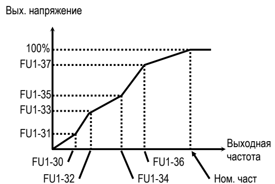
[U/F-характеристика пользователя]
