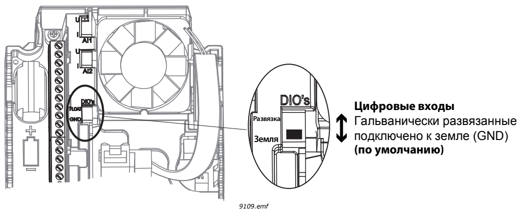
Рис. 103. DIP-переключатель изоляции
