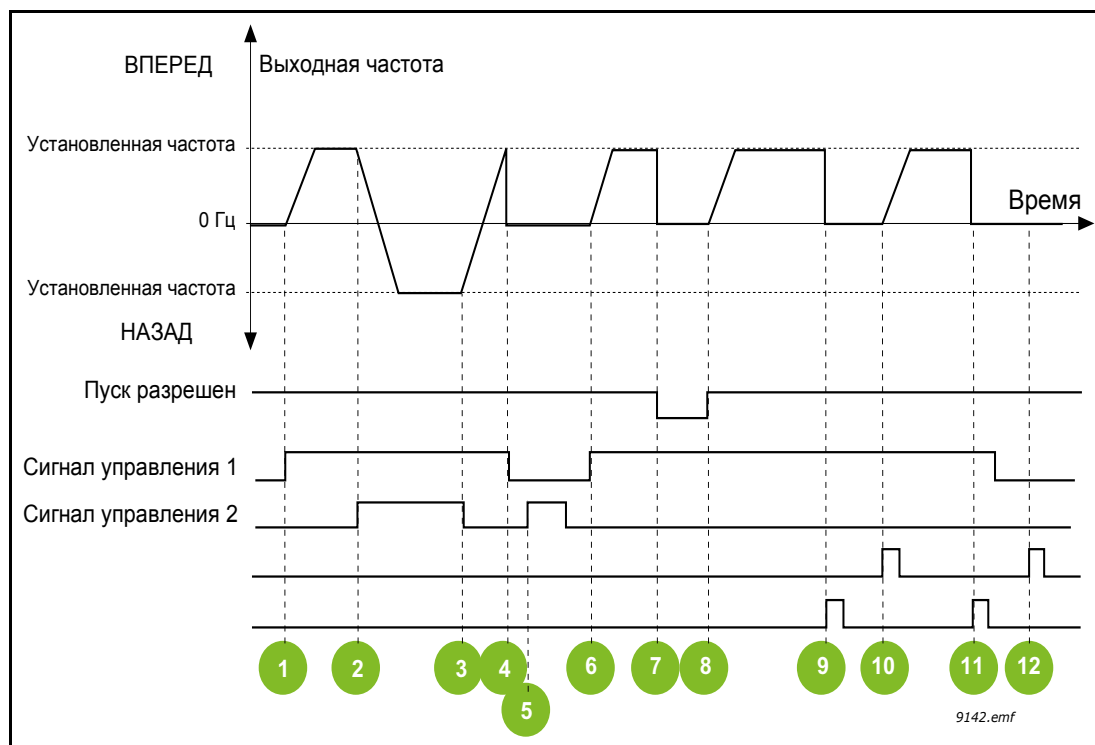
Рис. 53. Логика пуска/останова I/O A = 3
