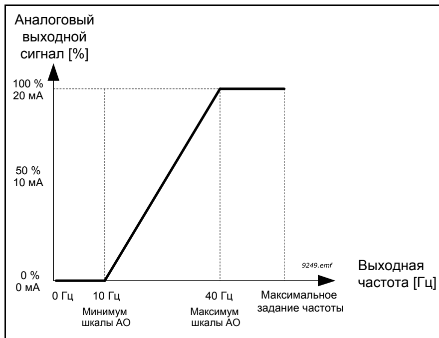
Рис. 71. Масштабирование сигнала АО1
