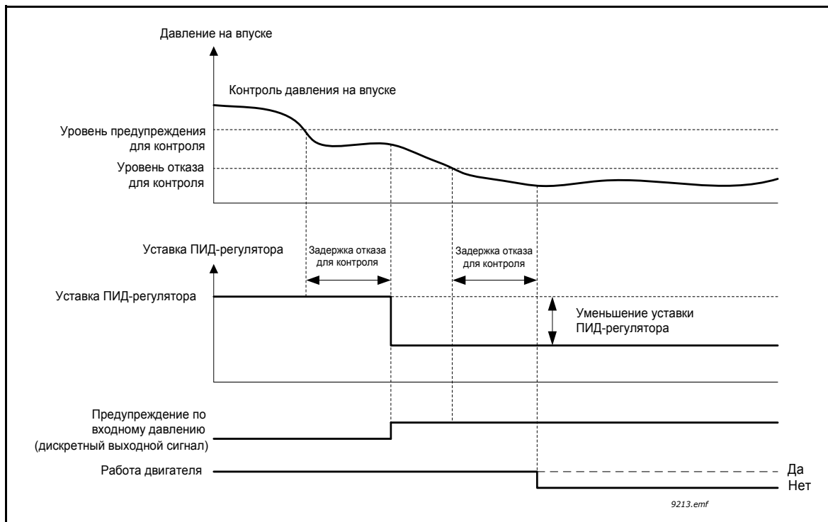
Рис. 94. Контроль входного давления
