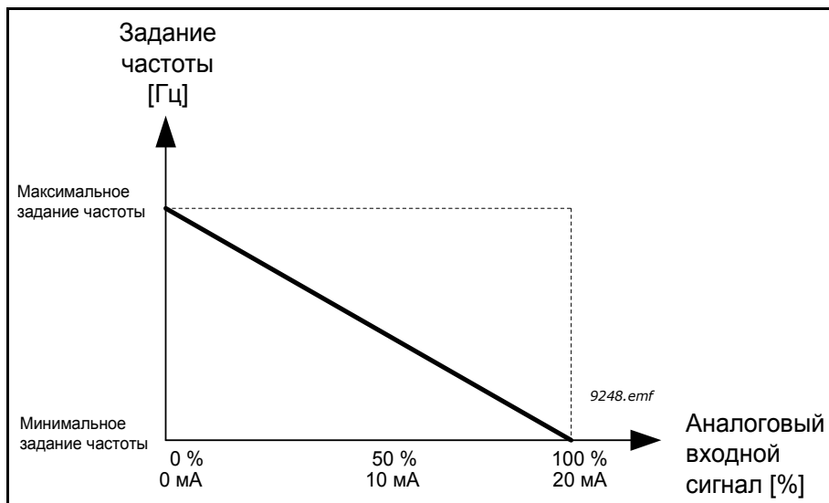
Рис. 70. Инверсия сигнала AI, вариант 1
