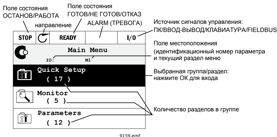
Рис. 21. Главное меню
