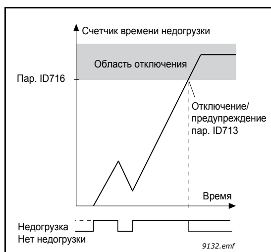
Рис. 79. Функция счетчика времени недогрузки, ИД 713 = Р3.9.4.1 Отказ из-за недогрузки, ИД 716 = Р3.9.4.4 Защита от недогрузки: предел времени
