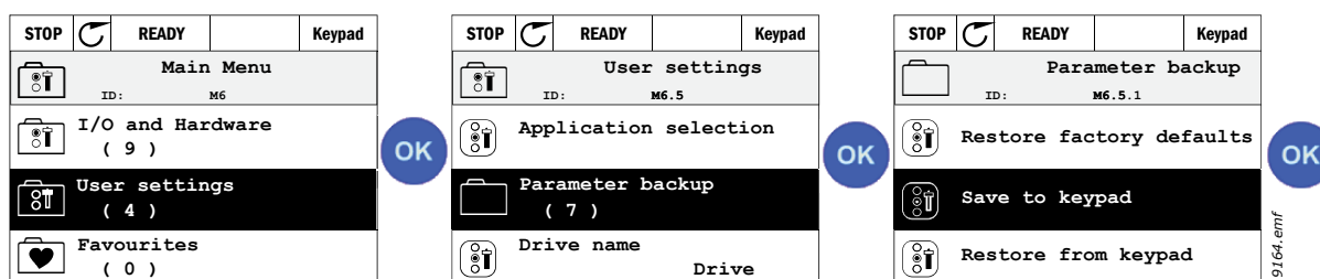
Рис. 28. Копирование параметров
