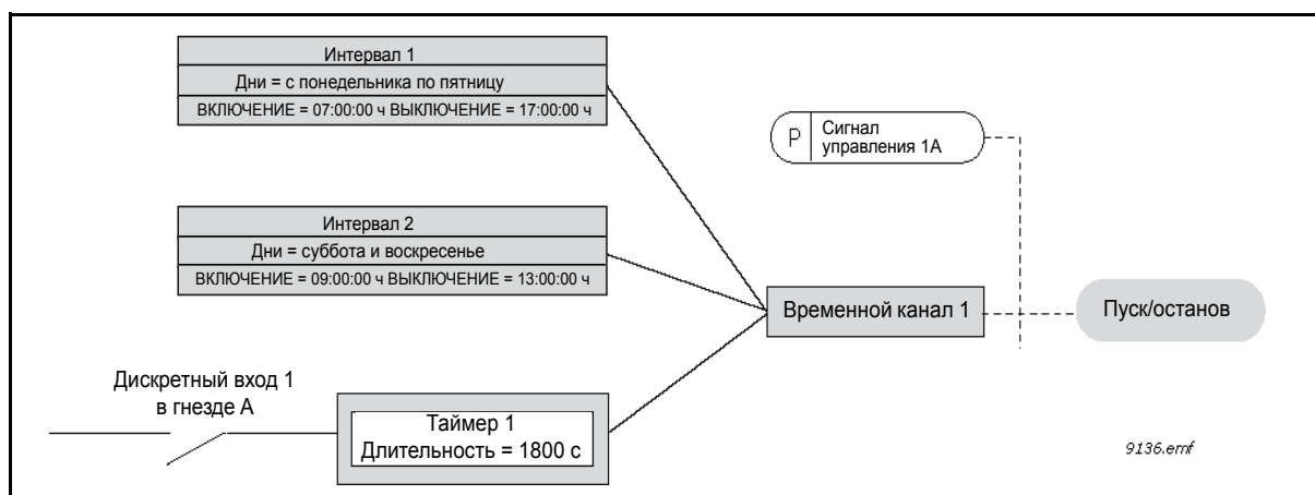
Рис. 84. Окончательная конфигурация, в которой временной канал 1 используется с целью формирования сигнала управления для команды пуска вместо дискретного входа.
