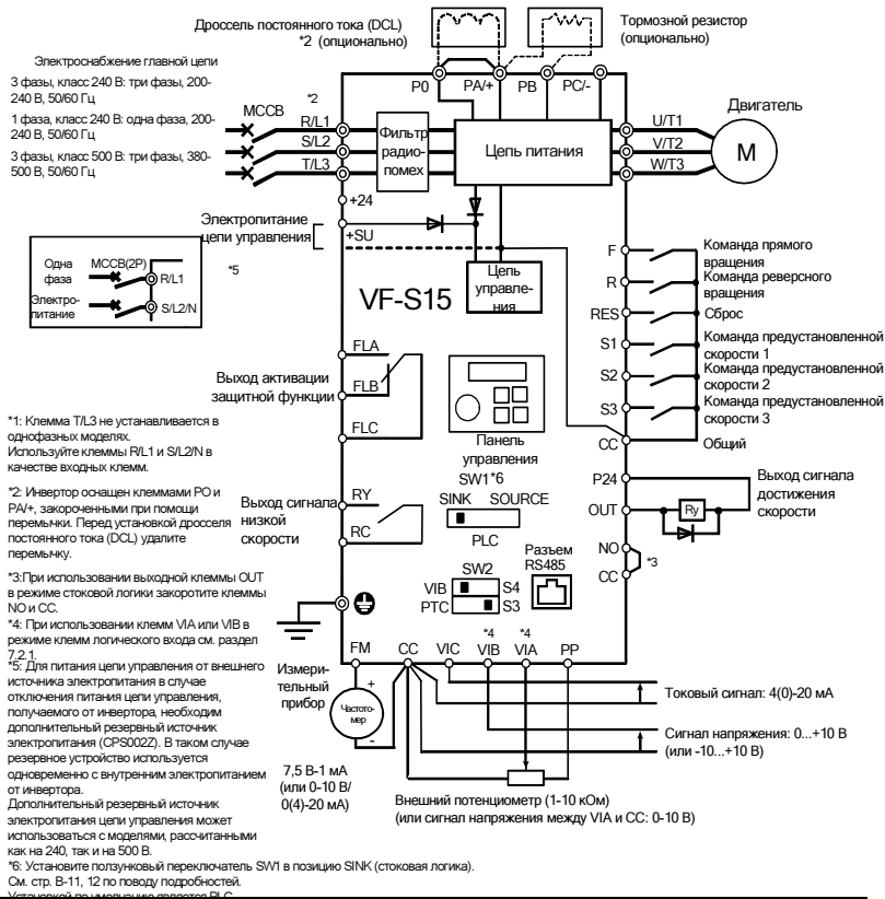
Схема стандартного подключения - SINK (стоковая логика) (общий: CC)
