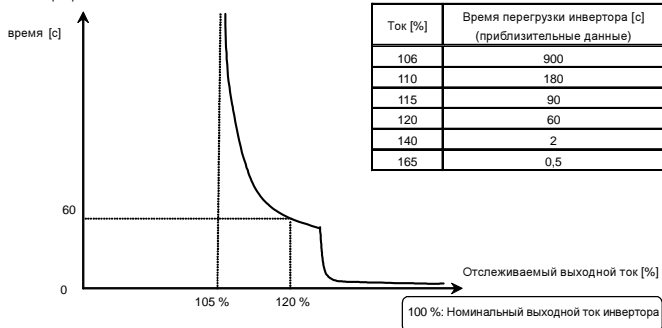
Характеристика защиты инвертора от перегрузки
