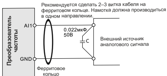
Рисунок 3-8. Схема подключения проводов к входной клемме аналогового сигнала
