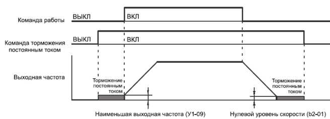
Временная характеристика режима торможения постоянным током
