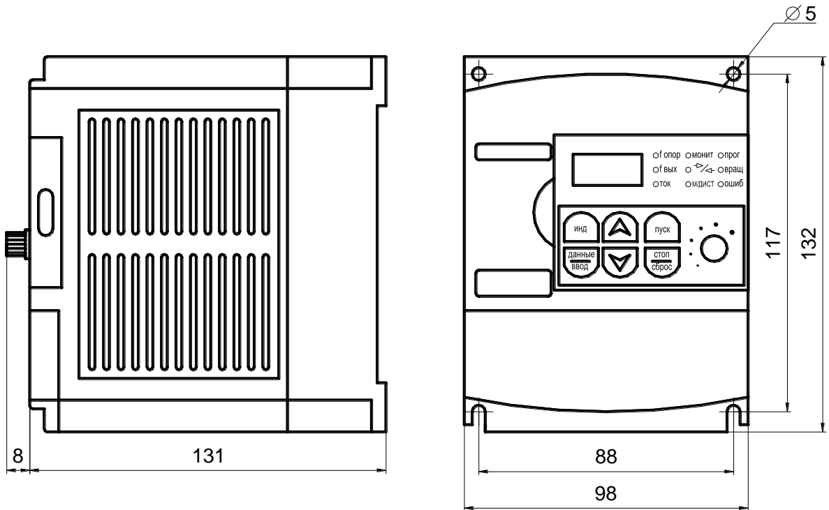
Преобразователь E3-8100B-002H
