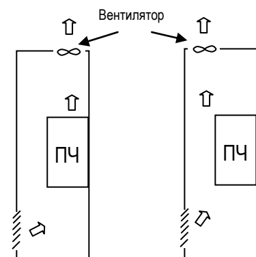
Размещение в шкафу (вид сбоку)
