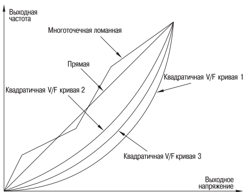
Рисунок 30 – V/F-кривые
