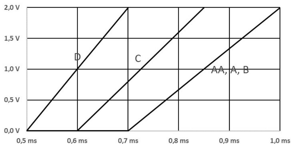
Корректировка напряжения для длинных тестовых импульсов OSSD
