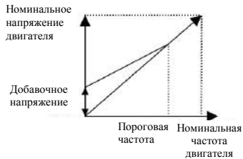
б Кривая постоянного момента при форсировании момента
