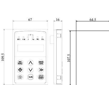
Рис.2-7 Монтажные размеры пульты управления
