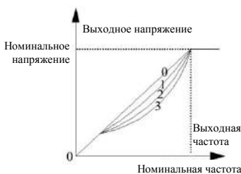
Рис. 7-7 а V/F-кривая
