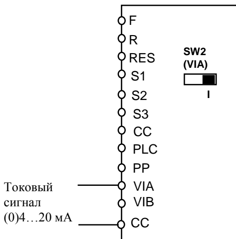
(3) Задание частоты внешним сигналом (0)4...20 мА (только вход VIA)
