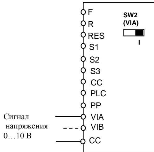
(2) Задание частоты внешним сигналом 0...10 В
