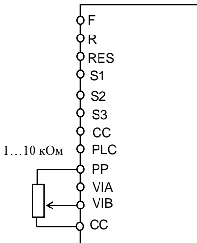
(1) Задание частоты внешним потенциометром
