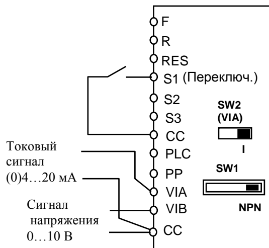
(4) Переключение задания частоты: “токовый сигнал / сигнал напряжения” внешним сигналом
