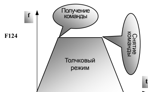
Рис 5-1 Толчковый режим
