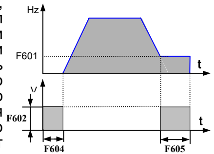
Рис 5-9 Торможение
