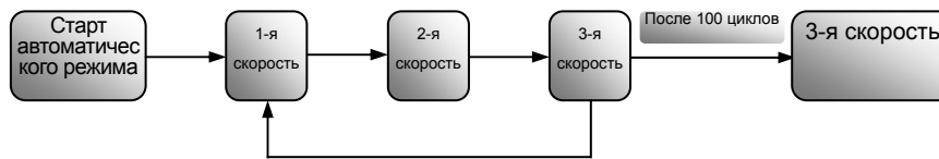
Рис 5-7 Автоматический режим
