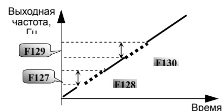
Рис 5-2 Пропуск частоты
