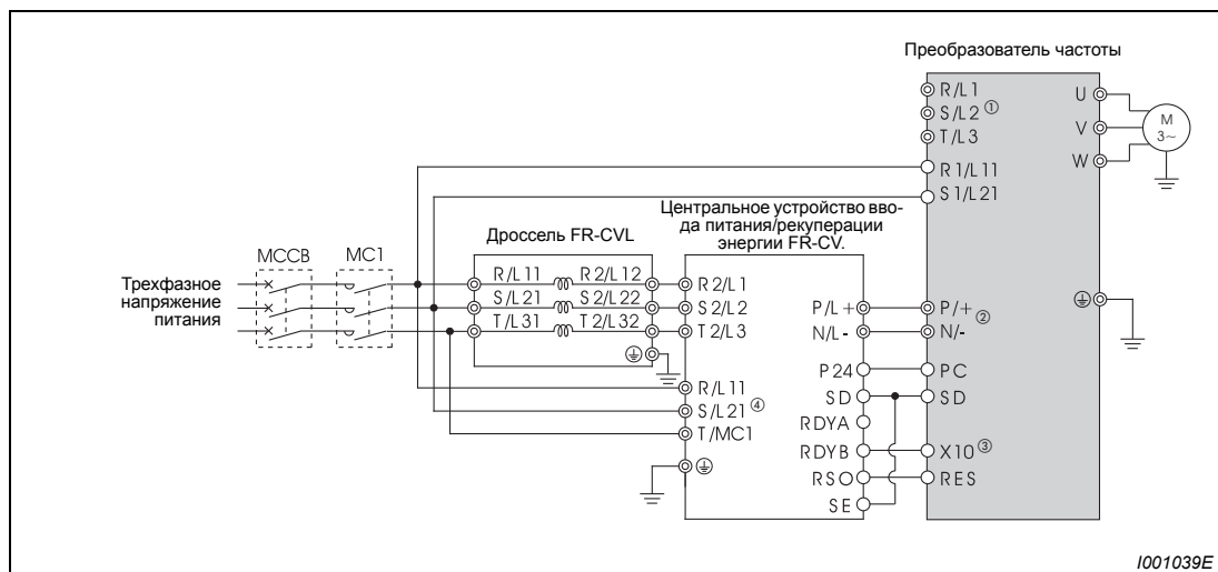
Рис. 3-32: Подключение комбинированного устройства рекуперации энергии/сетевого фильтра FR-FC
