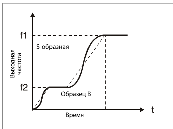
Рис. 6-35: Характеристика при пар. 29 = "2"
