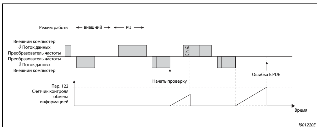
Рис. 6-149: Контроль кабеля на разрыв
