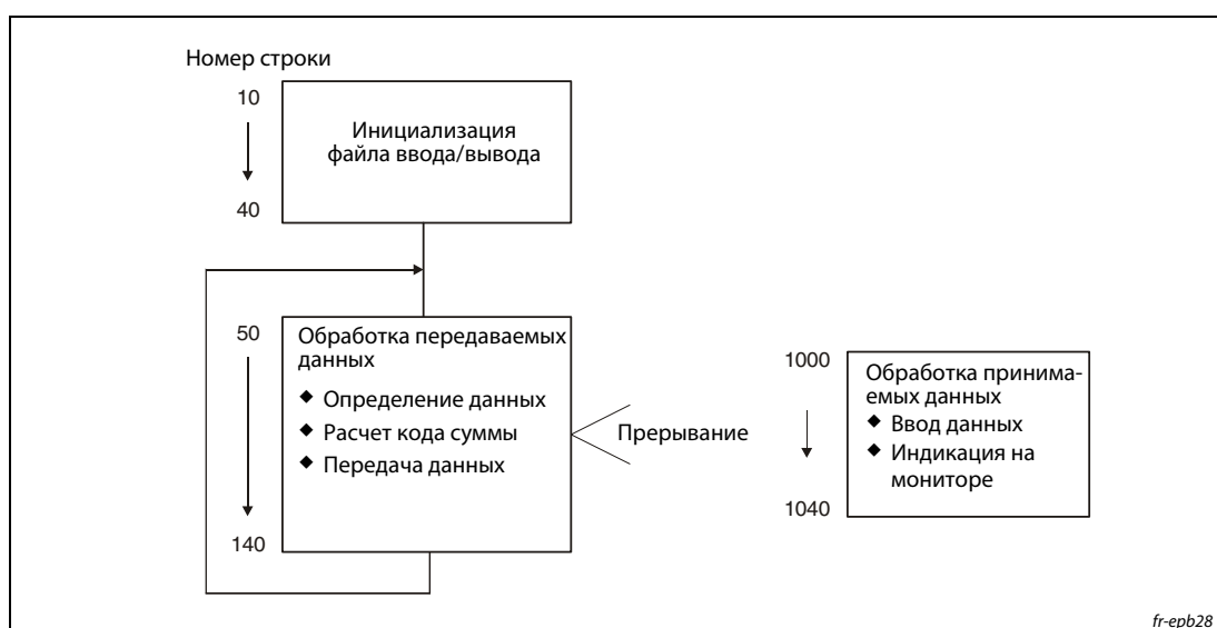
Рис. 6-151: Общая схема последовательности действий
