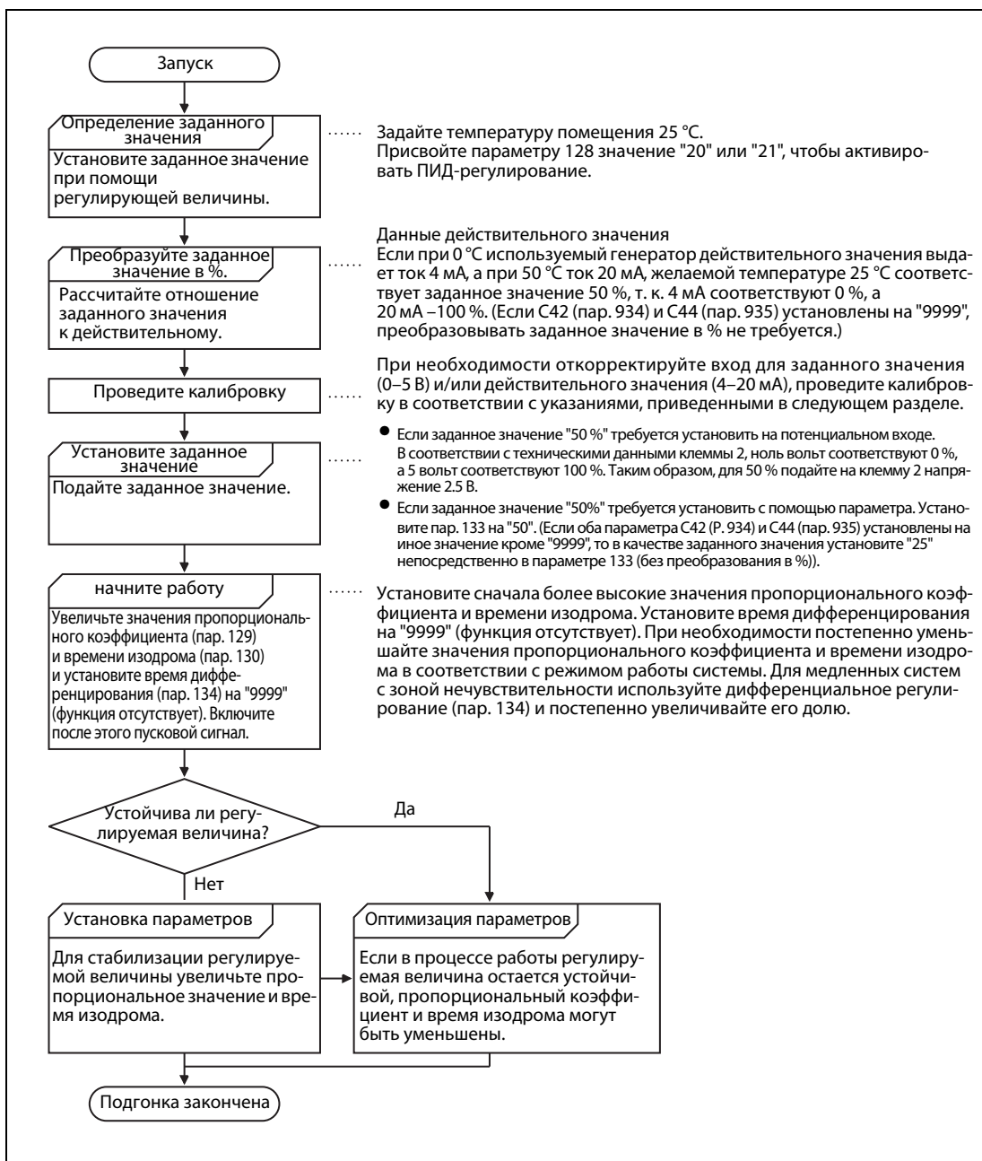
Рис. 6-169: Пример подгонки
