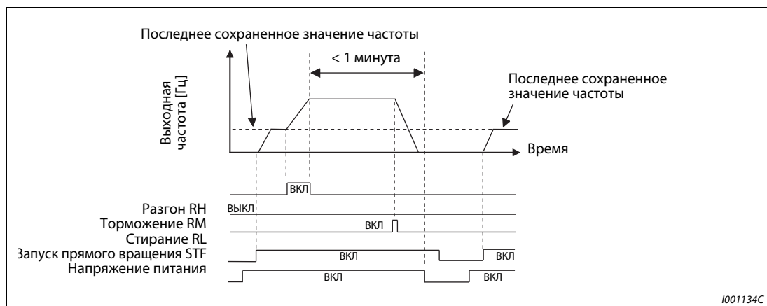
Рис. 6-28: Выдача частоты с последним сохраненным значением
