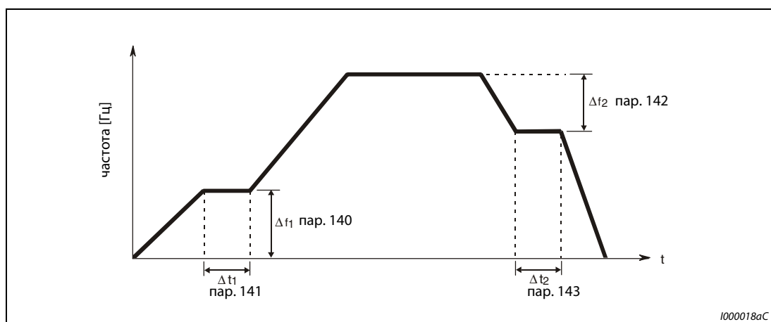
Рис. 6-36: Изменения частоты для компенсации зазора редуктора.
