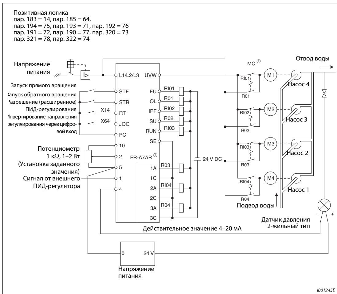
Рис. 6-178: Расширенное ПИД-регулирование ( переменный режим, режим переключения и комбинированный переменный режим/режим переключения)
