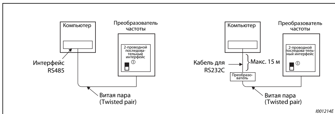
Рис. 6-139: Кабельное соединение с преобразователем частоты
