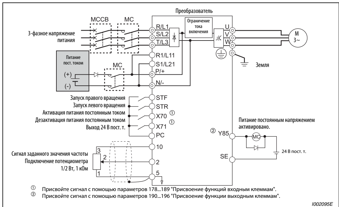
Рис. 6-47: Пример подключения для варианта 2 питания контура постоянного тока
