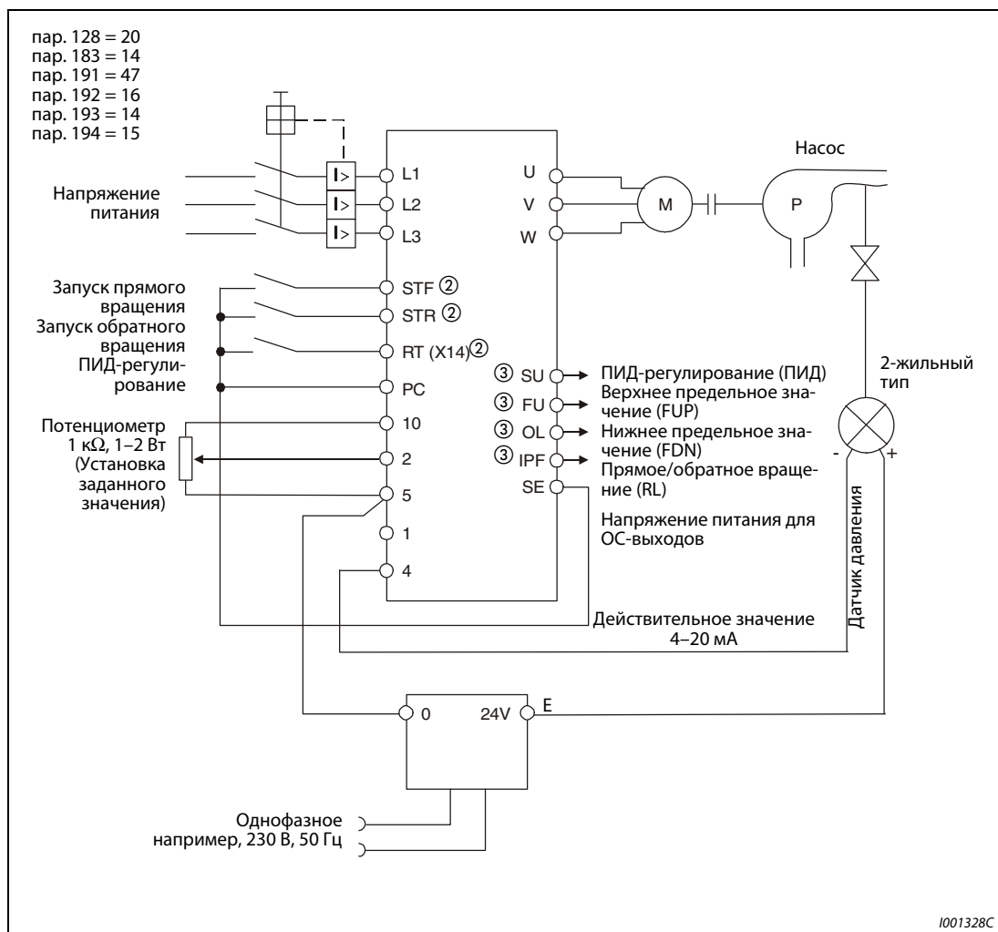
Рис. 6-164: Пример подключения при использовании позитивной логики
