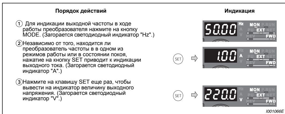
Рис. 4-6: Индикация различных рабочих параметров
