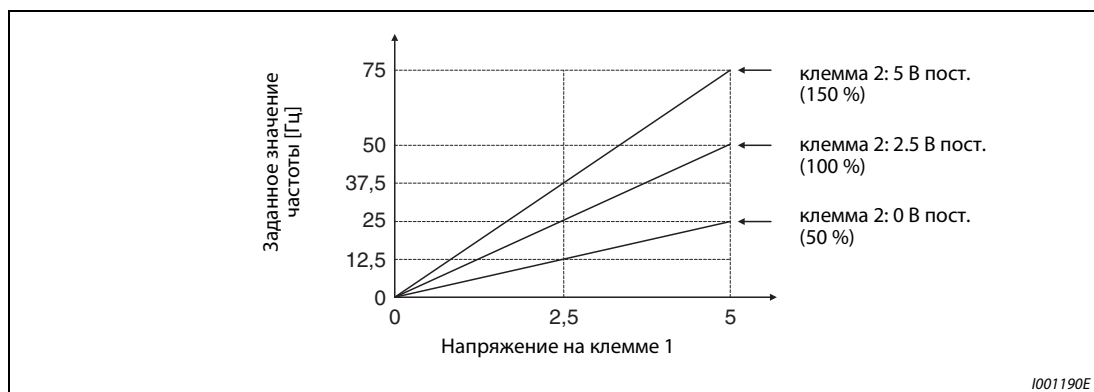
Рис. 6-113: Заданное значение частоты в зависимости от сигналов на клеммах 1 и 2.
