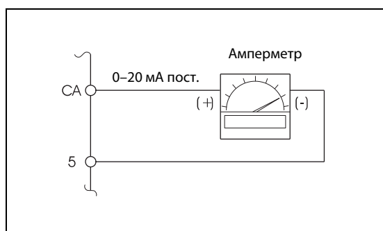
Рис. 6-78: Подключение аналогового измерительного устройства к выходу CA
