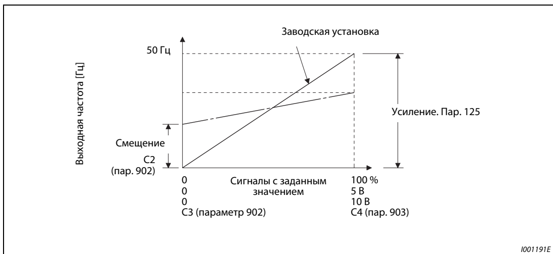
Рис. 6-114: Подгонка сигнала на клемме 2.
