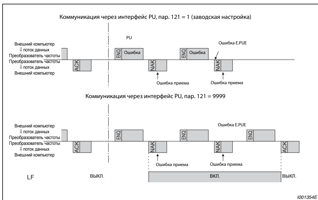
Рис. 6-148: Ошибка передачи данных
