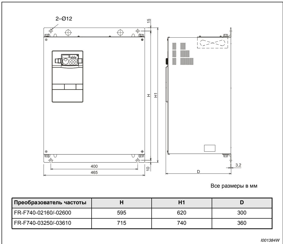
Рис. А-6: Размеры от FR-F740-02160 до -03610
