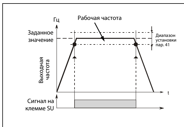
Рис. 6-64: Диаграмма выходного сигнала на клемме SU
