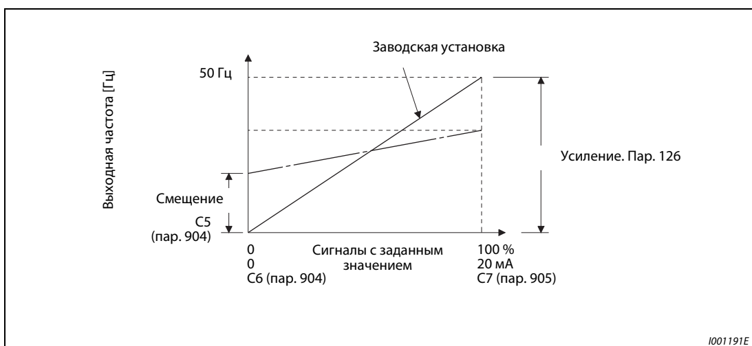
Рис. 6-115: Подгонка сигнала на клемме 4.
