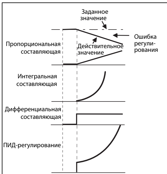
Рис. 6-161: Принцип действия ПИД-регулятора
