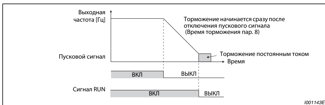
Рис. 6-50: Способ останова при пар. 250 = 9999
