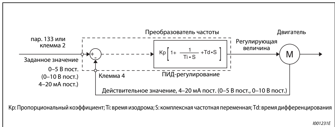
Рис. 6-158: Конфигурация системы для пар. 128 = 20 или 21, 120, 121 (клемма для установки заданного/действительного значения)
