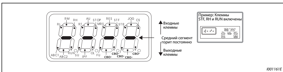
Рис. 6-73: Индикация коммутационных состояний клемм ввода/вывода
