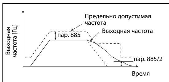
Рис. 6-190: Ограничение выходной частоты
