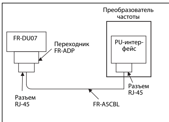
Рис. 6-133: Подключение панели управления к интерфейсу PU
