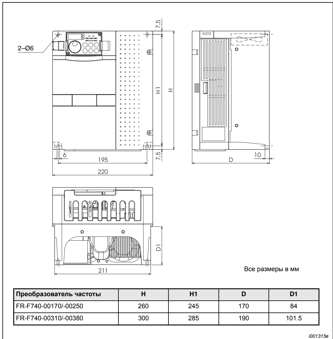
Рис. А-2: Размеры от FR-F740-00170 до -00380
