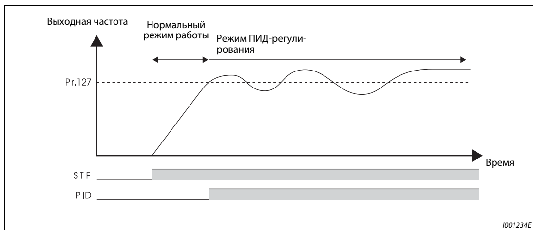
Рис. 6-165: Автоматическое переключение в режим ПИД-регулирования.
