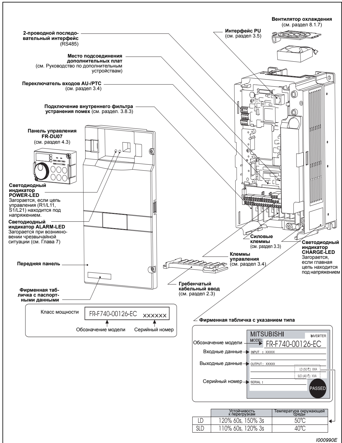
Рис. 1-3: Устройство преобразователя частоты
