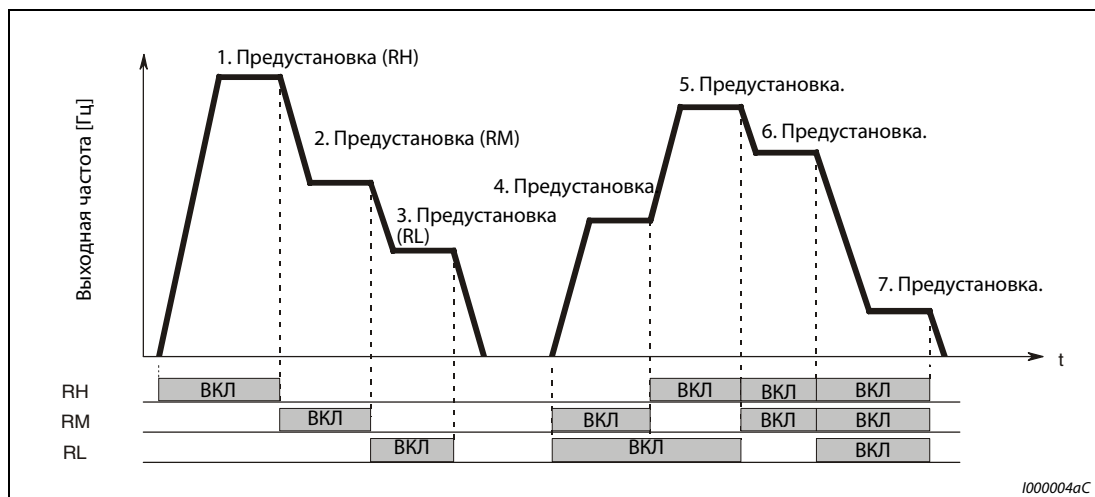
Рис. 6-17: Вызов предустановленных скоростей вращения в зависимости от наличия сигналов на клеммах.
