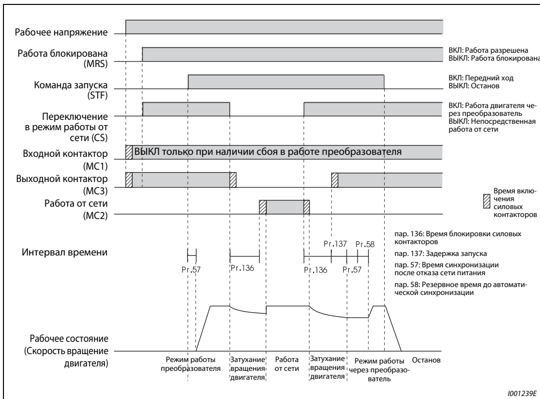
Рис. 6-172: Временная диаграмма сигналов без автоматического переключения в режим работы от сети
