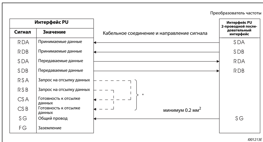
Рис. 6-136: Кабельное соединение с преобразователем частоты
