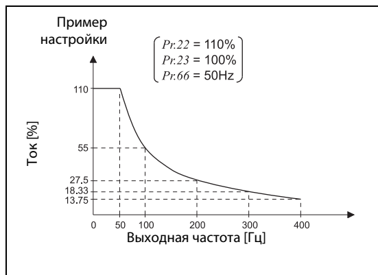
Рис. 6-5: Характеристика предельного значения тока для пар. 22 = 110 %, пар. 23 = 100 % и пар. 66 = 60 Гц
