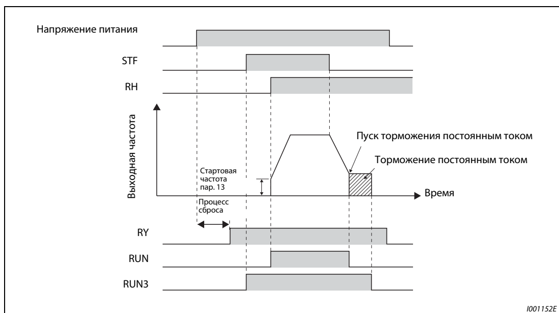
Рис. 6-62: Готовность к работе и работа двигателя
