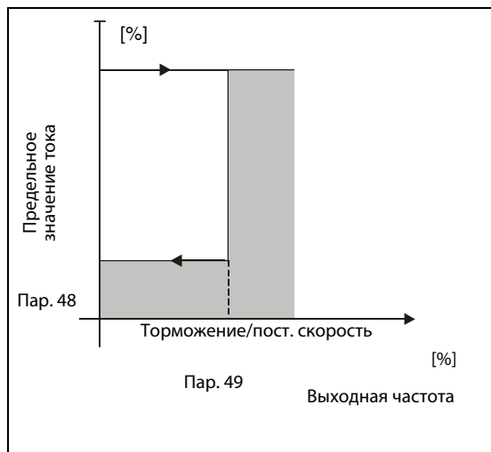
Рис. 6-6: Пример установки второго предельного значения тока
