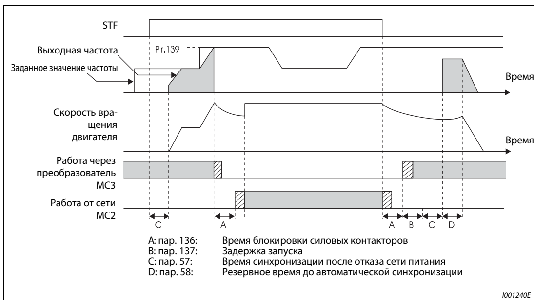
Рис. 6-173: Временная диаграмма сигналов с автоматическим переключения в режим работы от сети
