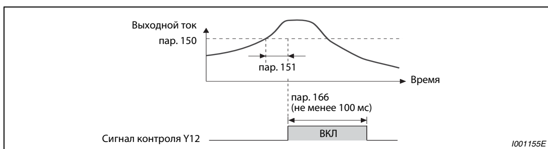
Рис. 6-66: Контроль выходного тока (Y12, пар. 166 ≠ 9999, пар. 167 = 0)
