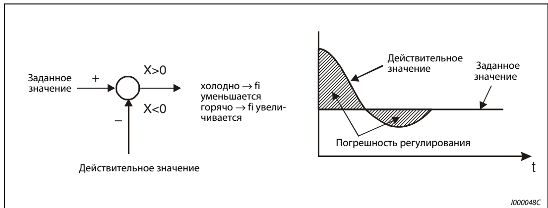
Рис. 6-163: Охлаждение
