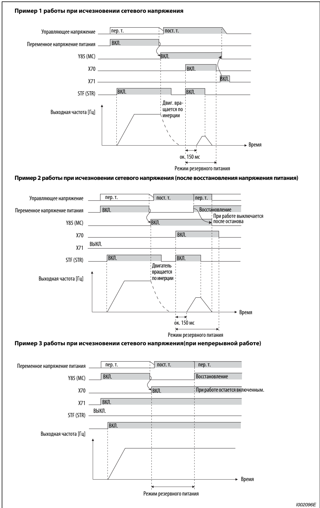
Рис. 6-48: Примеры работы при исчезновении сетевого напряжения
