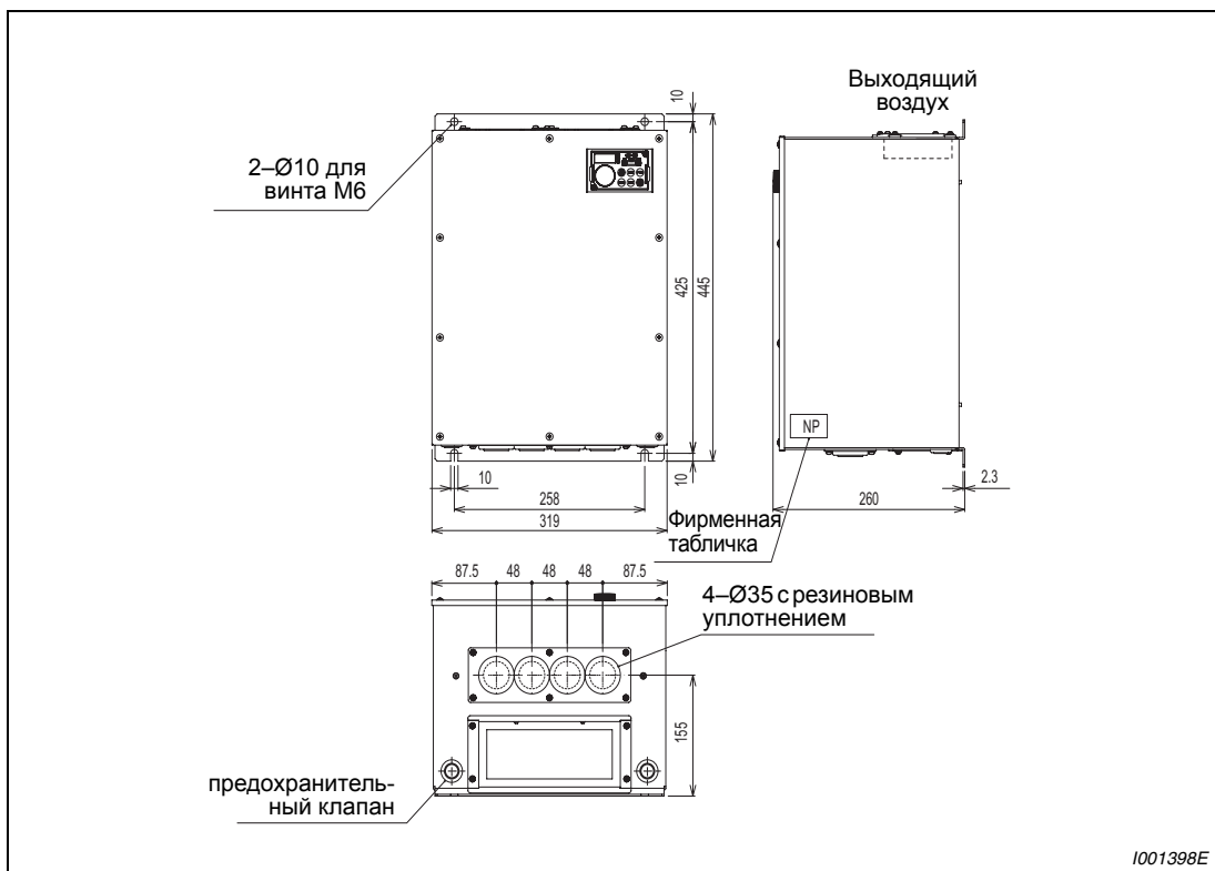
Рис. А-12: Размеры FR-F746-00310 и -00380
