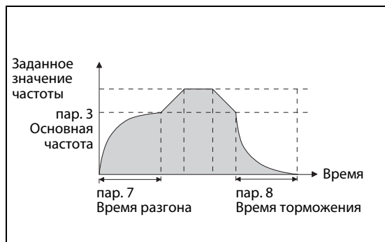
Рис. 6-37: Характеристика при пар. 29 = "6"
