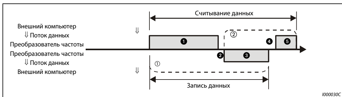
Рис. 6-144: Схематическое представление обмена данными
