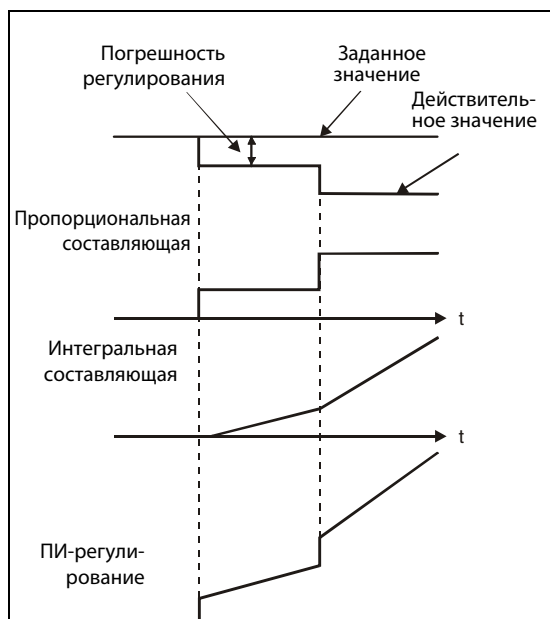
Рис. 6-159: Принцип действия ПИ-регулятора
