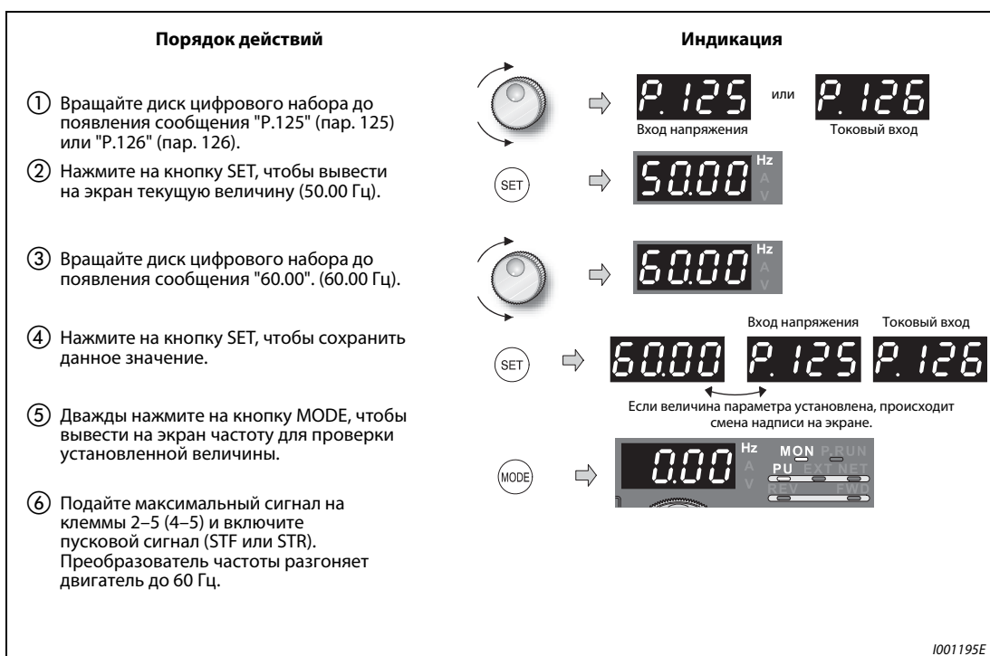
Рис. 6-118: Установка частоты без установки напряжения (тока)
