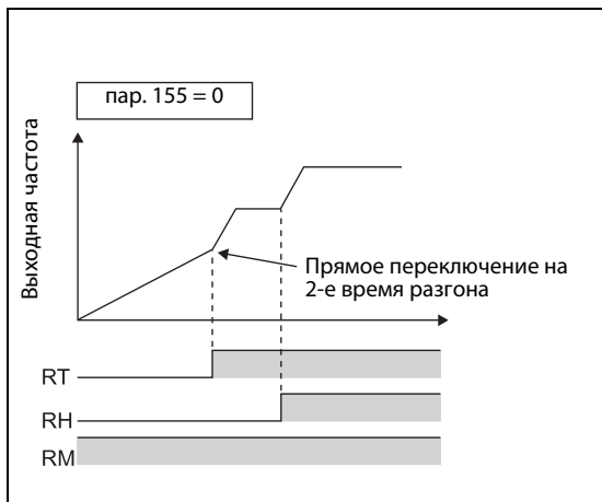
Рис. 6-57: Пример переключения времени разгона/ торможения
