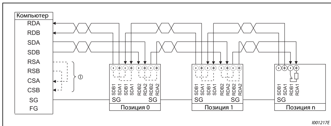
Рис. 6-142: Кабельное соединение с несколькими преобразователями частоты
