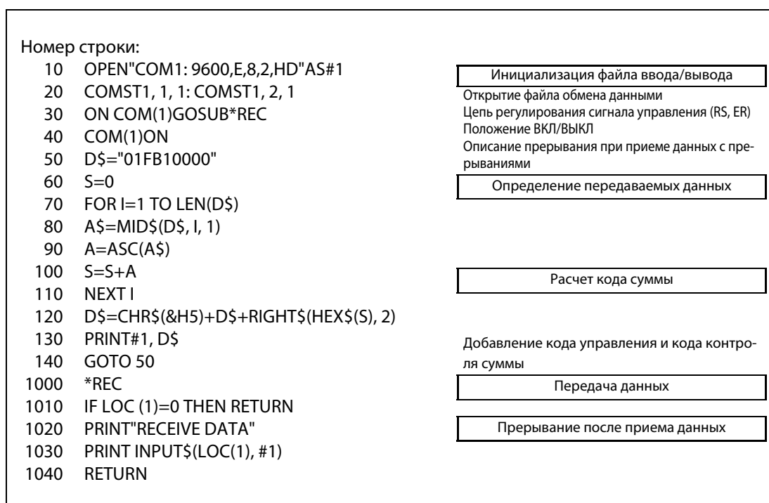
Рис. 6-150: Пример программы
