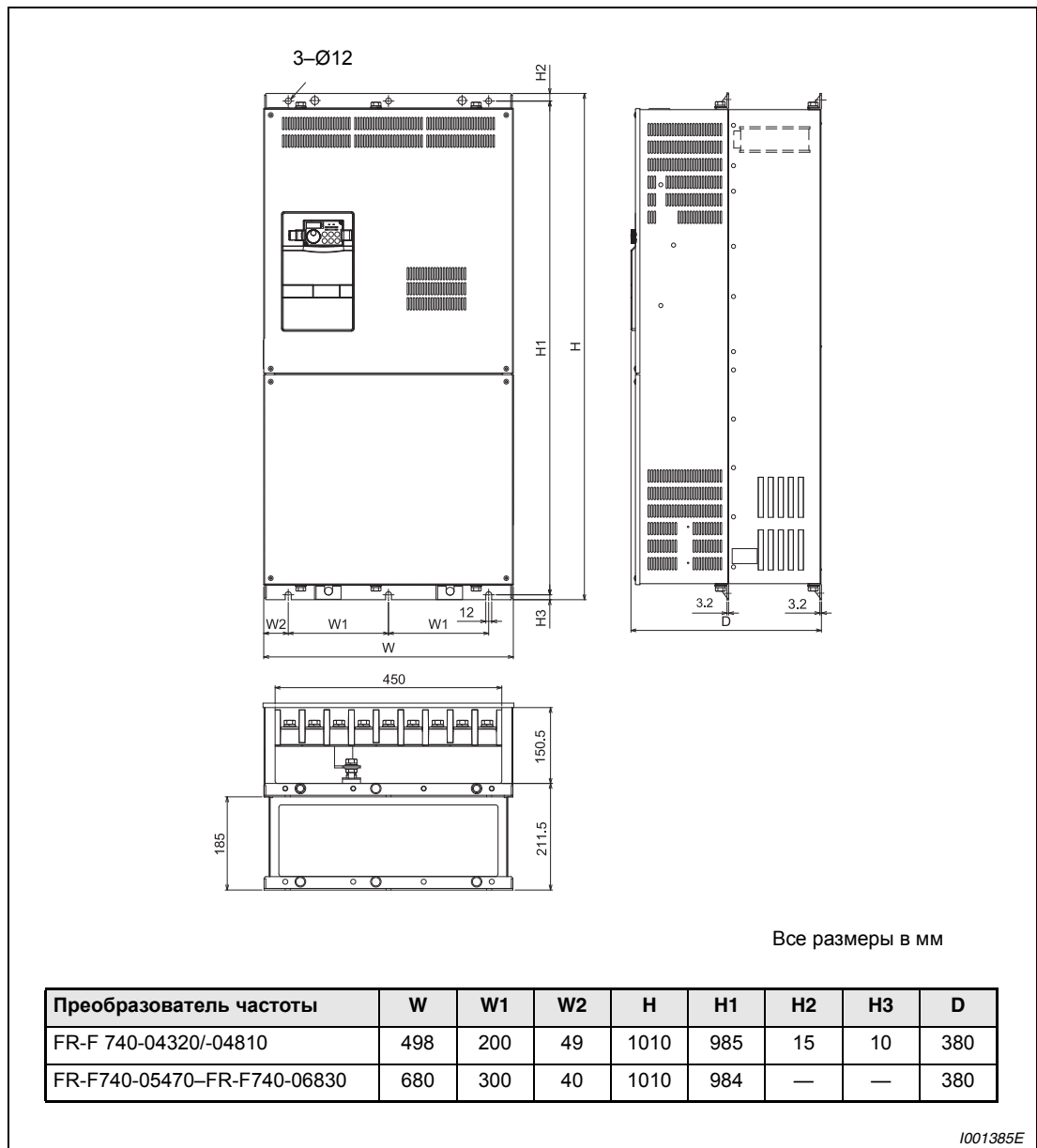
Рис. А-7: Размеры от FR-F740-04320 до -06830
