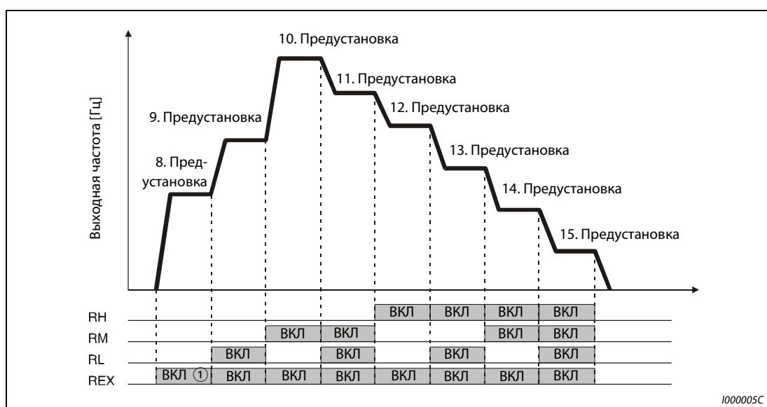
Рис. 6-18: Вызов предустановленных скоростей вращения в зависимости от наличия сигналов на клеммах.
