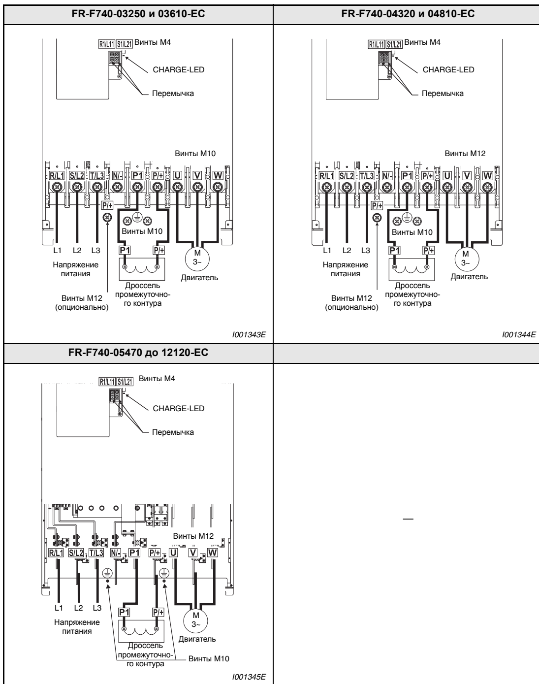
Таб. 3-3: Расположение клемм и проводные соединения (3)
