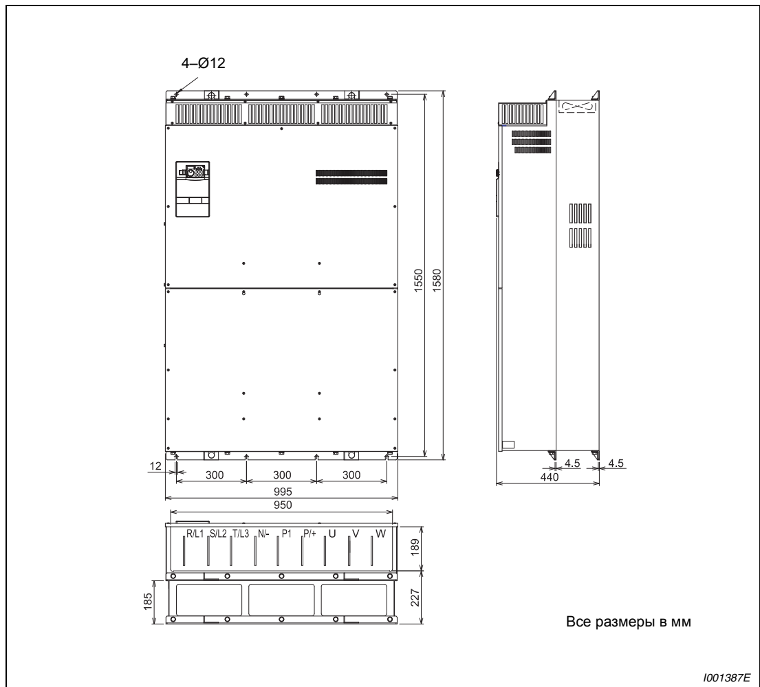
Рис. А-9: Размеры от FR-F740-09620 до -12120
