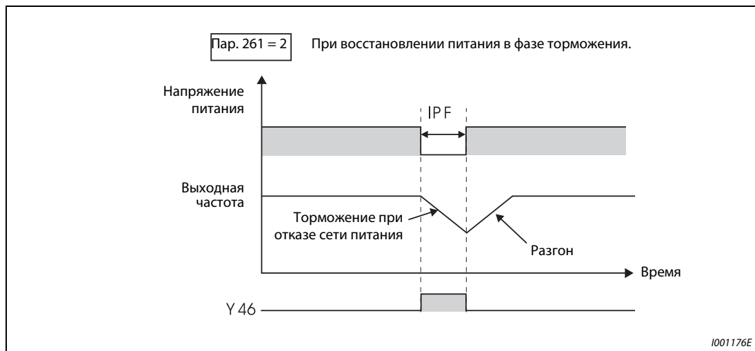
Рис. 6-91: Продолжение работы после отключения сети.
