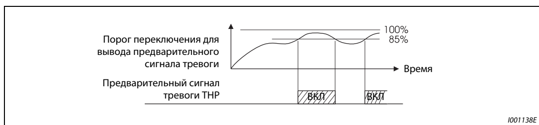
Рис. 6-40: Вывод предварительного сигнала тревоги
