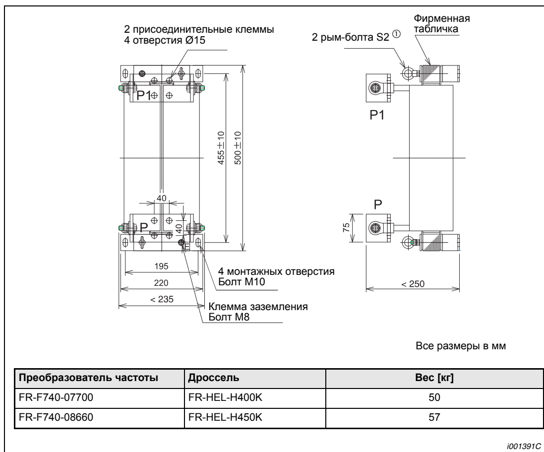
Рис. А-19: Дроссель промежуточного контура FR-HEL-H400K–450K
