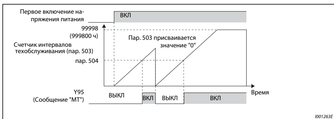
Рис. 6-193: Счетчик интервалов техобслуживания
