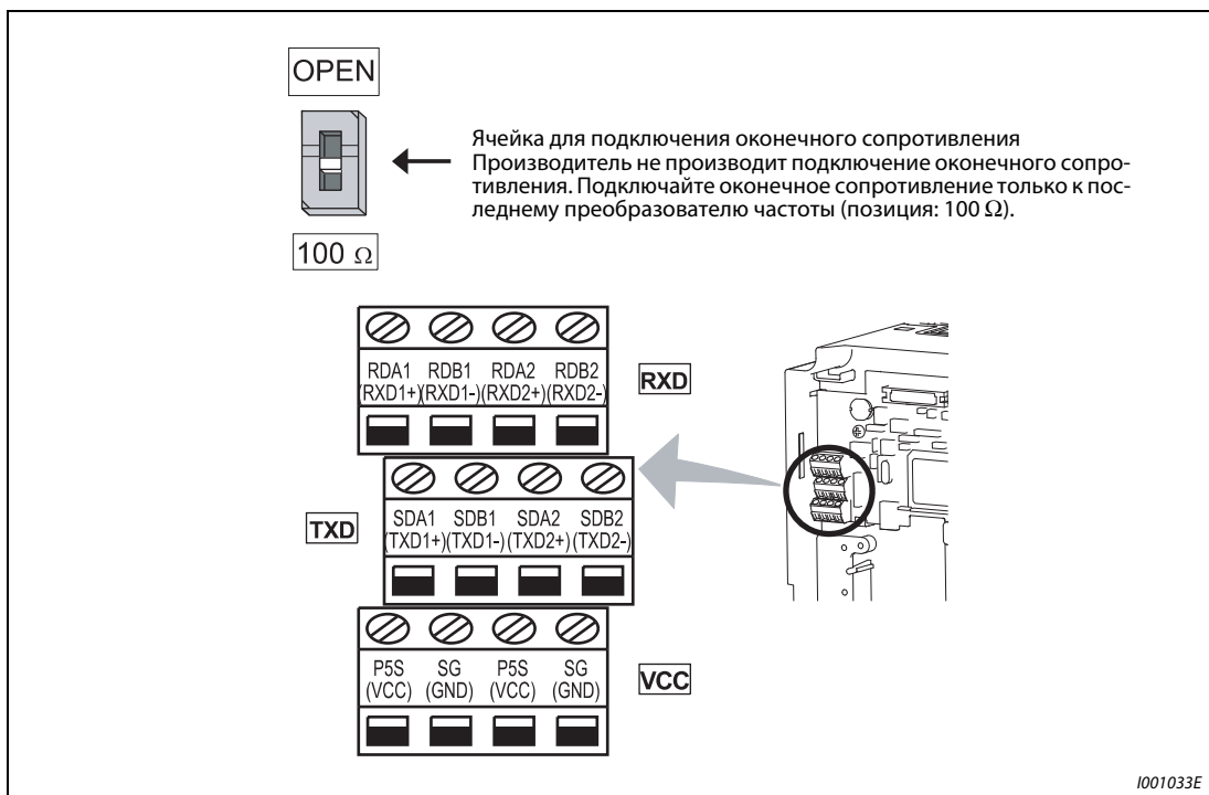
Рис. 6-137: 2.-проводной последовательный интерфейс преобразователя частоты
