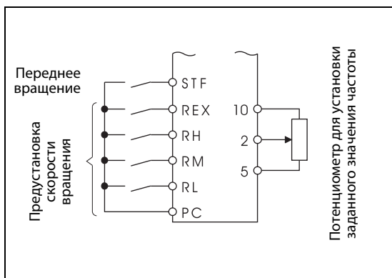
Рис. 6-19: Пример подключения
