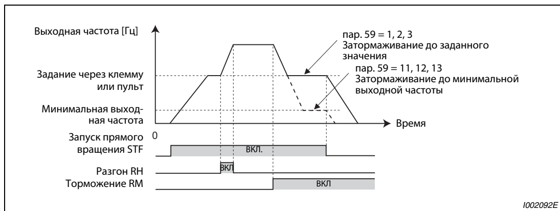
Рис. 6-27: Пример работы цифрового потенциометра двигателя (2)
