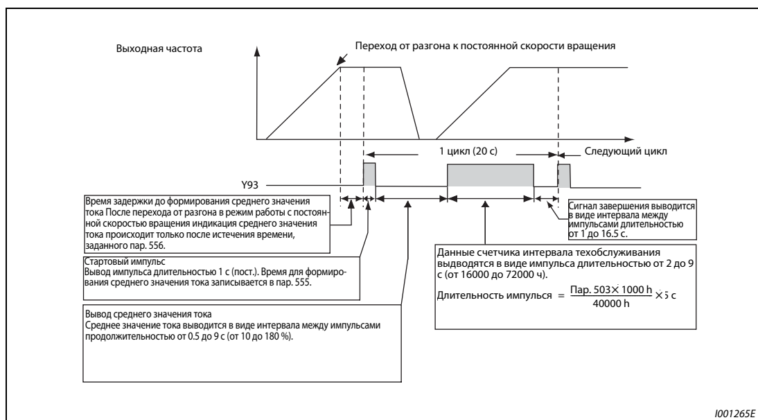
Рис. 6-195: Вывод импульсного сигнала Y93
