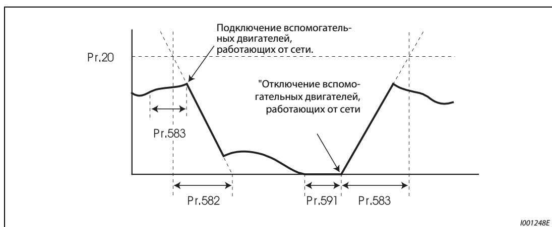
Рис. 6-181: Время торможения/разгона
