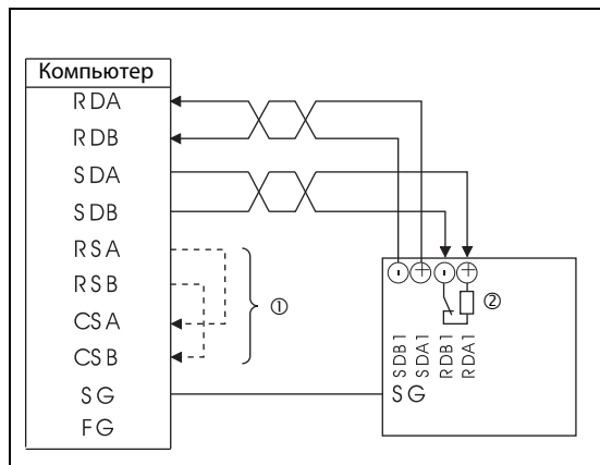
Рис. 6-141: Кабельное соединение с преобразователем частоты
