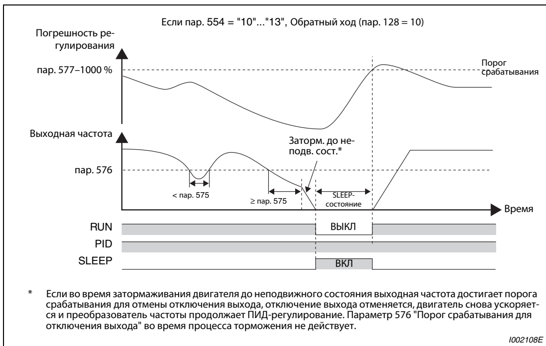
Рис. 6-167: Отключение выхода (функция SLEEP), если пар. 554 = "10" ... "13"
