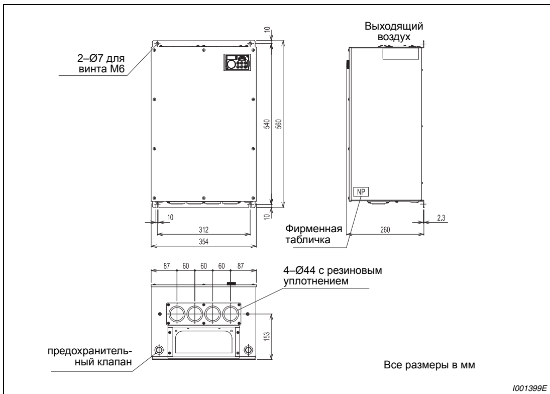
Рис. А-13: Размеры FR-F746-00470 и -00620
