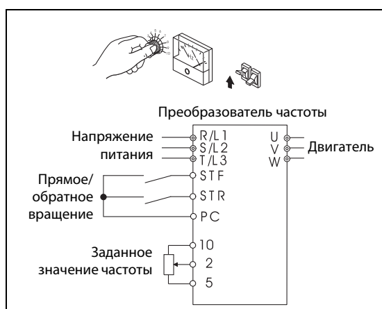
Рис. 6-128: Внешнее управление
