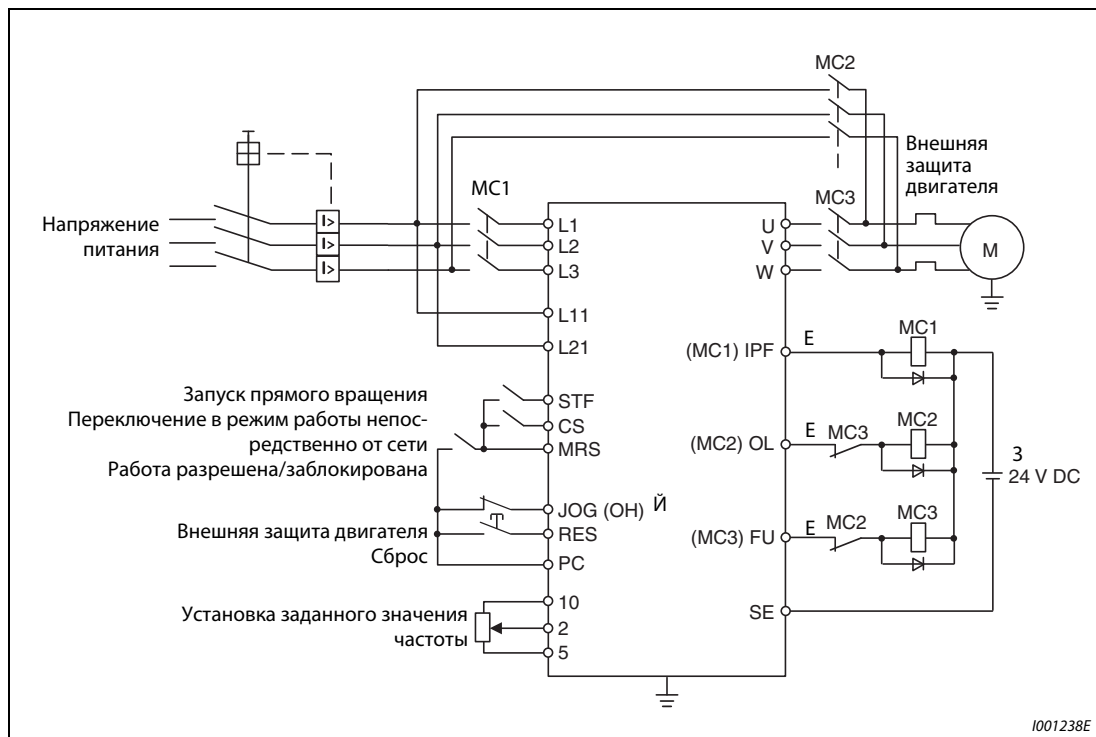
Рис. 6-171: Подключение силовых контакторов
