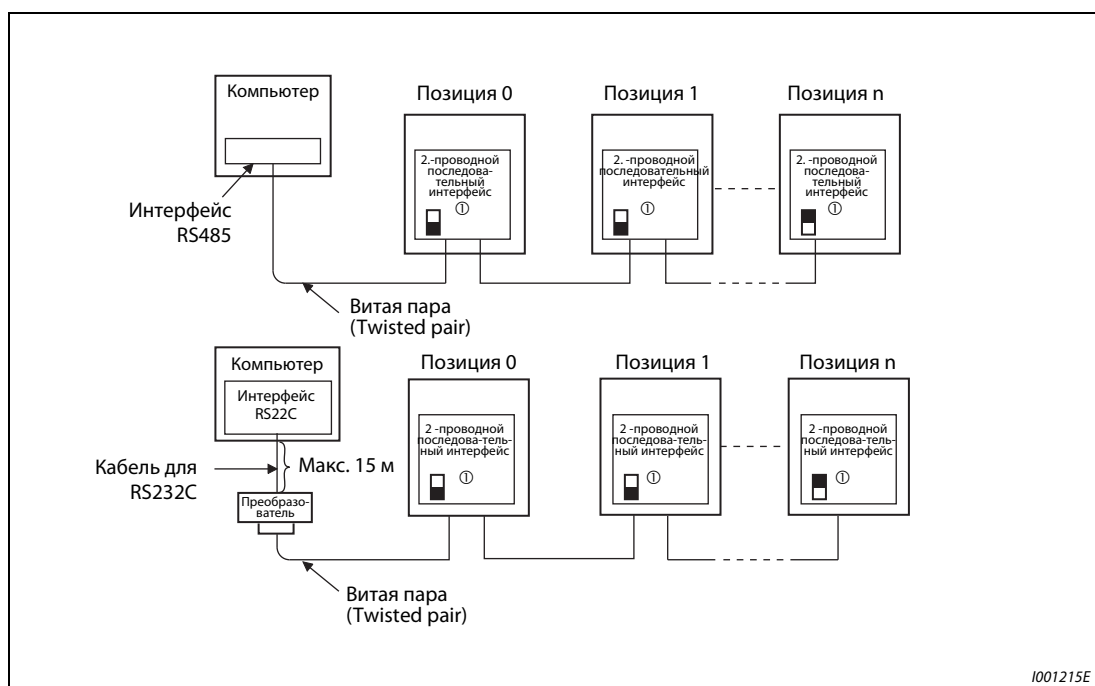
Рис. 6-140: Кабельное соединение с несколькими преобразователями частоты
