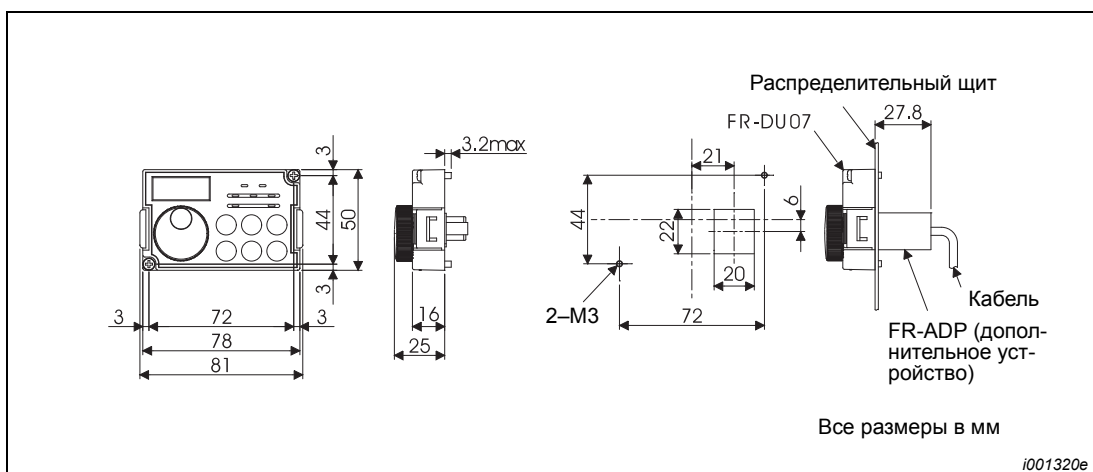
Рис. А-21: Панель управления FR-DU07
