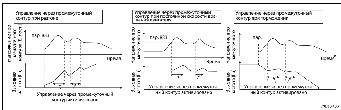
Рис. 6-189: Управление через промежуточный контур
