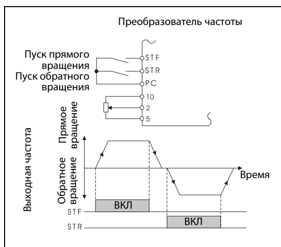
Рис. 6-58: Управление по 2-жильному проводу цепи управления (пар. 250 = 9999)
