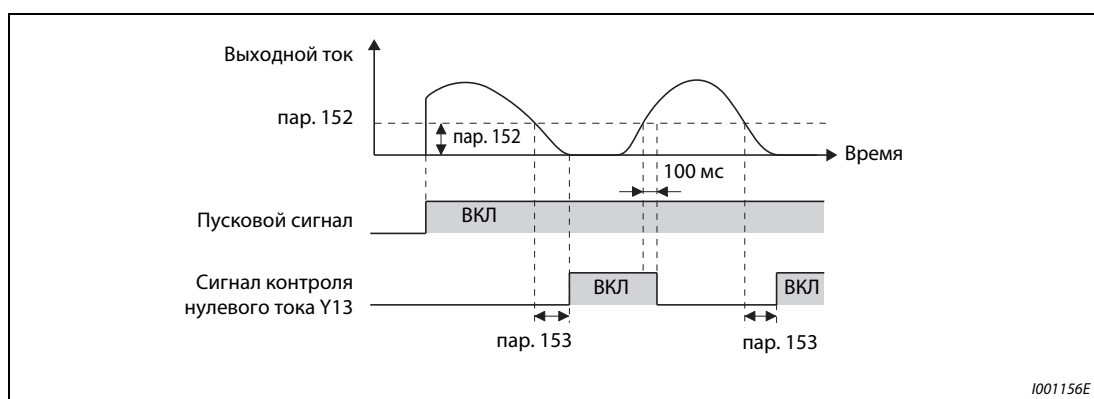
Рис. 6-67: Контроль нулевого тока
