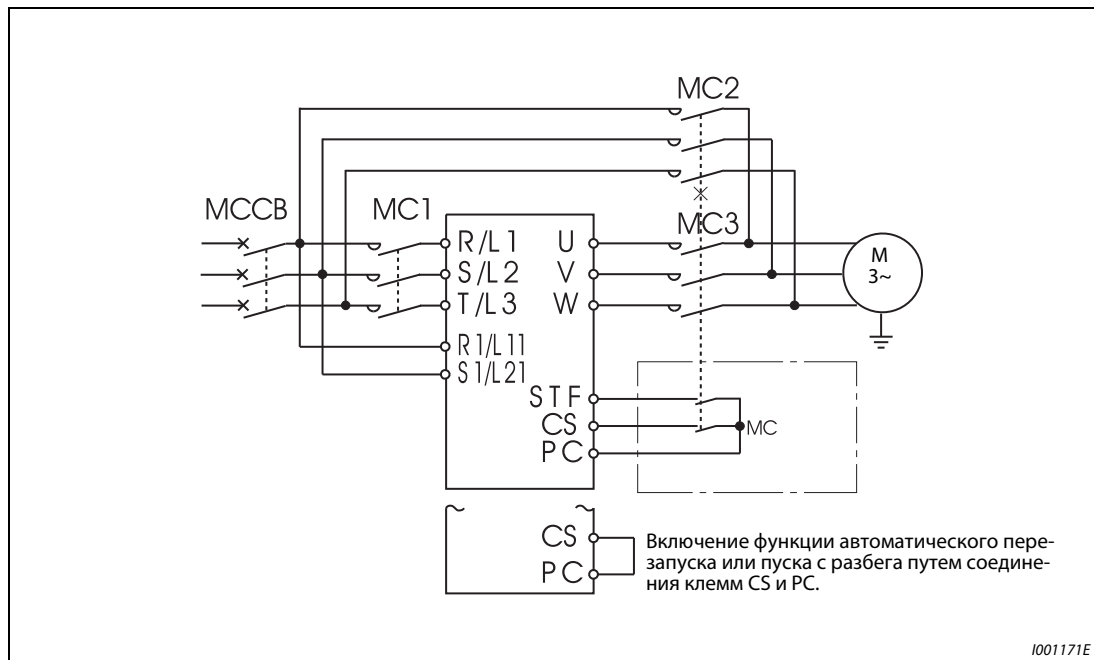
Рис. 6-86: Пример подключения
