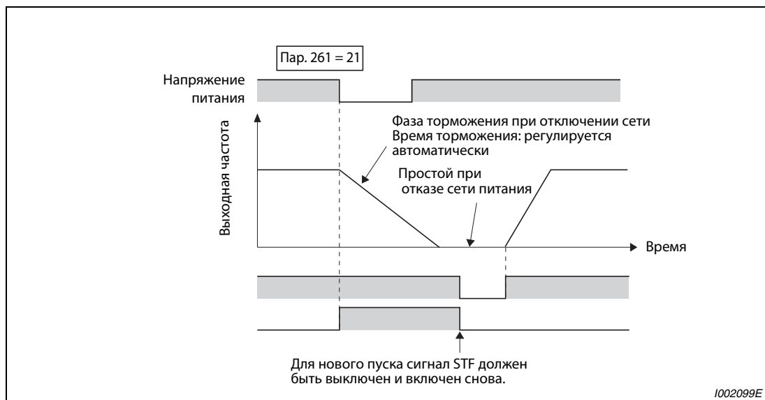
Рис. 6-93: Режим останова при исчезновении сетевого напряжения
