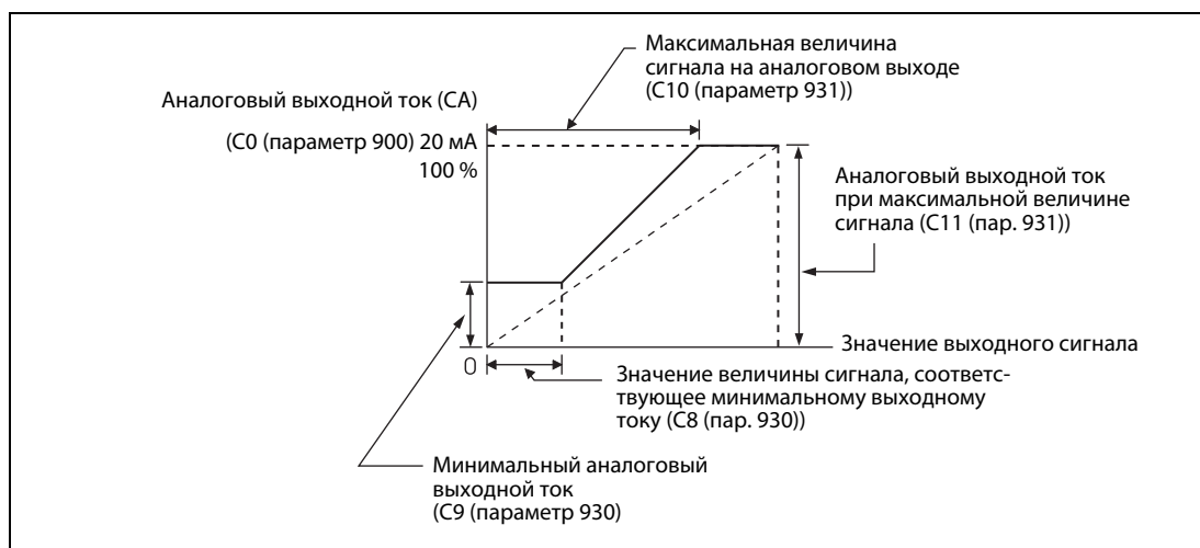
Рис. 6-79: Калибровка выхода СА
