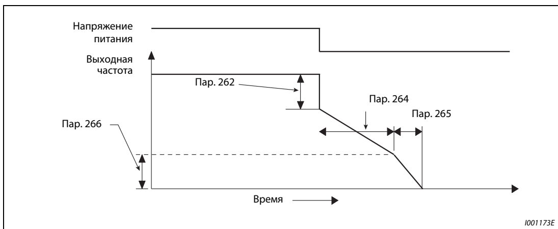
Рис. 6-88: Параметры для выбора способа останова при отказе сети питания
