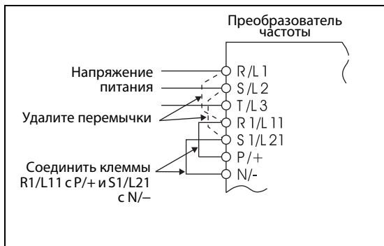
Рис. 6-87: Подключение
