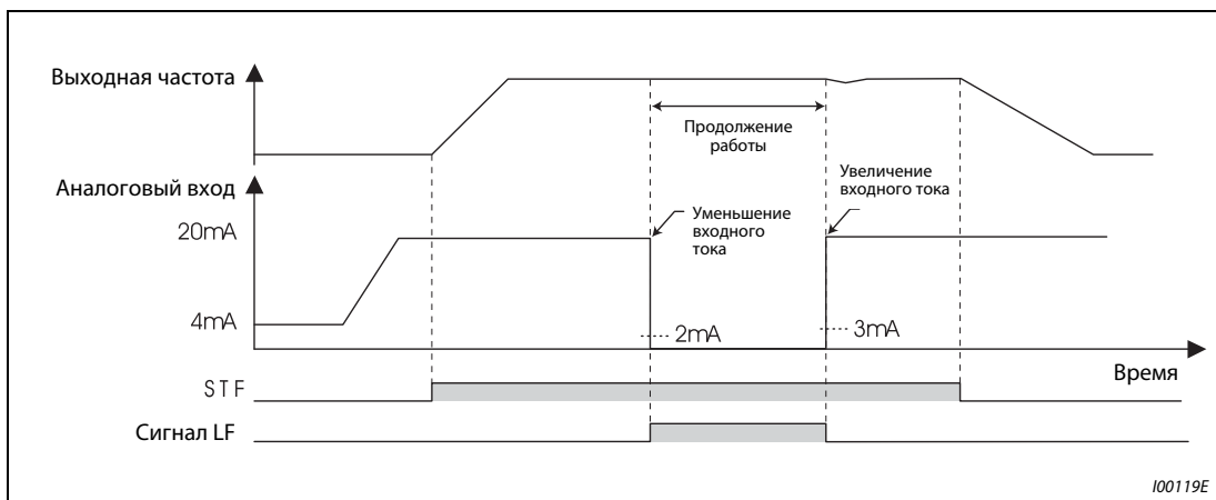
Рис. 6-120: Снижение заданной величины тока при работе в режиме внешнего управления (пар. 573 = 1)
