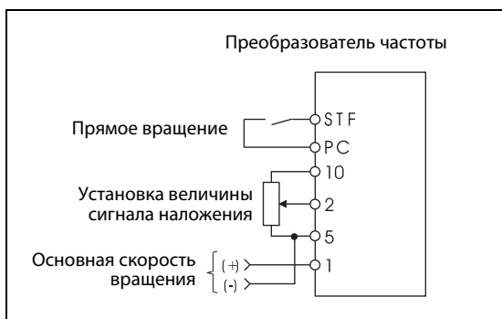
Рис. 6-111: Пример схемы для осуществления процентного наложения
