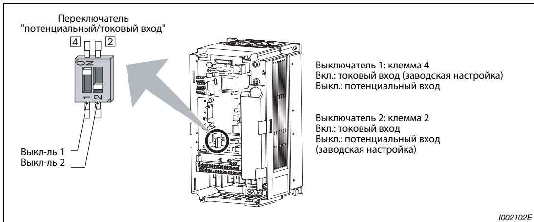
Рис. 6-102: Переключатель "Потенциальный/токовый вход"
