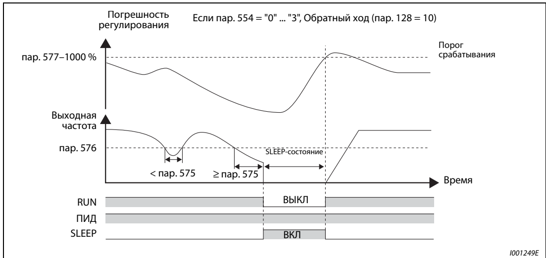
Рис. 6-182: Отключение выхода при обратном ходе (пар. 554 = "10" ... "13", пар. 128 = "10 "
