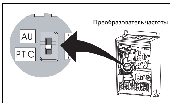
Рис. 6-43: Переключатель AU/PTC
