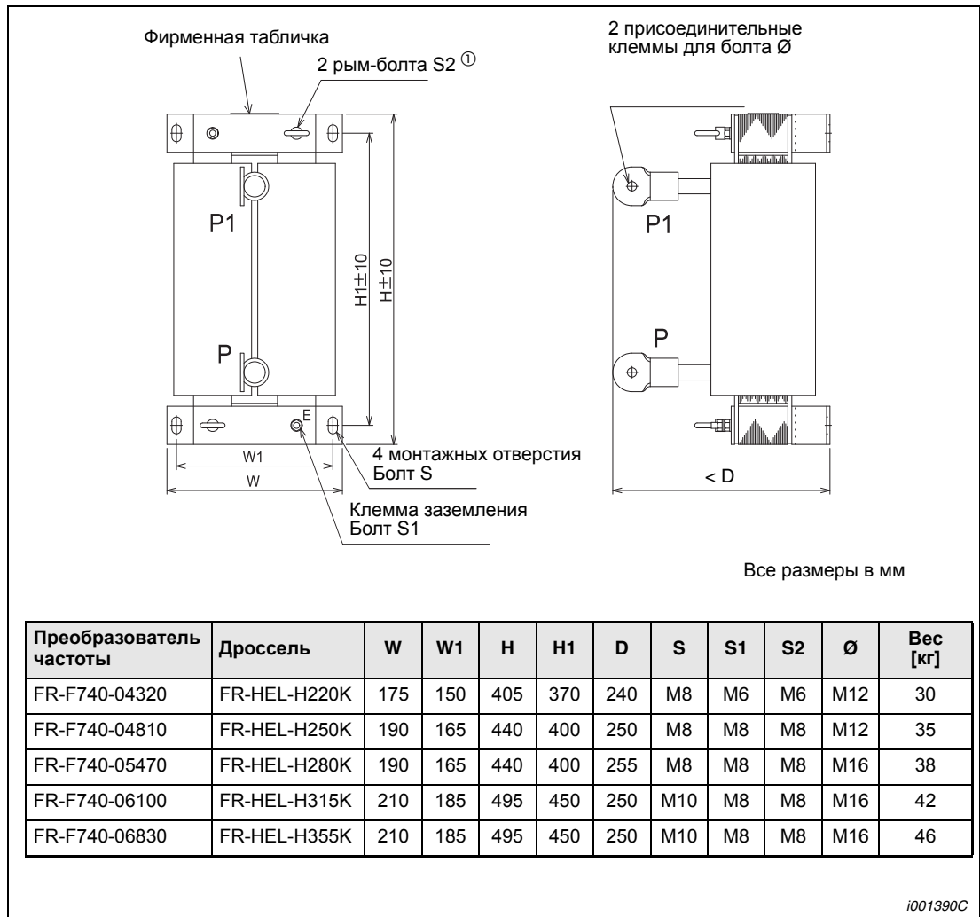
Рис. А-18: Дроссель промежуточного контура FR-HEL-H220K-355K
