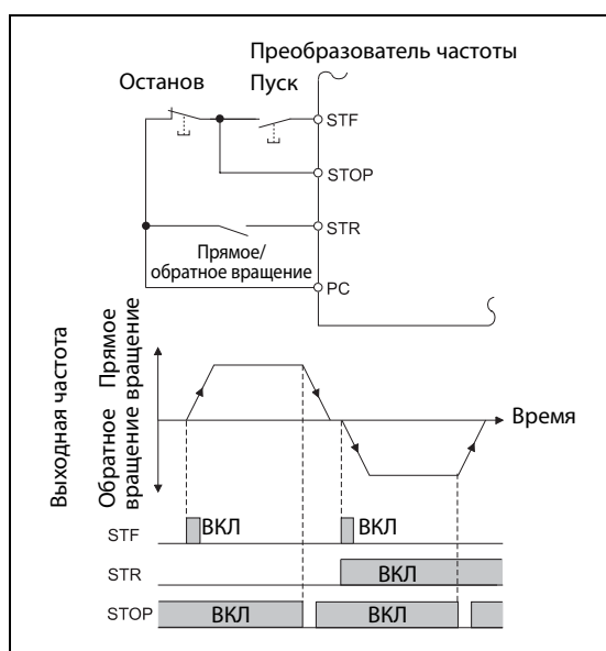
Рис. 6-61: Управление по 3-жильному проводу цепи управления (пар. 250 = 8888)
