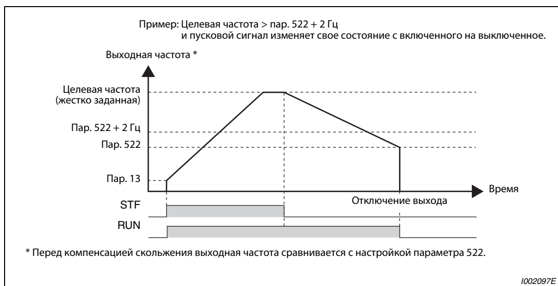
Рис. 6-52: Пример 1: Целевая частота > пар. 522 + 2 Гц, пусковой сигнал = ВКЛ./ВЫКЛ.
