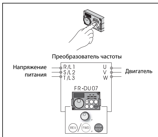
Рис. 6-129: Управление через панель управления
