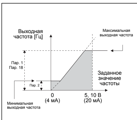
Рис. 5-3: Минимальная и максимальная выходная частота
