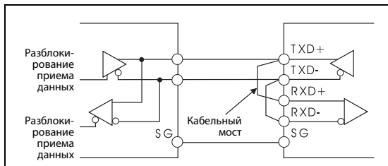
Рис. 6-143: Соединение через двухпроводную линию
