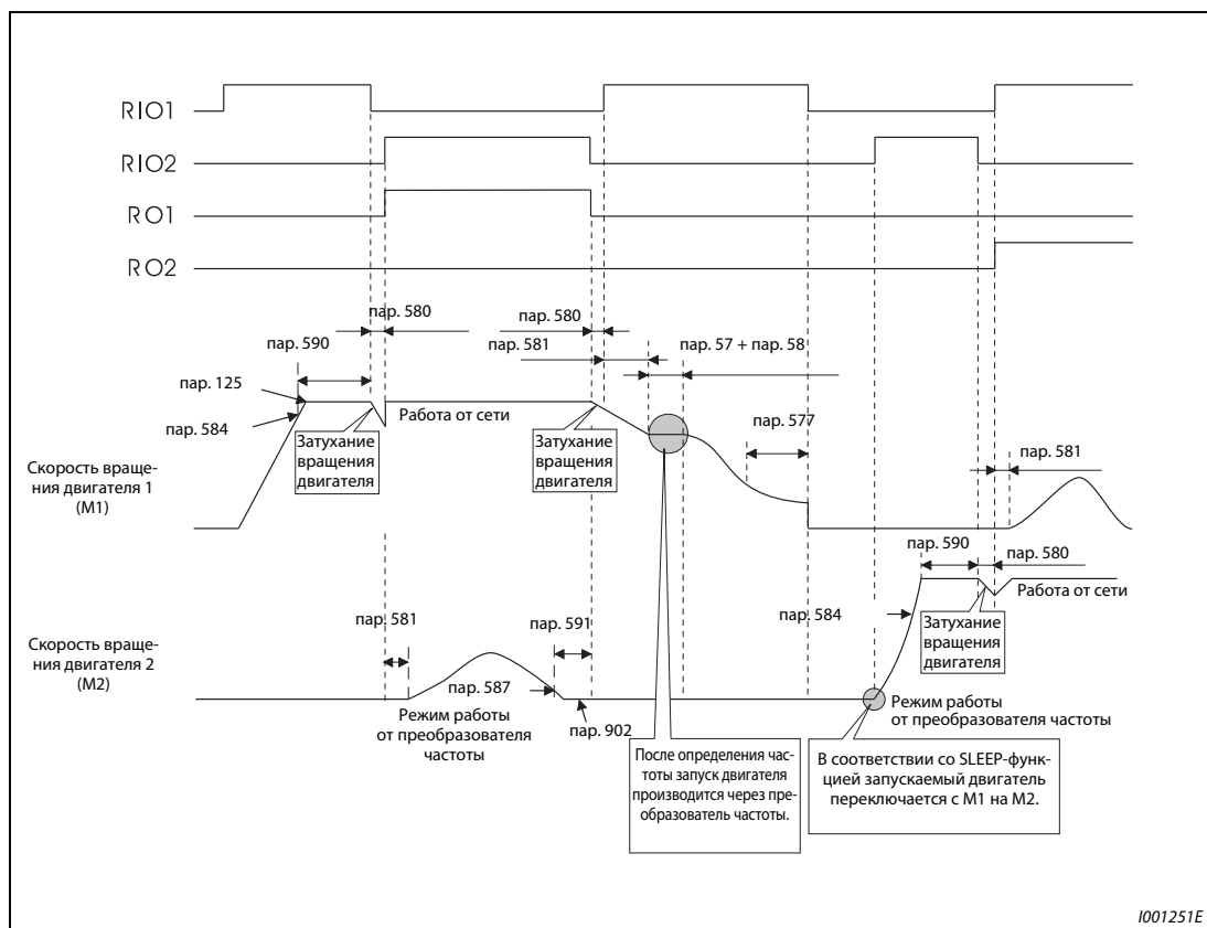
Рис. 6-187: Переходная характеристика в переменном режиме/режиме переключения
