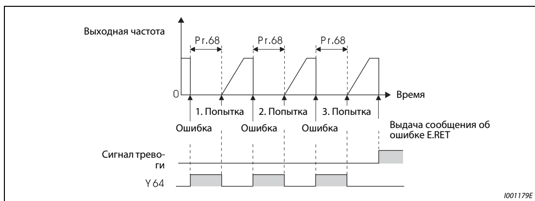
Рис. 6-97: Пример неудачных попыток перезапуска
