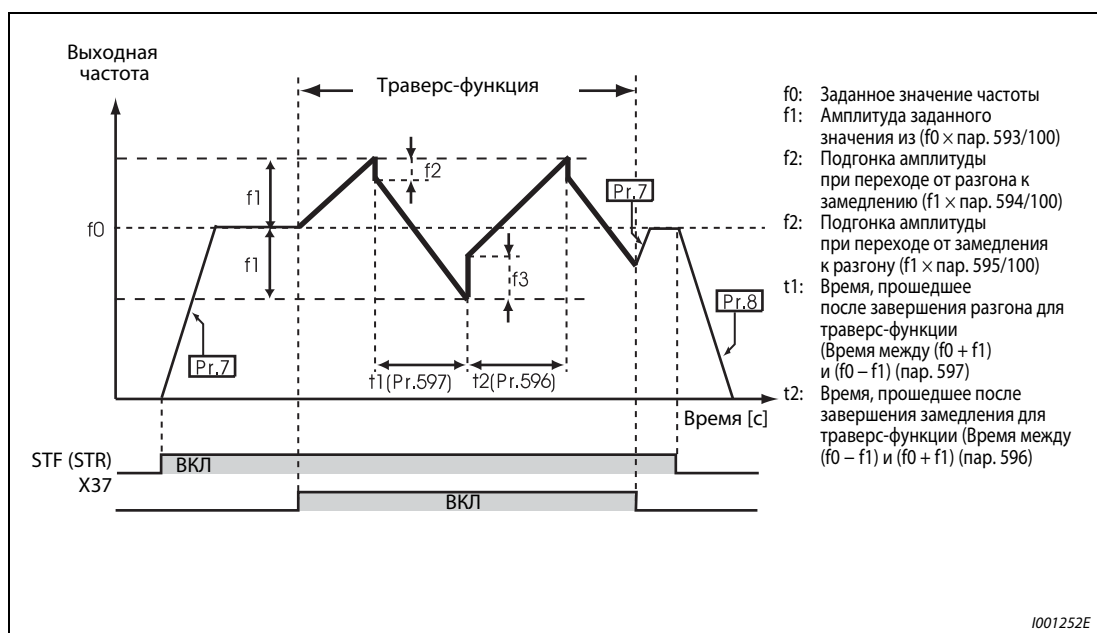
Рис. 6-188: Траверс-функция
