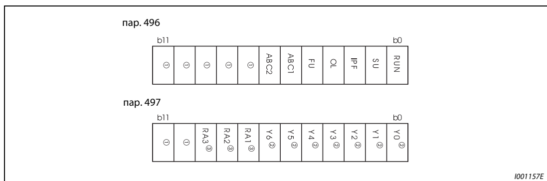
Рис. 6-68: Децентрализованные выходные данные
