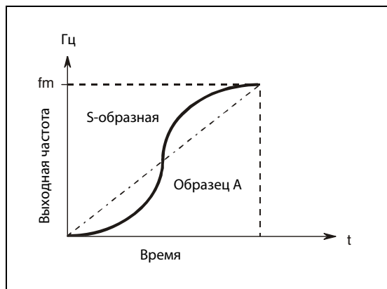
Рис. 6-34: Характеристика при пар. 29 = "1"
