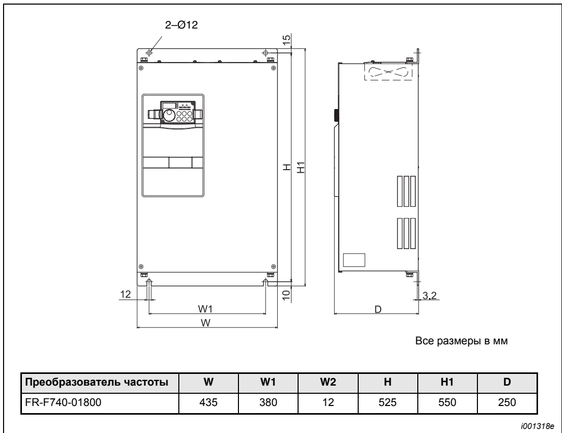
Рис. А-5: Размеры FR-F740-01800
