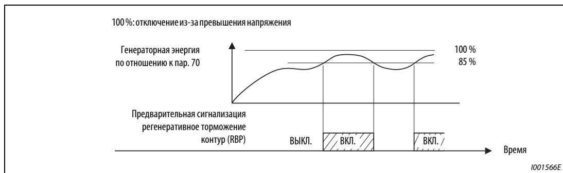
Рис. 6-49: Генераторная перегрузка
