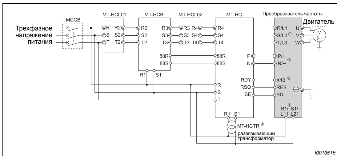
Рис. 3-31: Подключение комбинированного устройства рекуперации энергии/ сетевого фильтра MT-НС.
