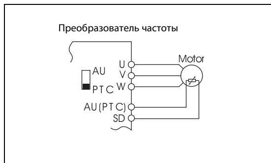
Рис. 6-42: Подключение температурного датчика РТС
