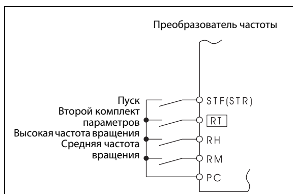
Рис. 6-56: Пример подключения для выбора второго комплекта параметров
