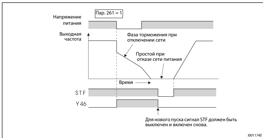
Рис. 6-89: Восстановление питания
