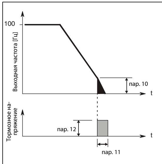
Рис. 6-44: Присвоение пар. 11 значения между 0.1 и 10 с.
