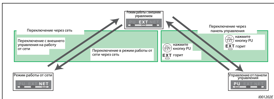
Рис. 6-126: Переключение режима работы при пар. 340 = 0, 1 или 2
