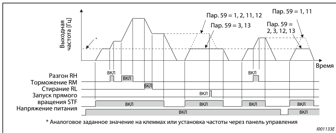
Рис. 6-26: Пример работы цифрового потенциометра двигателя (1)
