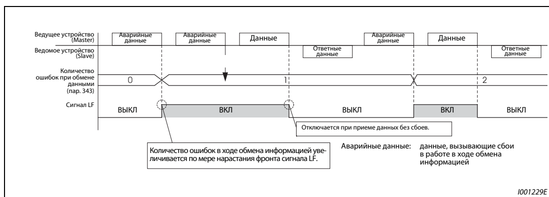
Рис. 6-155: Вывод сигнала LF
