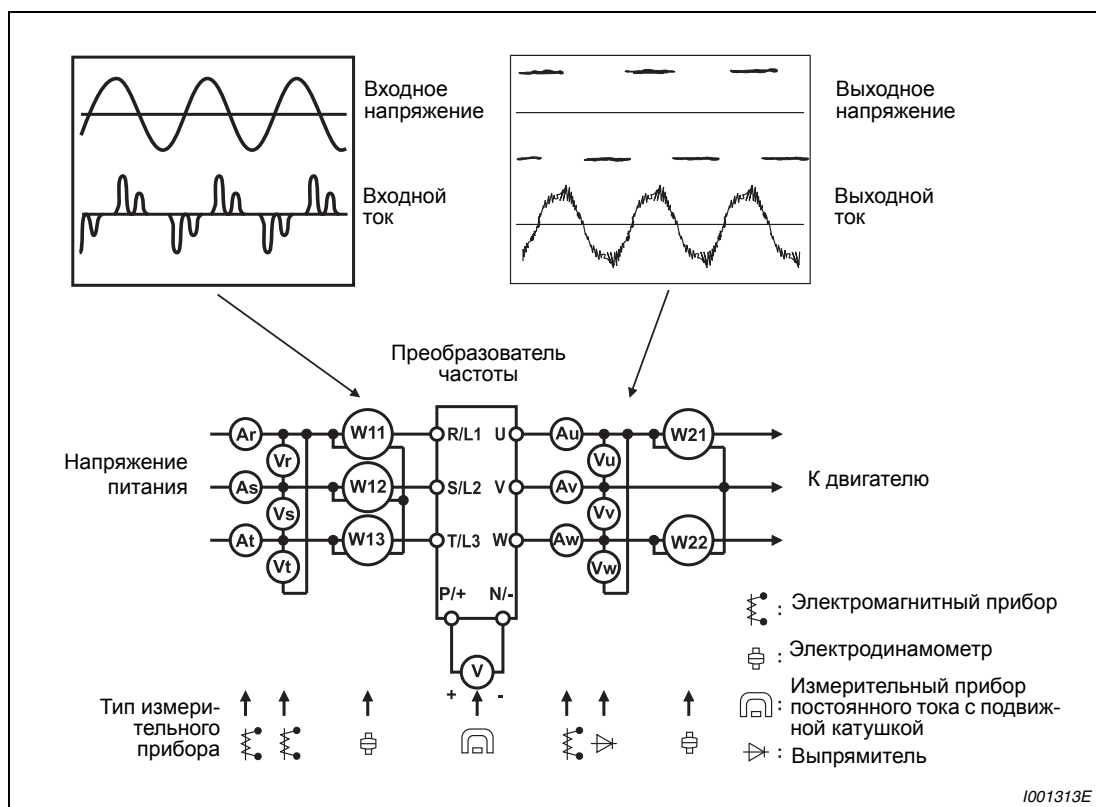
Рис. 7-7: Измерения на блоке питания
