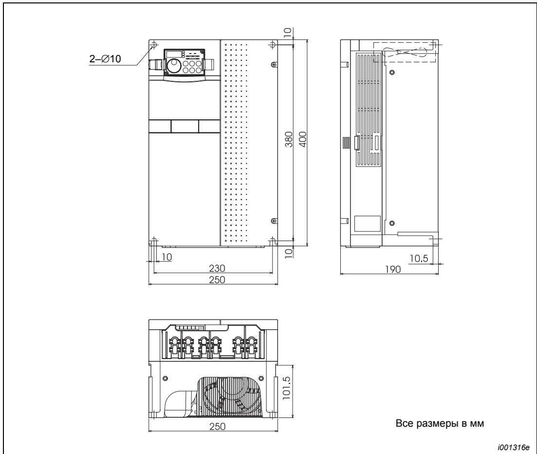
Рис. А-3: Размеры от FR-F740-00470 и -00620
