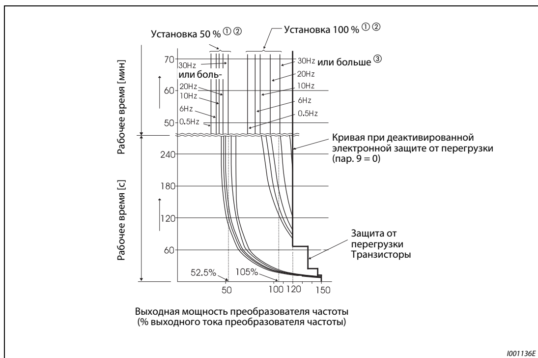
Рис. 6-38: Характеристики защиты двигателя
