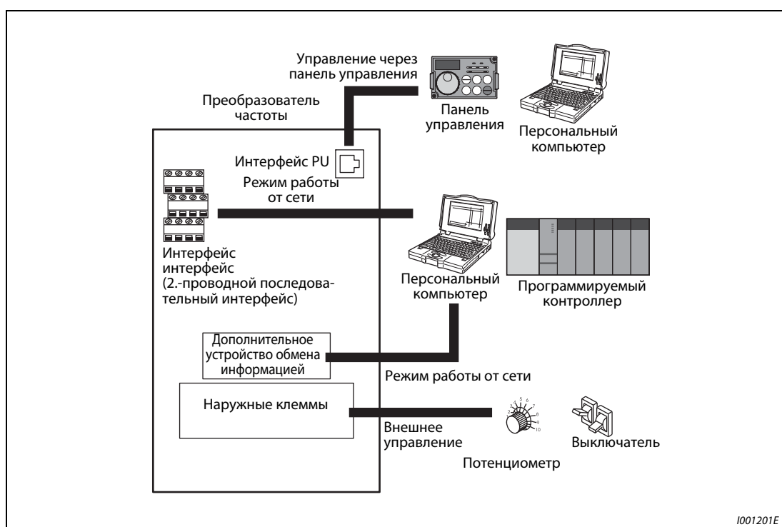
Рис. 6-125: Режимы работы преобразователя частоты
