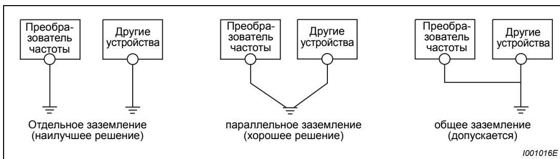
Рис. 3-6: Заземление приводной системы
