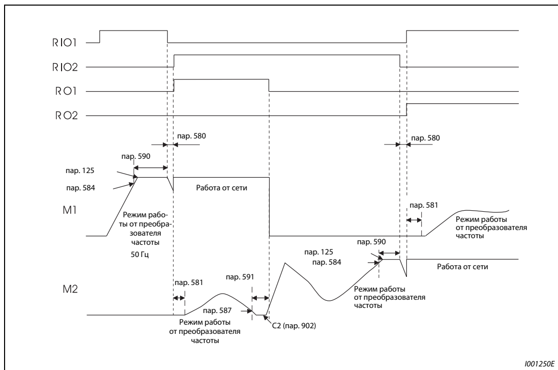
Рис. 6-186: Переходная характеристика в режиме переключения
