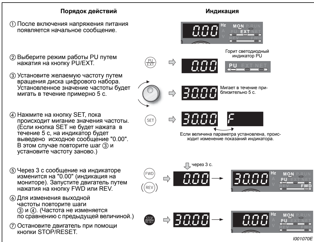
Рис. 4-10: Установка частоты при помощи диска цифрового набора
