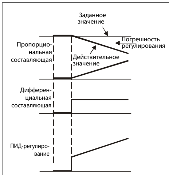
Рис. 6-160: Принцип действия ПД-регулятора
