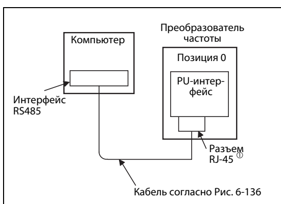
Рис. 6-134: Подключение компьютера с интерфейсом RS485 к интерфейсу PU
