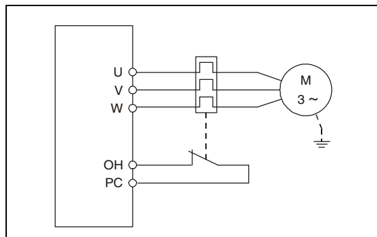
Рис. 6-41: Подключение внешней защиты двигателя
