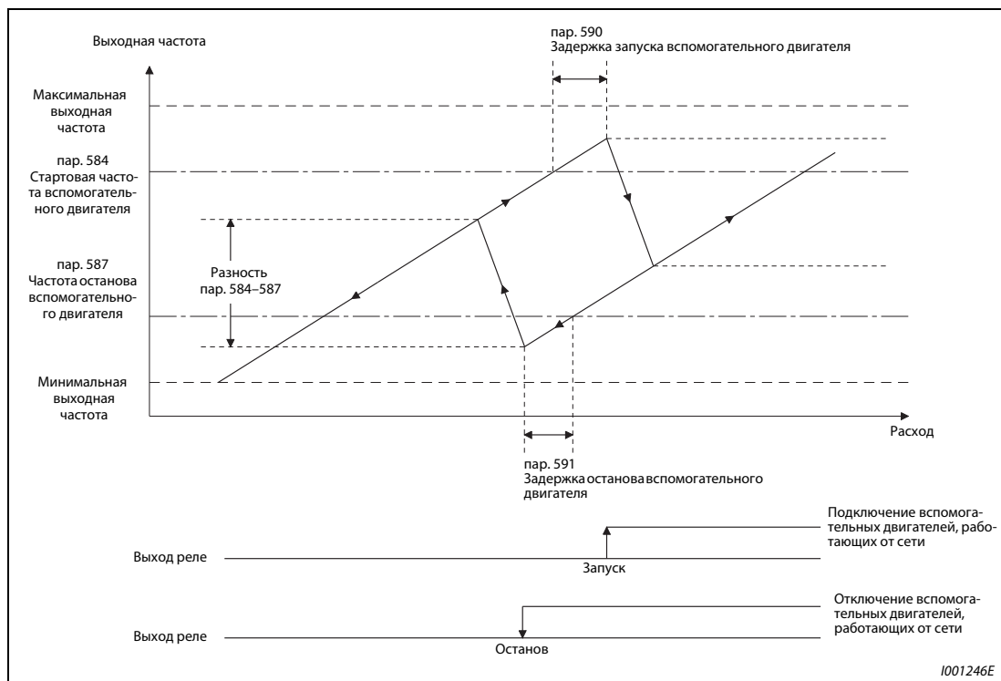
Рис. 6-179: Схема последовательности действий при запуске и останове вспомогательного двигателя 1
