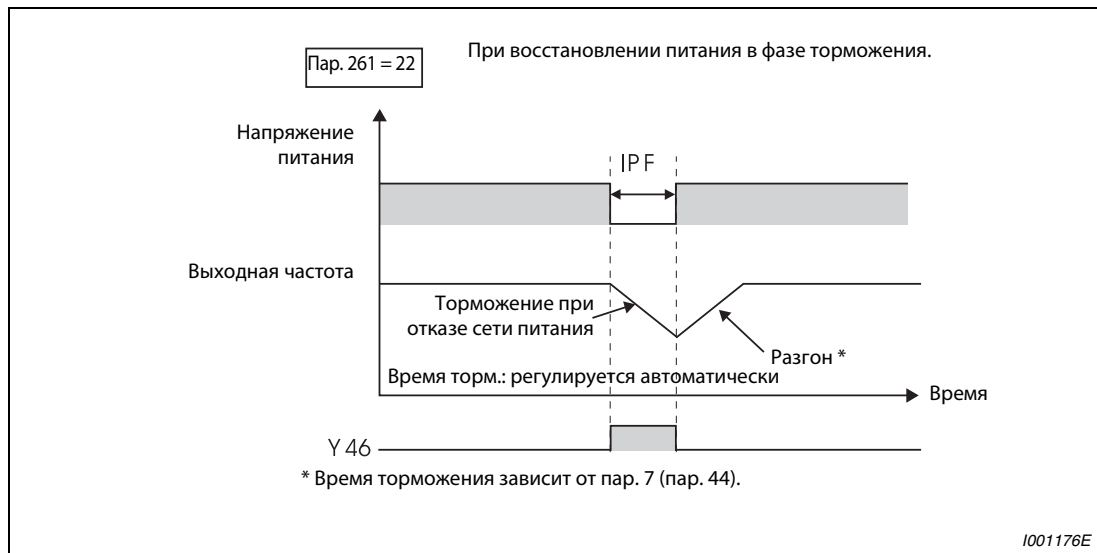
Рис. 6-94: Продолжение работы после отказа сети питания (пар. 261 = 22)
