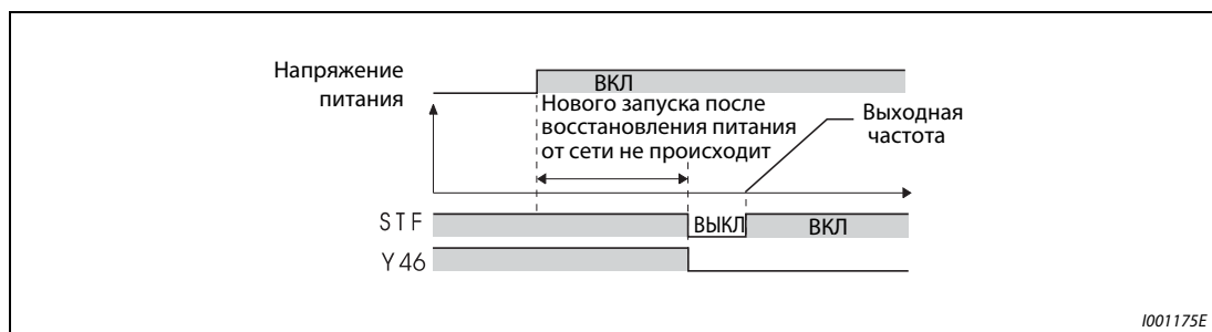
Рис. 6-90: Новый запуск при восстановлении питания
