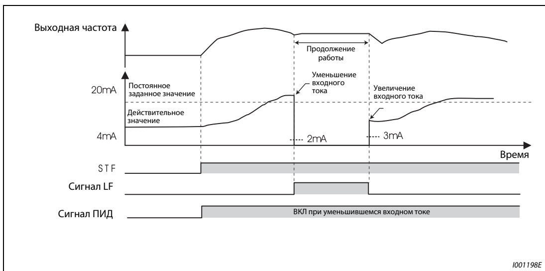
Рис. 6-121: Уменьшение заданного значения тока при ПИД-регулировании (обратный ход, пар. 573 = 1)
