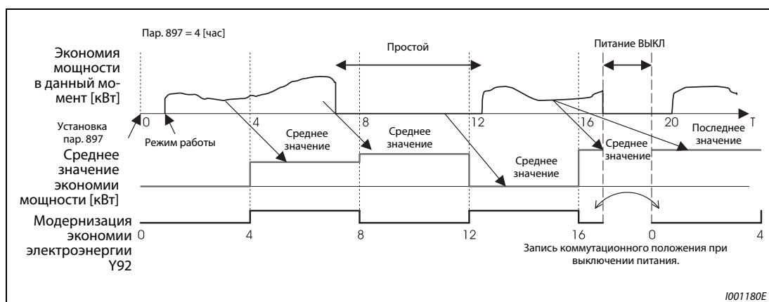
Рис. 6-98: Модернизация экономии электроэнергии
