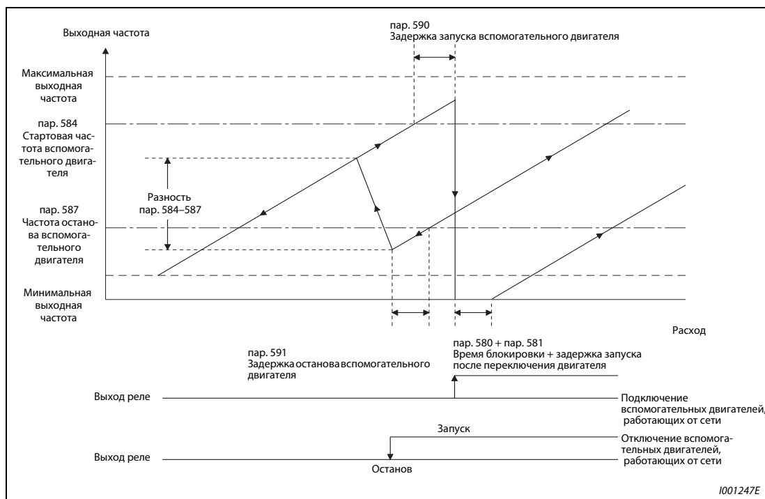
Рис. 6-180: Схема последовательности действий при запуске и останове вспомогательного двигателя 1
