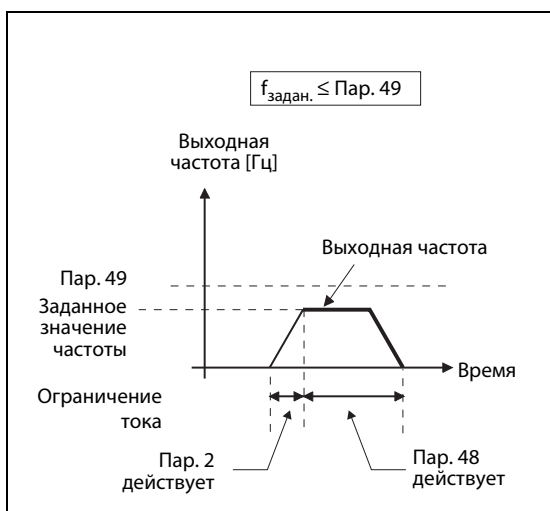
Рис. 6-8: Предельное значение тока, в случае если номинальное значение частоты меньше или равно значению, заданному параметром 49.
