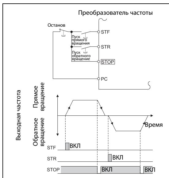
Рис. 6-60: Управление по 3-жильному проводу цепи управления (пар. 250 = 9999)
