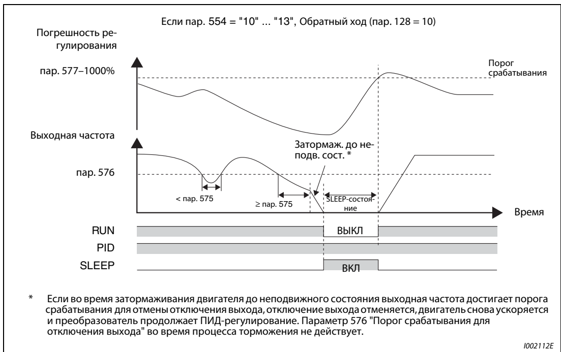
Рис. 6-183: Отключение выхода (функция SLEEP), если пар. 554 = "10" ... "13", пар. 128 = "10 "
