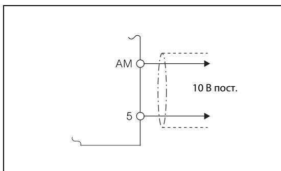
Рис. 6-80: Подключение аналогового индикатора к выходу АМ
