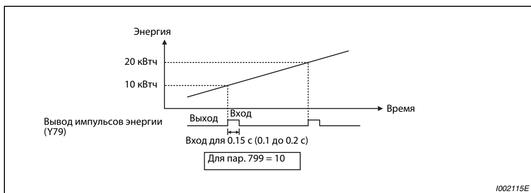
Рис. 6-70: Задание величины шага для вывода значения энергии (сигнал Y79, пар. 799)
