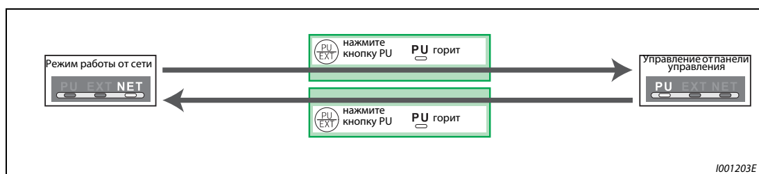
Рис. 6-127: Переключение режима работы при пар. 340 = 10 или 12
