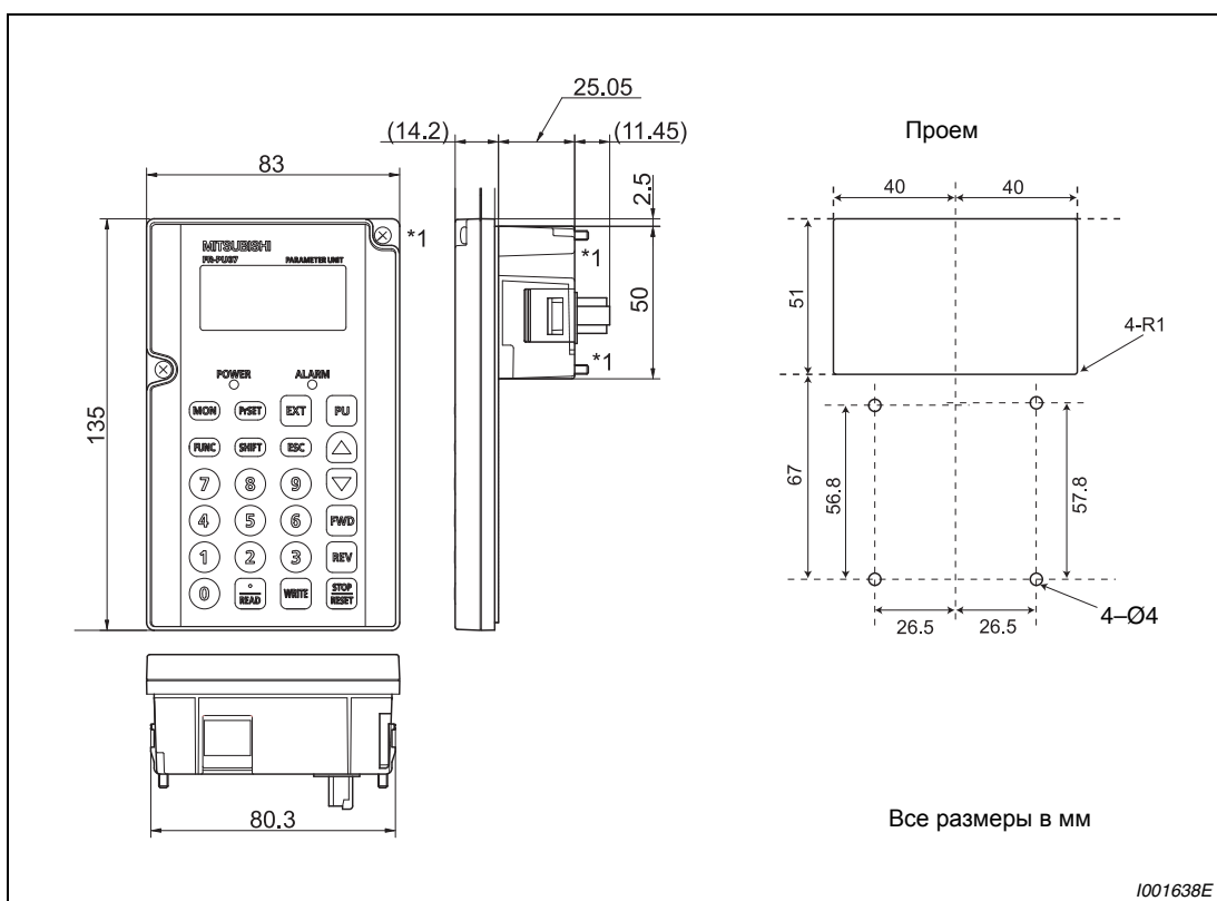
Рис. А-22: Панель управления FR-PU07
