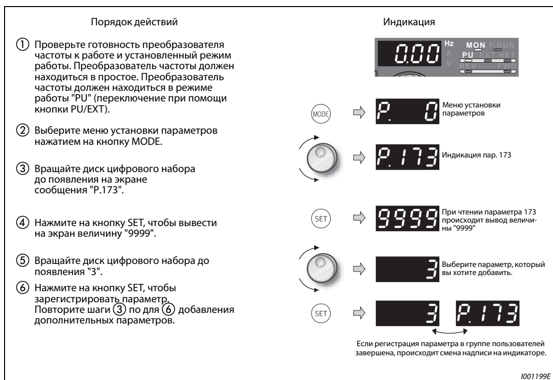
Рис. 6-123: Включение параметра 3 в группу пользователей
