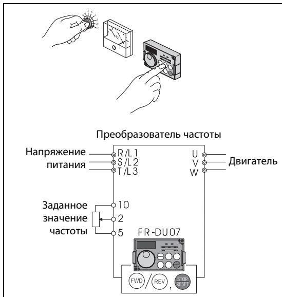
Рис. 6-131: Комбинированный режим работы 2
