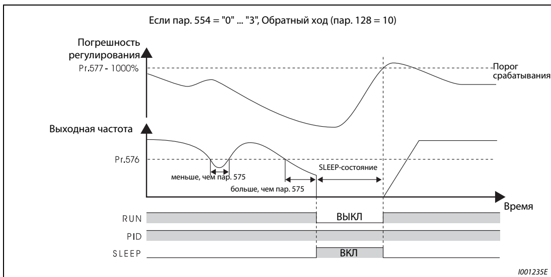
Рис. 6-166: Отключение выхода (SLEEP-функция), если пар. 554 = "0" ... "3"
