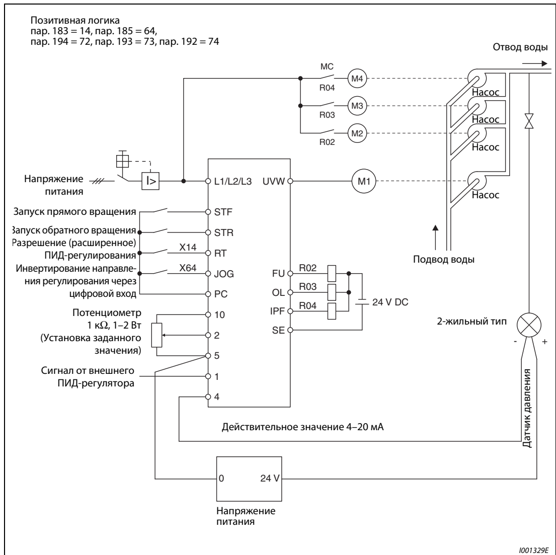
Рис. 6-177: Расширенное ПИД-регулирование (стандартный режим работы)
