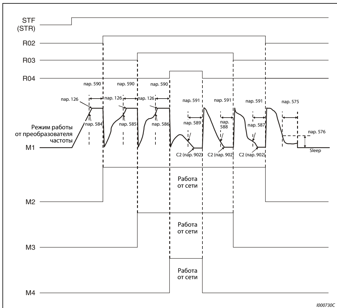
Рис. 6-184: Переходная характеристика в стандартном режиме работы
