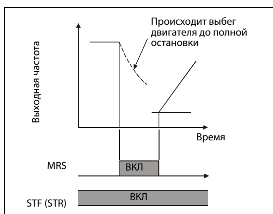
Рис. 6-54: Блокировка регулятора
