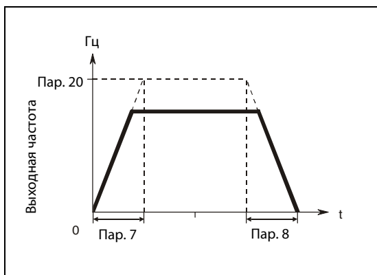
Рис. 6-30: Время разгона/замедления
