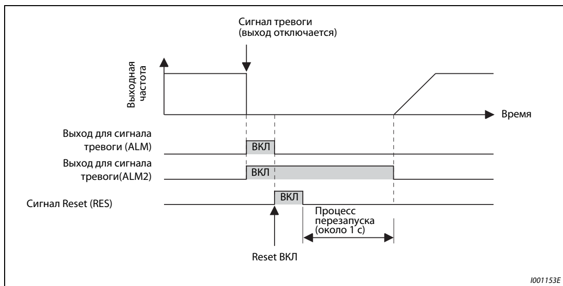
Рис. 6-63: Сигналы тревоги
