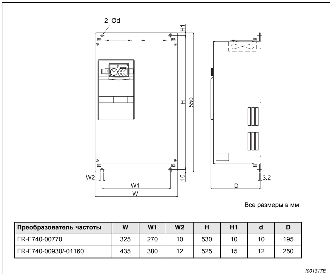
Рис. А-4: Размеры от FR-F740-00770 до -01160
