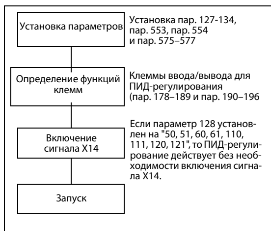
Рис. 6-168: Метод установки
