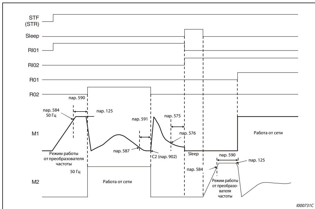
Рис. 6-185: Переходная характеристика при переменном режиме работы
