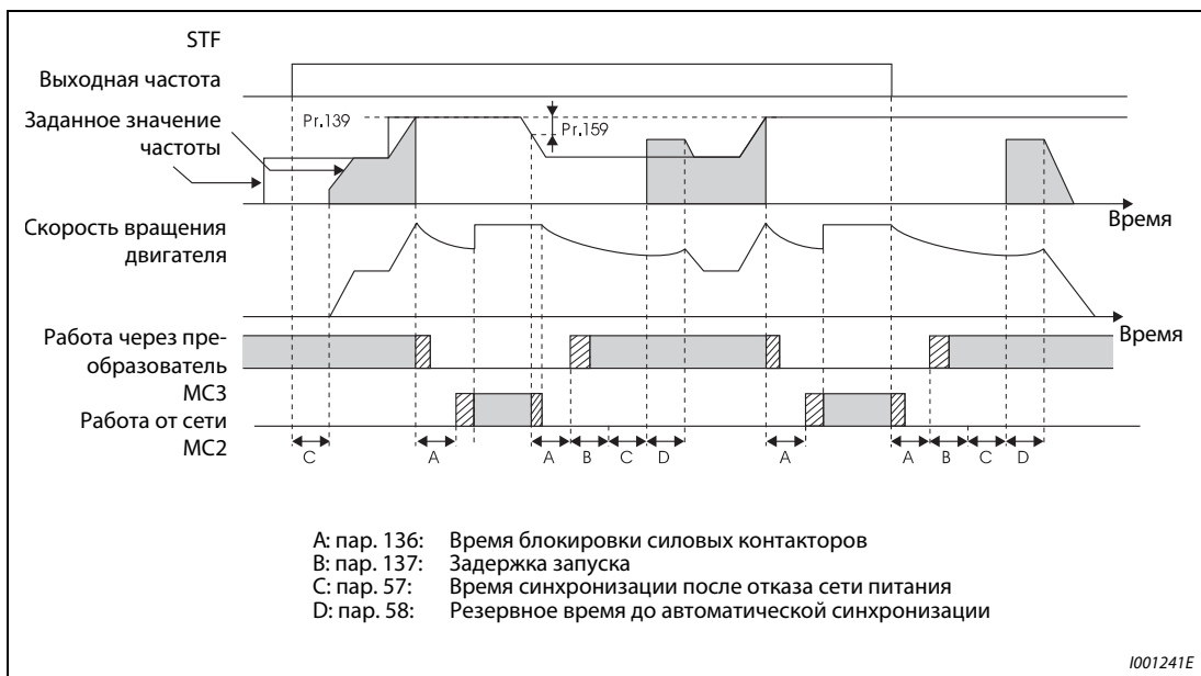
Рис. 6-174: Временная диаграмма сигналов с автоматическим переключением в режим работы от сети
