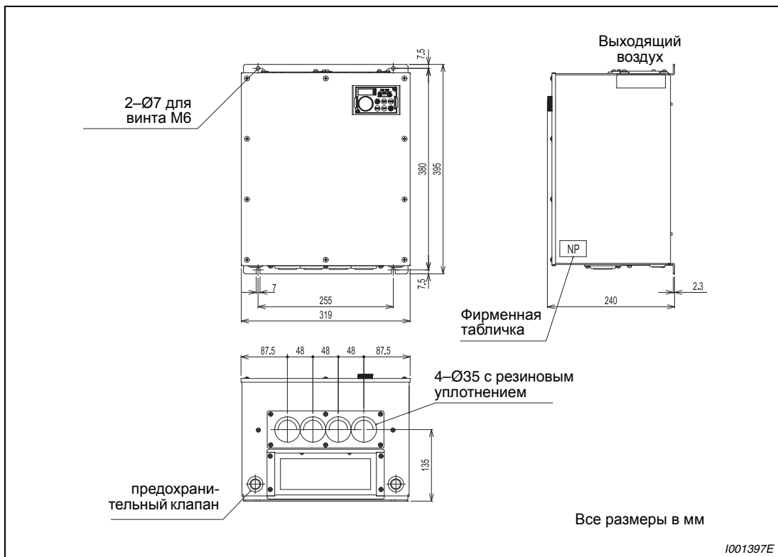
Рис. А-11: Размеры FR-F746-00170 и -00250
