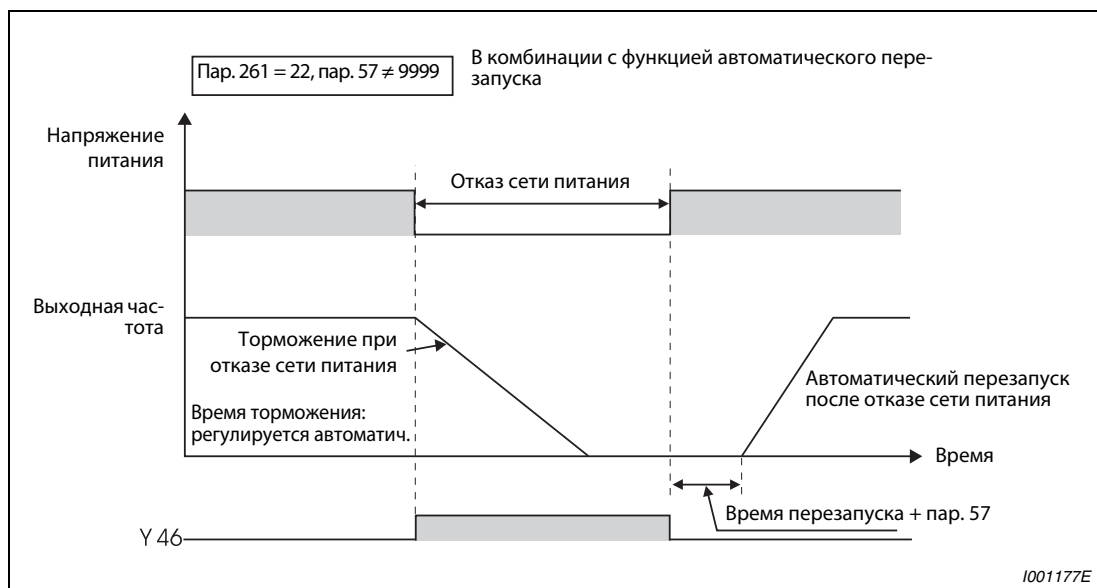
Рис. 6-95: Продолжение работы после отказа сети питания (пар. 261 = 22, пар. 57 ≠ 9999)
