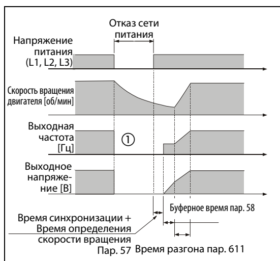
Рис. 6-83: Автоматический перезапуск с определением выходной частоты (пар. 162 = 0/10)
