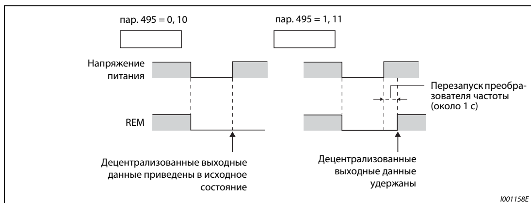
Рис. 6-69: Децентрализованные выходные данные при выключении питания.
