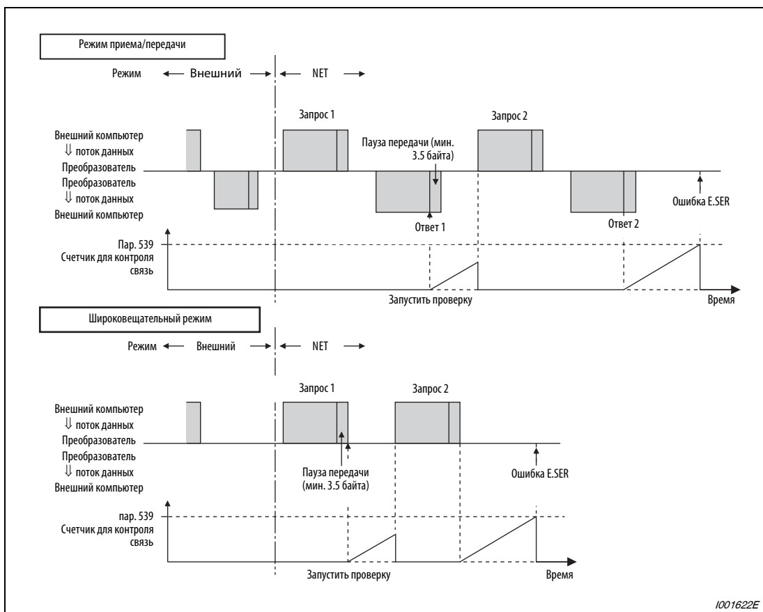
Рис. 6-156: Контроль потери связи
