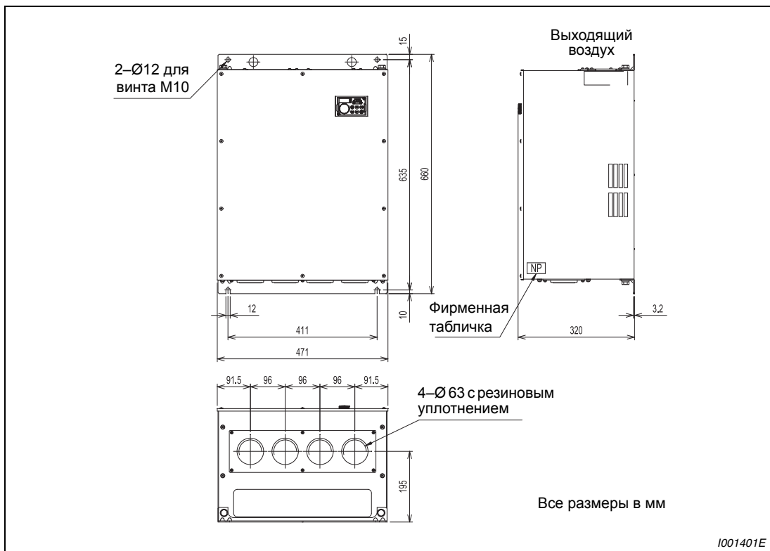
Рис. А-15: Размеры FR-F746-00930 и -01160
