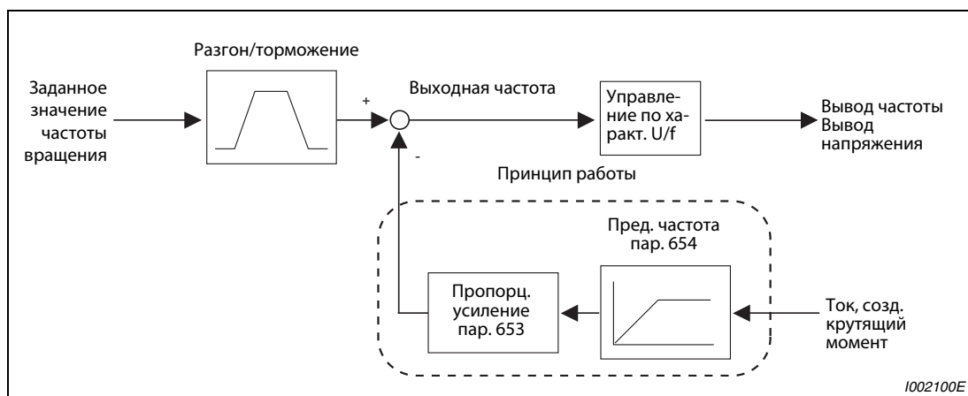
Рис. 6-100: Принцип подавления вибрации
