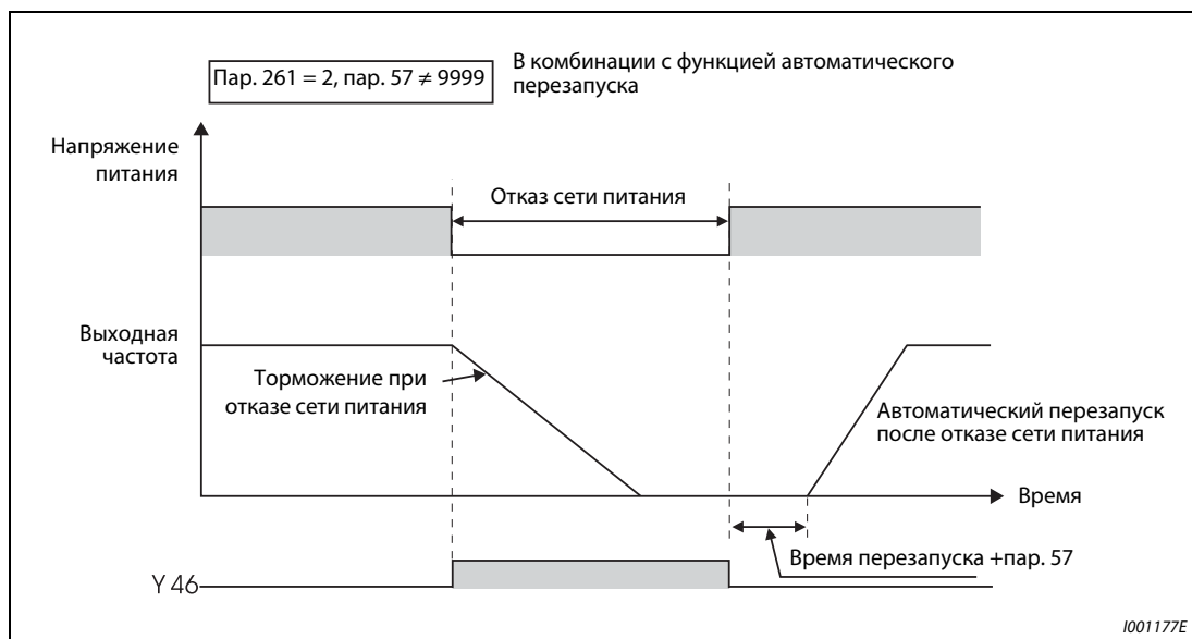
Рис. 6-92: Продолжение работы после отказа сети.
