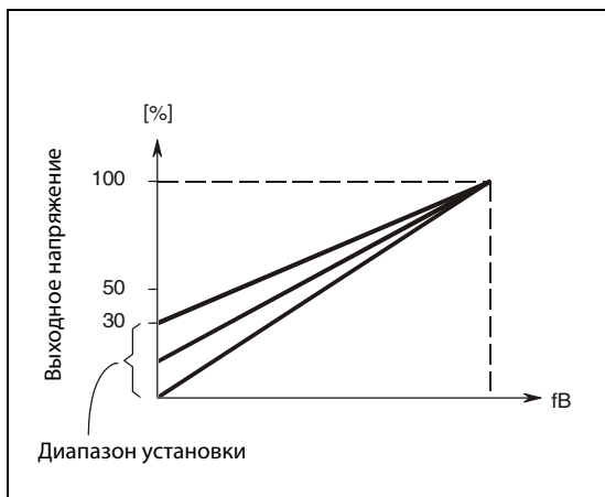
Рис. 6-1: Отношение выходной частоты к выходному напряжению
