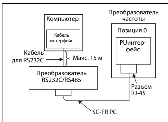
Рис. 6-135: Подключение компьютера с интерфейсом RS485 к интерфейсу PU
