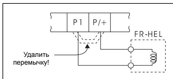
Рис.3-34: Подключение дросселя промежуточного контура
