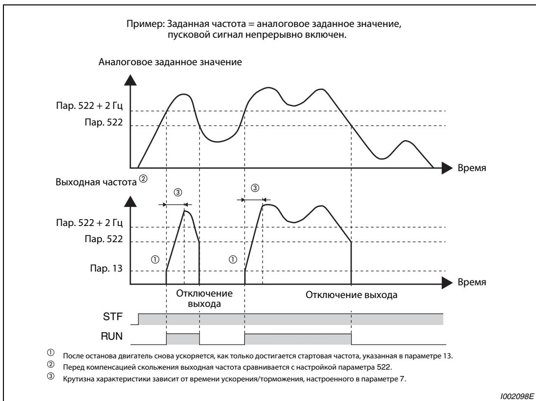
Рис. 6-53: Пример 2: Заданная частота = аналоговое заданное значение, пусковой сигнал непрерывно включен
