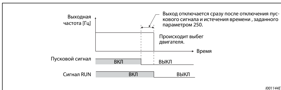
Рис. 6-51: Способ останова при пар. 250 ≠ 8888 или 9999
