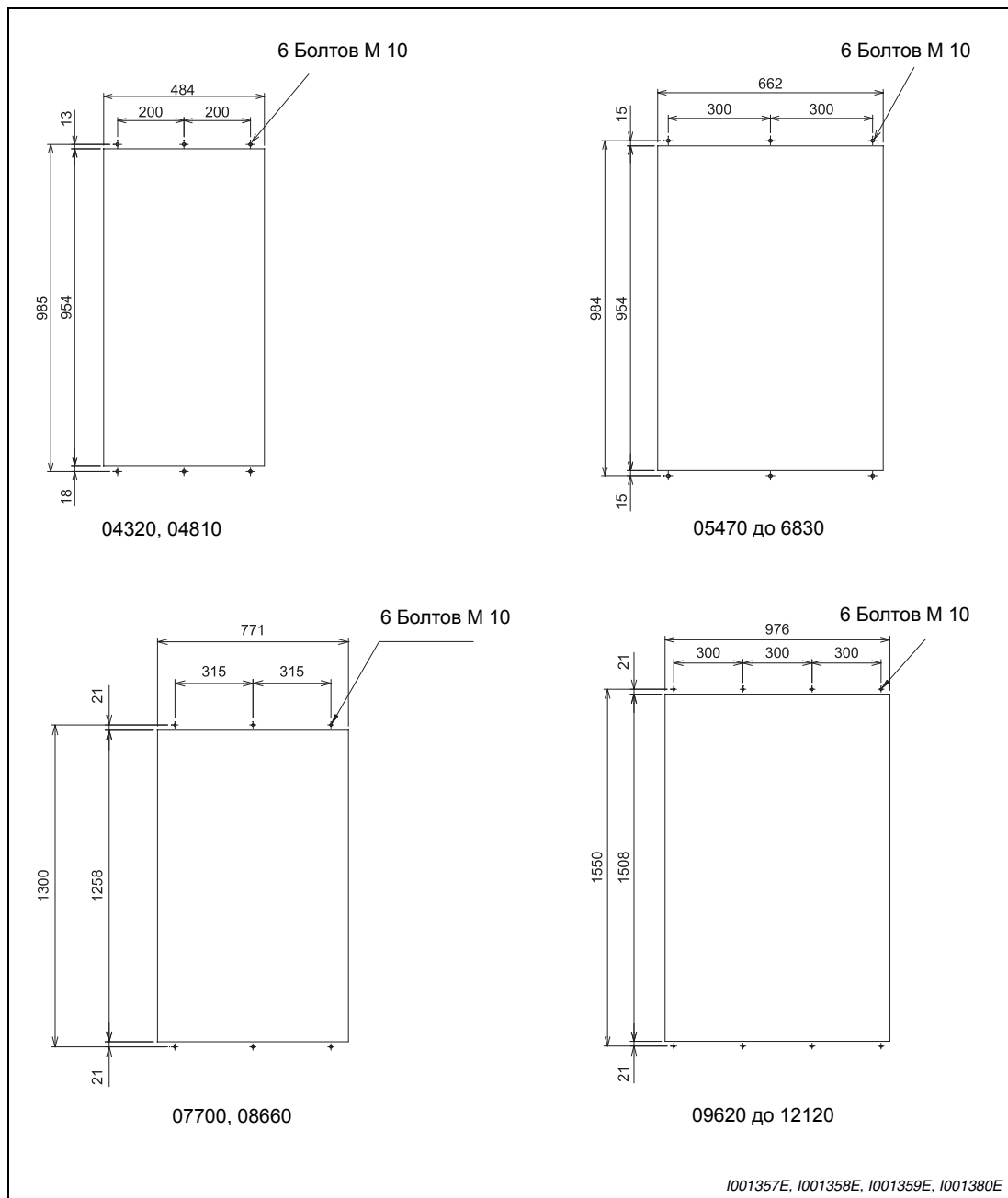
Рис. 20-1: Размеры проема в распределительном шкафу
