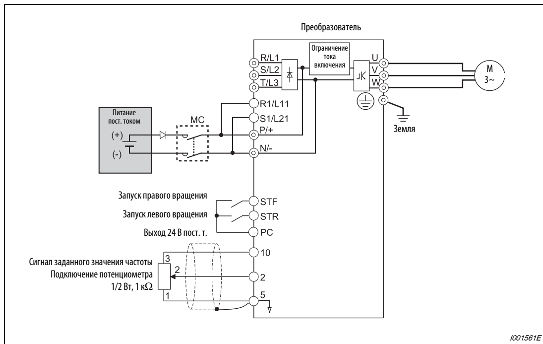
Рис. 6-46: Пример подключения для варианта 1 питания контура постоянного тока
