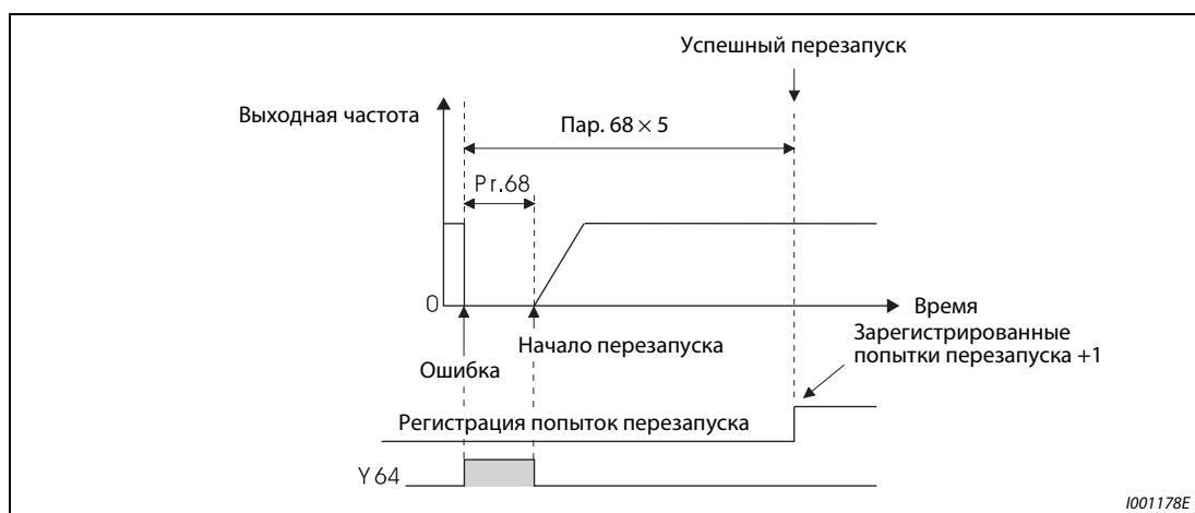
Рис. 6-96: Пример успешно выполненного перезапуска
