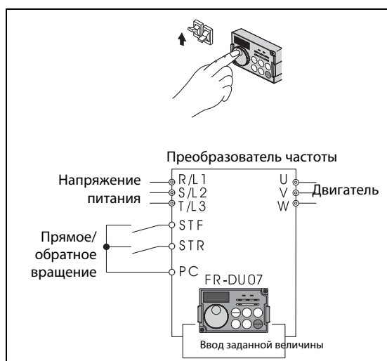
Рис. 6-130: Комбинированный режим работы 1
