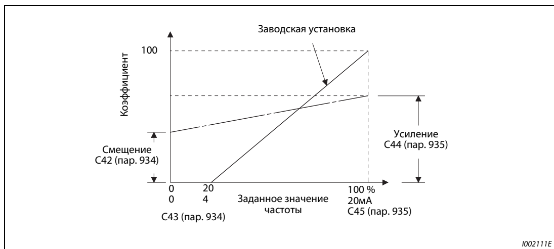
Рис. 6-170: Смещение и усиление для ПИД-индикации
