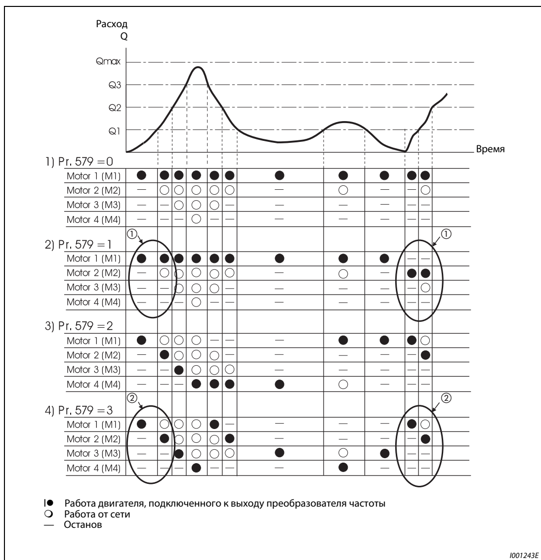
Рис. 6-176: Регулирование расхода жидкости через вспомогательные двигатели
