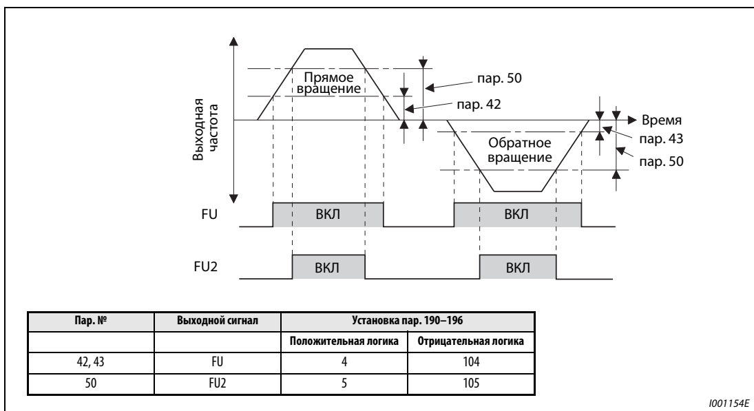
Рис. 6-65: Контроль частоты при прямом и обратном вращении
