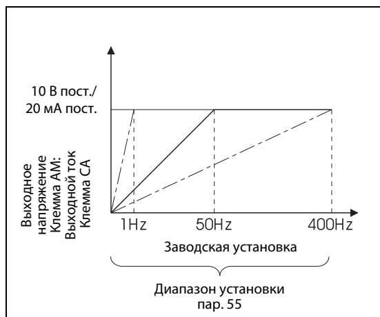
Рис. 6-76: Опорная величина для внешней индикации частоты
