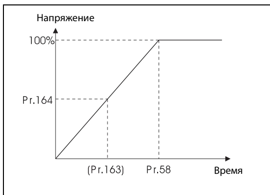
Рис. 6-85: Увеличение напряжения при автоматическом перезапуске
