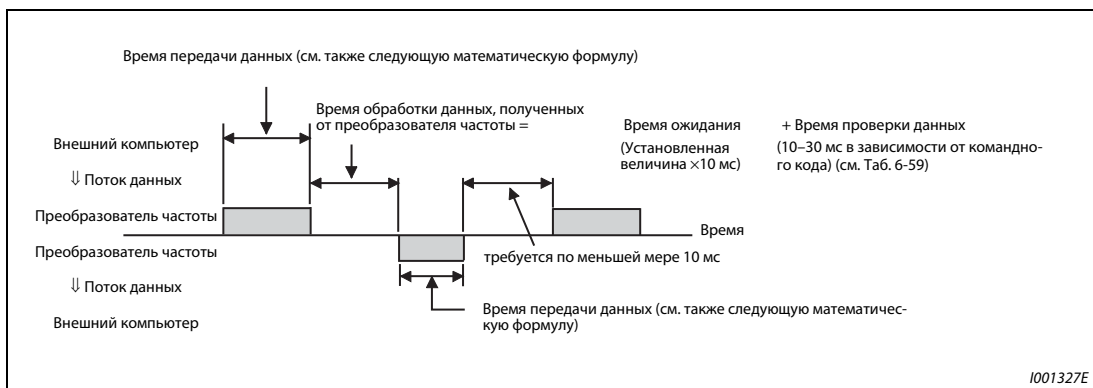
Рис. 6-147: Время передачи данных
