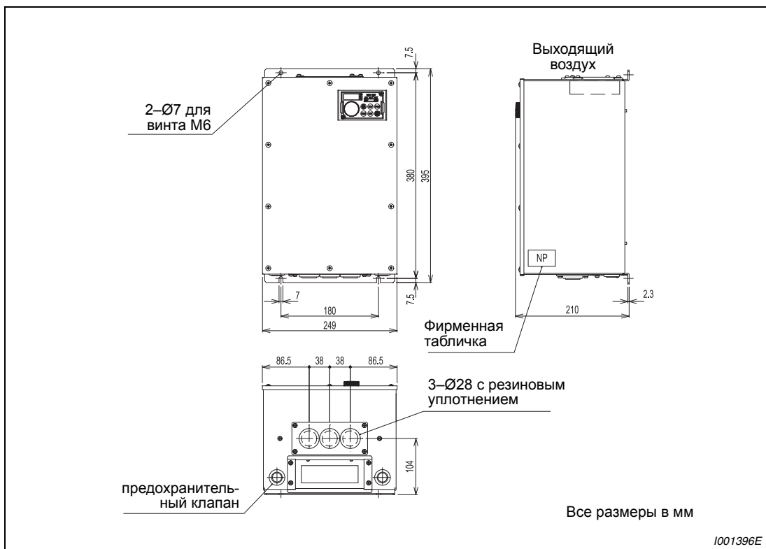
Рис. А-10: Размеры от FR-F746-00023 до -00126
