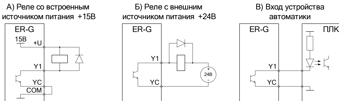
Рисунок 6 – Подключение выходов типа «открытый коллектор» Y1
