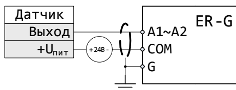
Рисунок 7 – Типовые схемы подключения аналоговых входов АIN
