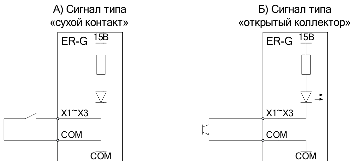
Рисунок 5 – Подключение дискретных входов X1...X3
