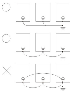
Соединение заземления
