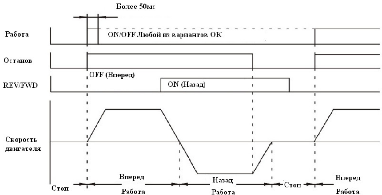
Схема последовательности сигналов процедуры 3-проводной системы
