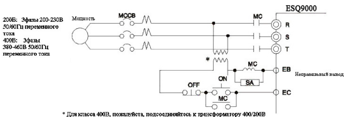
Установка размыкателя для прокладки проводов
