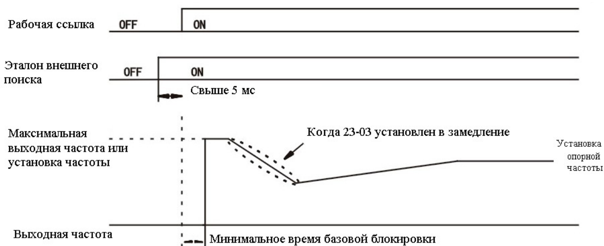
Схема последовательности сигналов эталона внешнего поиска.
