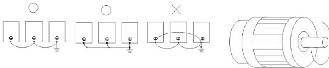
Инверсия
