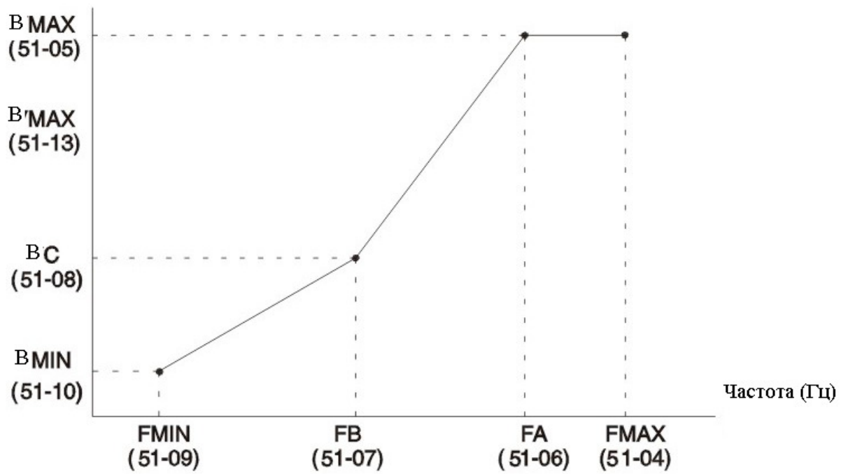
Кривая V/F (Напряжения/частоты)
