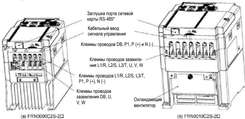
Рисунок 1.2. Внешний вид FRENIC-Mini
