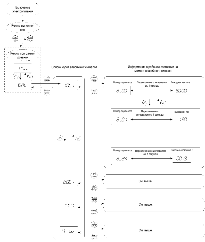
Рисунок 3.10 Переход состояний в меню «Информация аварии»
