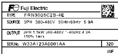
(a) Главный шильдик
