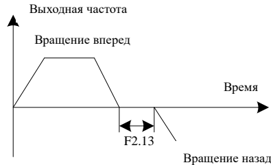
Рис. 6-6 Переключение вперед/назад
