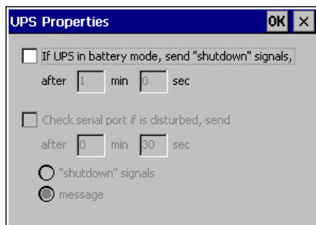
Рисунок 8-7 Параметры UPS [ИБП]
