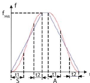
Диаграмма Кривой S ускорения и замедления
