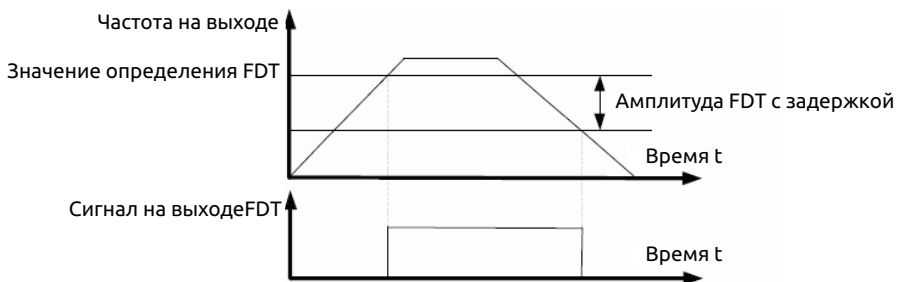
Схема сигнала F_ .
