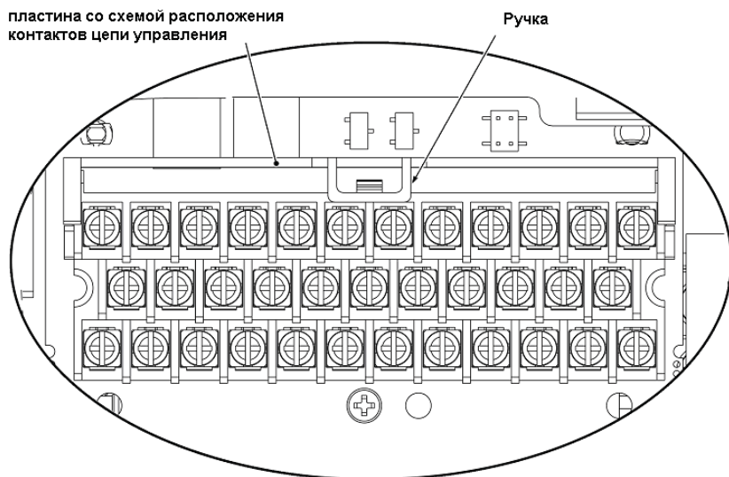
Рисунок 2.27 Открытие панели
