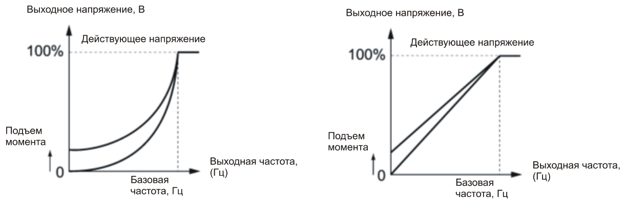
Переменный крутящий момент (F37 = 0)
