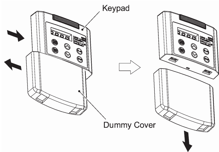
Рисунок 2.33 Снятие фальшпанели.
