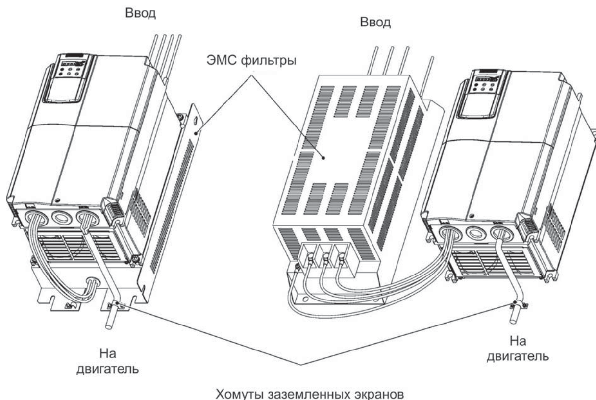
А) Установка под ПЧ
