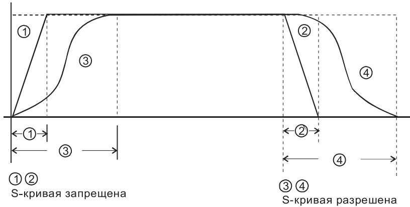
Характеристики разгона/торможения
