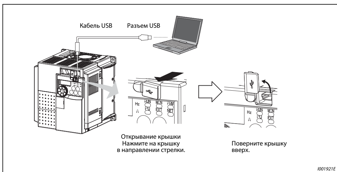
Рис. 6-132: Подключение к интерфейсу USB
