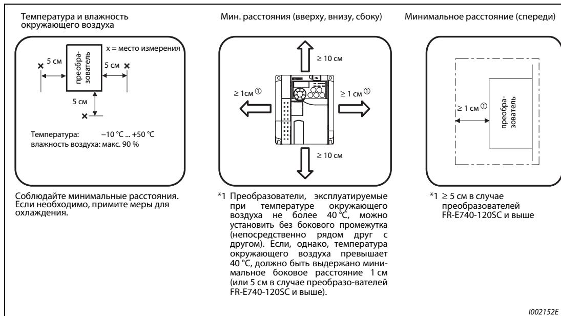
Рис. 2-9: Минимальные зазоры
