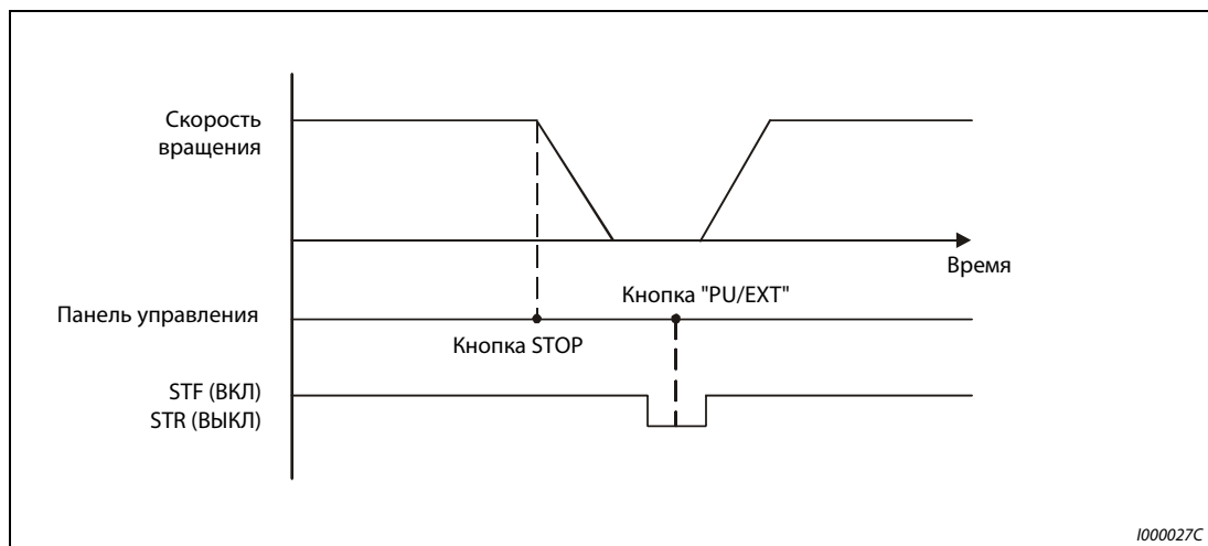
Рис. 6-99: Останов при работе в режиме внешнего управления
