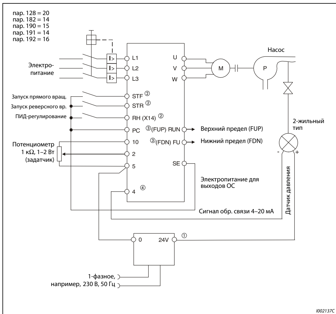
Рис. 6-139: Пример подключения при положительной логике
