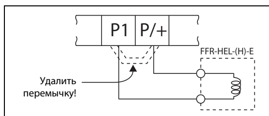
Рис. 3-34: Подключение дросселя постоянного тока
