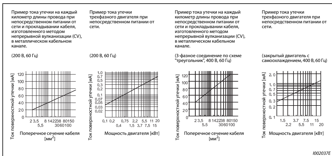
Рис. 3-37: Токи утечки
