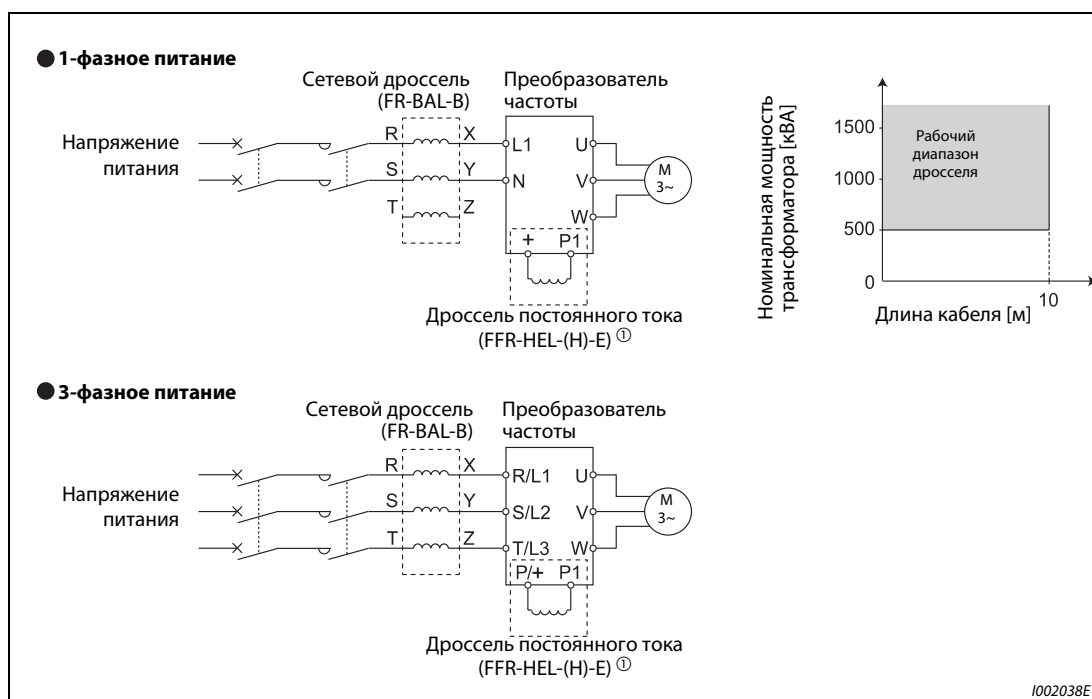
Рис. 3-35: Запуск и останов преобразователя частоты
