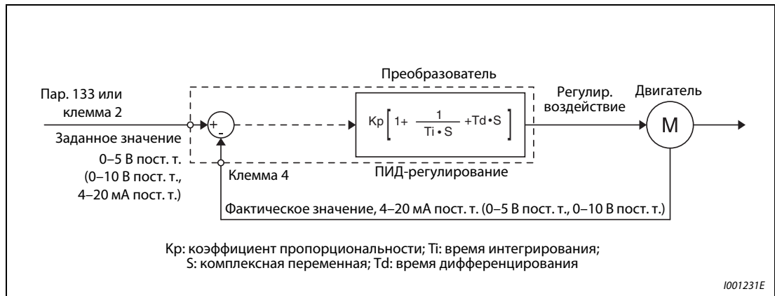
Рис. 6-133: Конфигурация системы для пар. 128 = 20 или 21 (подключение задания/сигнала обратной связи к преобразователю)
