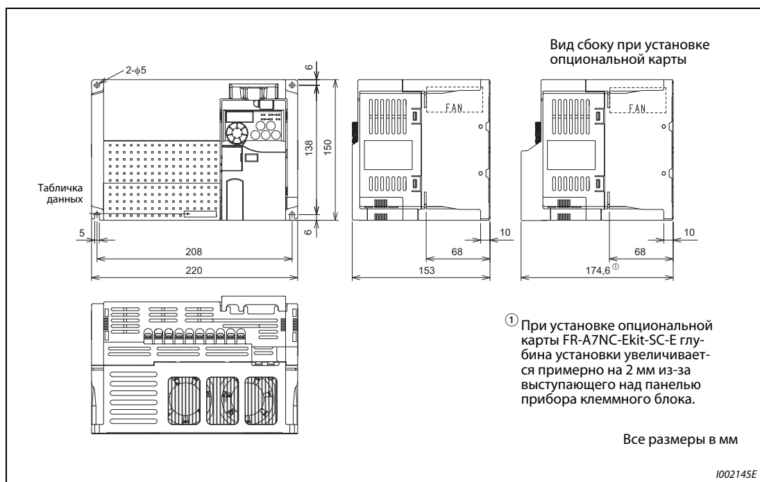
Рис. А-4: Размеры преобразователей частоты FR-E740-120SC и 170SC
