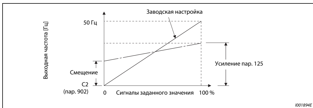
Рис. 6-147: Компенсация сигнала на клемме 2
