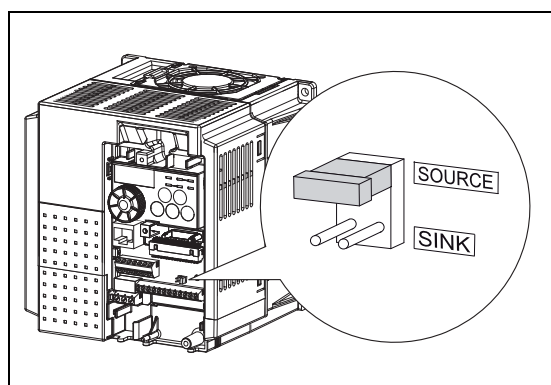
Рис. 3-17: Выбор логической схемы управления
