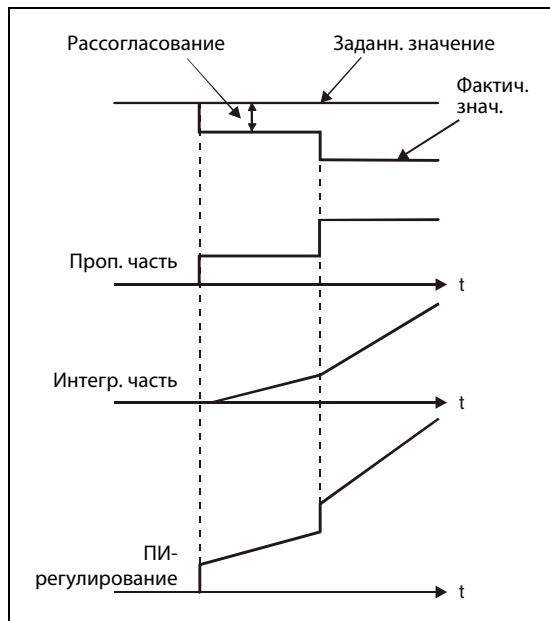
Рис. 6-134: Принцип действия ПИ-регулятора
