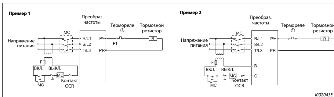
Рис. 3-28: Защитные схемы
