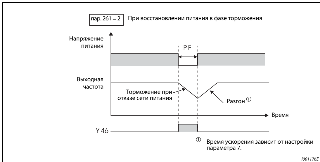
Рис. 6-85: Продолжение работы после отключения сети
