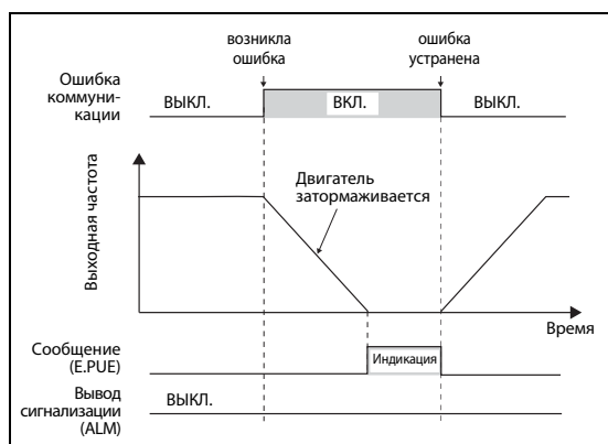
Рис. 6-121: Характер работы при пар. 502 = "2"
