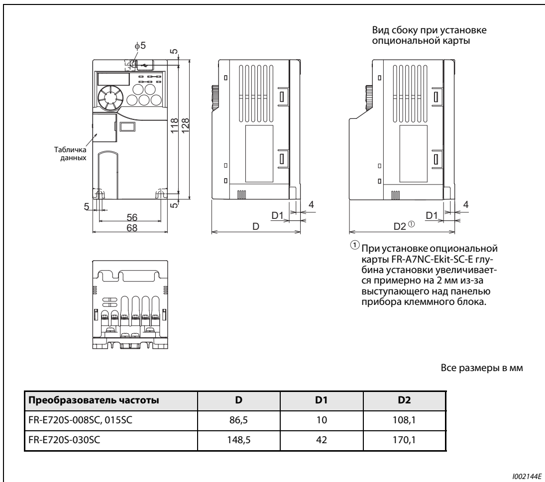
Рис. А-1: Размеры преобразователей частоты FR-E720S-008SC ...030SC
