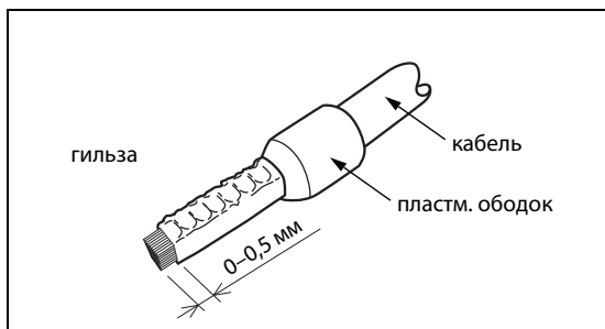
Рис. 3-8: Крепление оконцовочной гильзы
