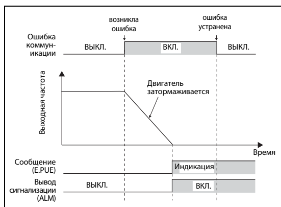
Рис. 6-120: Характер работы при пар. 502 = "1"
