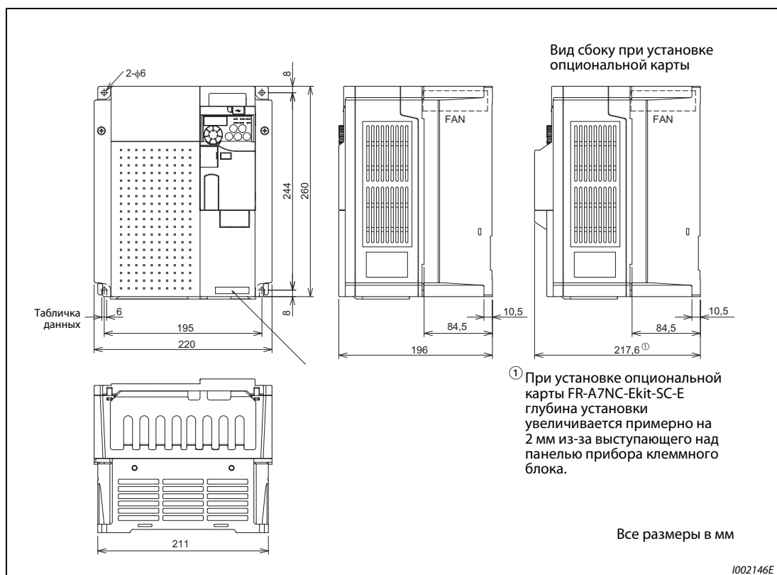
Рис. А-5: Размеры преобразователя частоты FR-E740-230SC и 300SC
