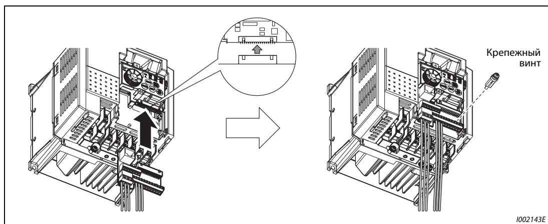
Рис. 8-8: Установка клеммного блока
