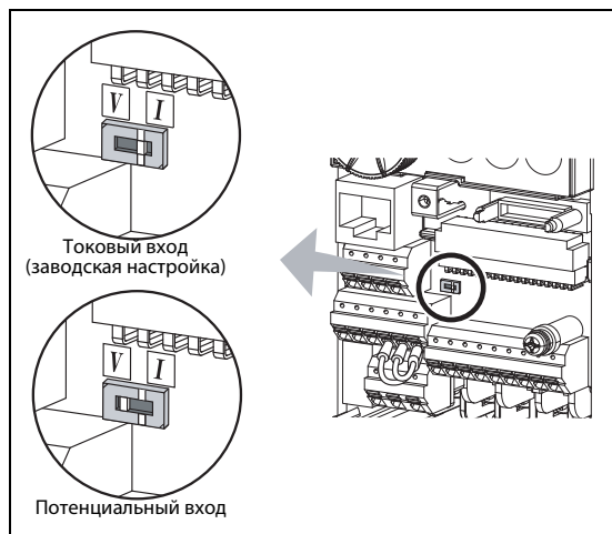
Рис. 6-90: Переключатель "Потенциальный/токовый вход"
