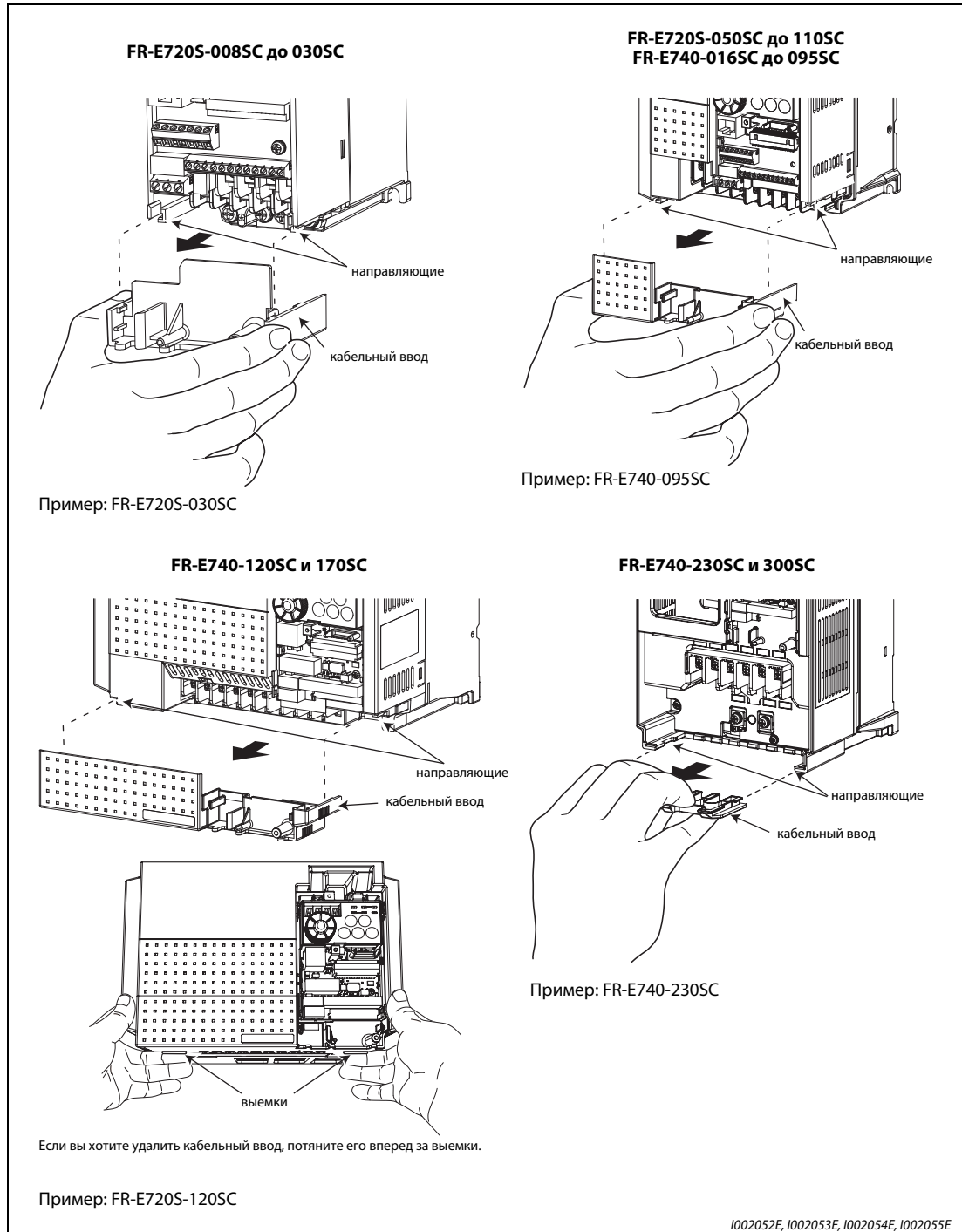
Рис. 2-5: Примеры удаления кабельного ввода
