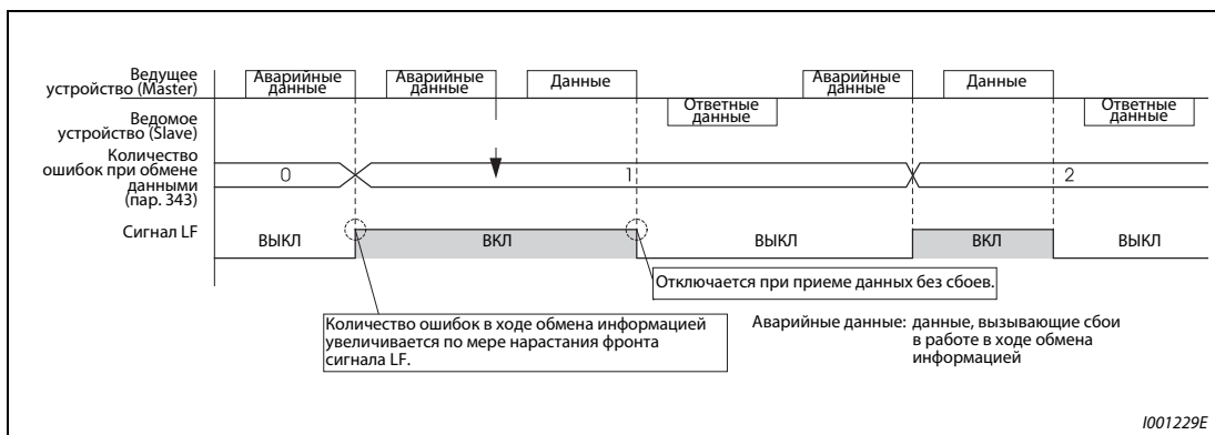
Рис. 6-131: Вывод сигнала LF
