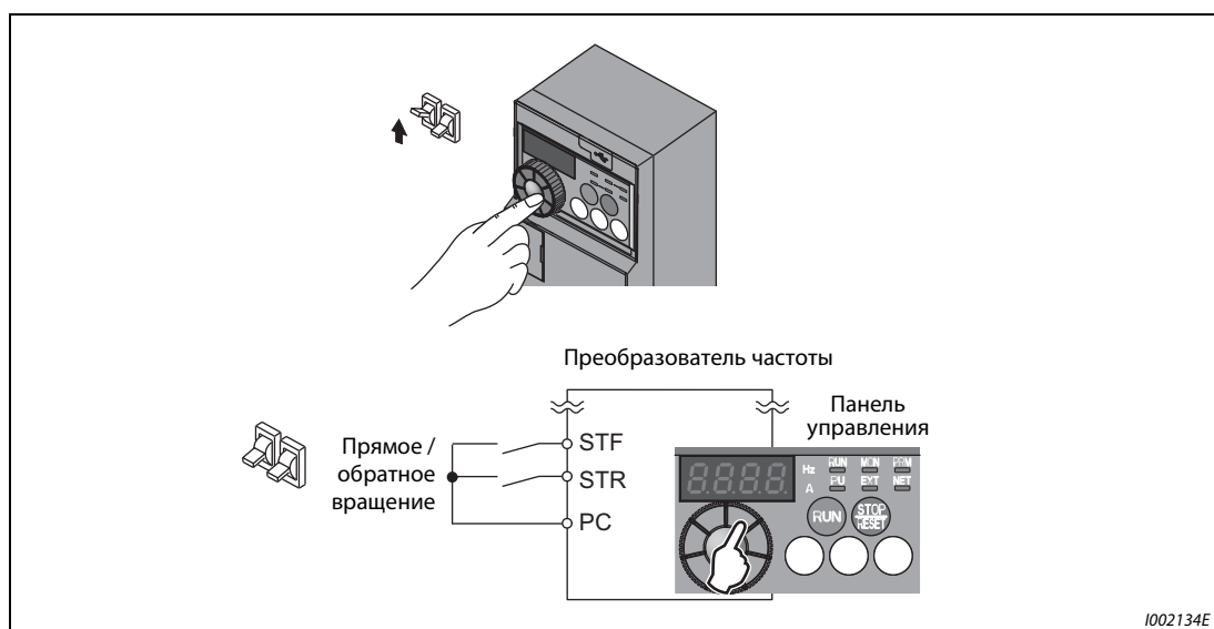
Рис. 6-107: Комбинированный режим работы 1
