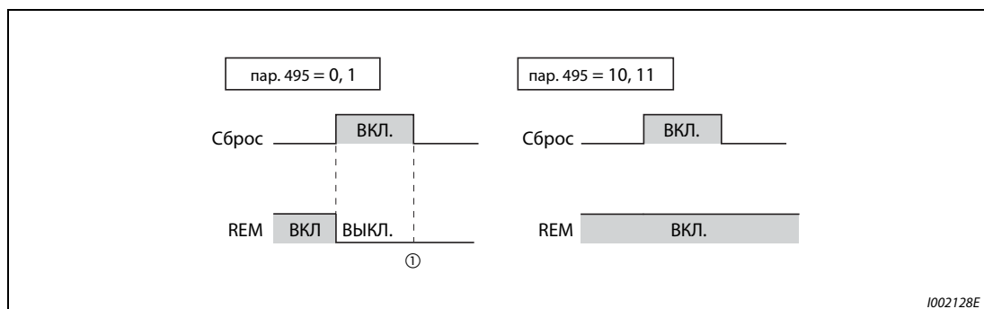
Рис. 6-67: Данные децентрализованного вывода при сбросе преобразователя частоты
