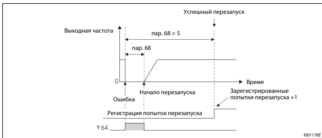
Рис. 6-87: Пример успешно выполненного перезапуска
