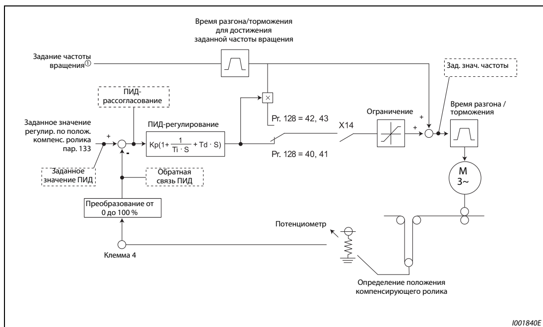
Рис. 6-144: Блок-схема регулирования по положению компенсирующего ролика
