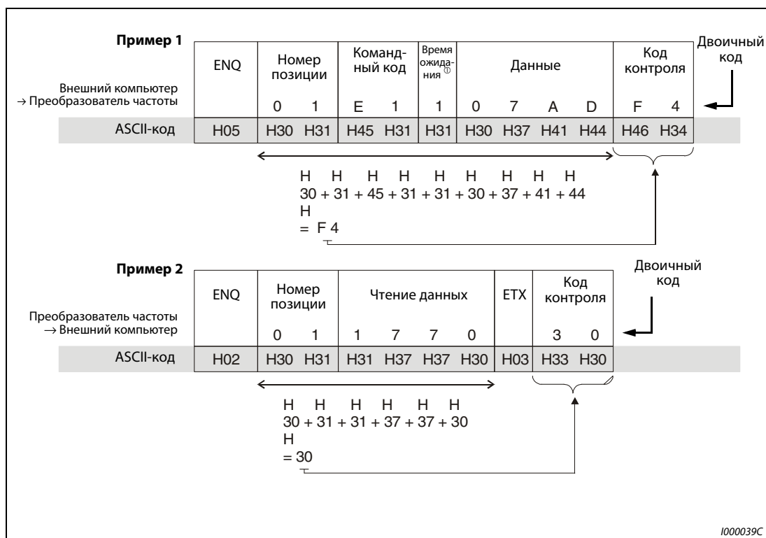
Рис. 6-124: Код контроля суммирования (примеры)
