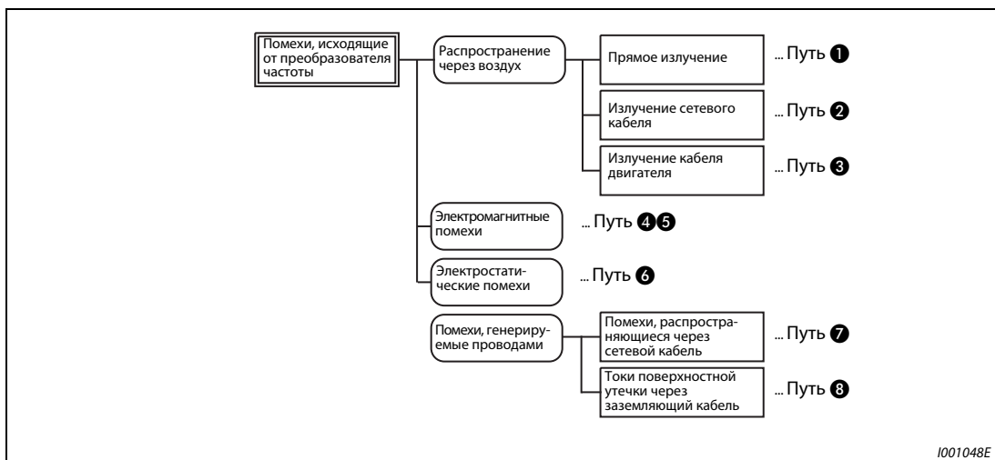
Рис. 3-38: Распространение помех
