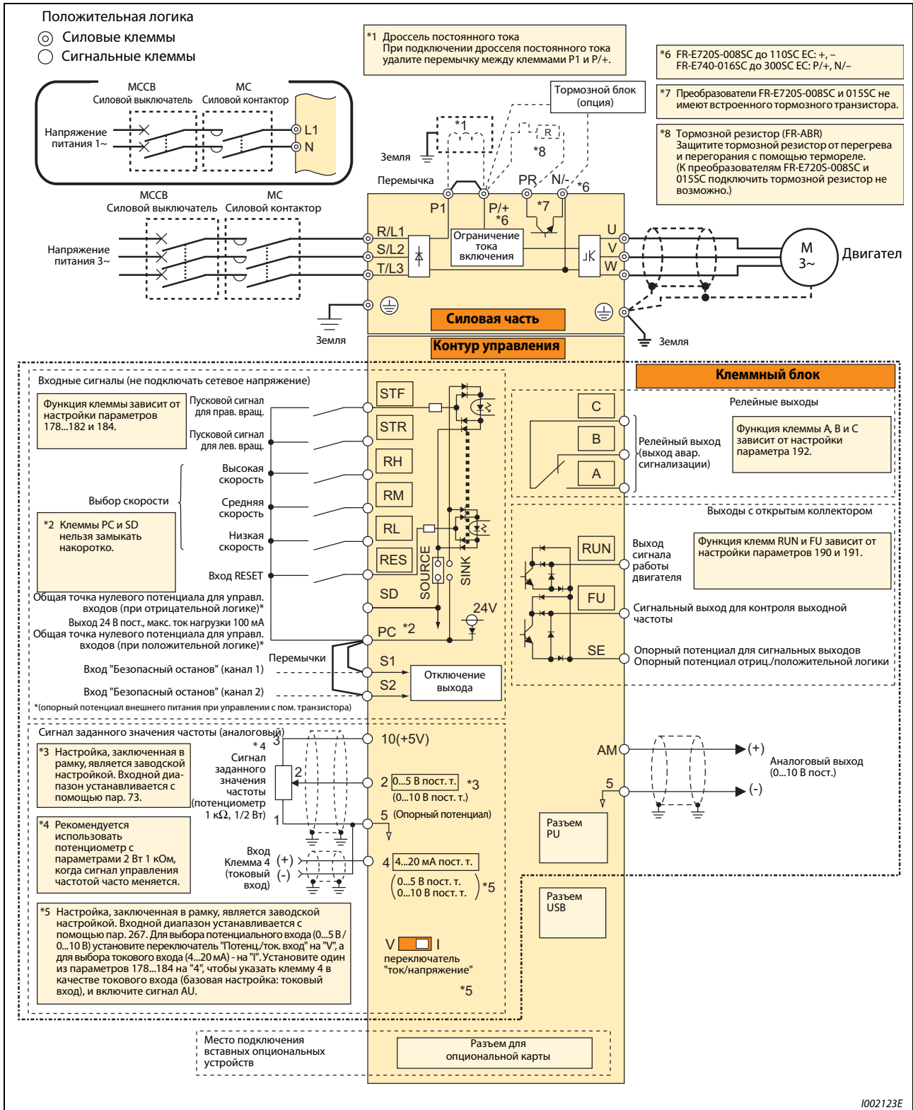
Рис. 3-3: Схема подключения преобразователя частоты
