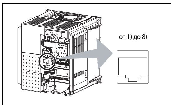
Рис. 6-109: Клеммы подключения панели управления (интерфейс PU)
