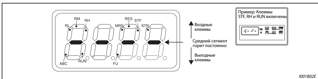
Рис. 6-70: Индикация коммутационных состояний клемм ввода/вывода
