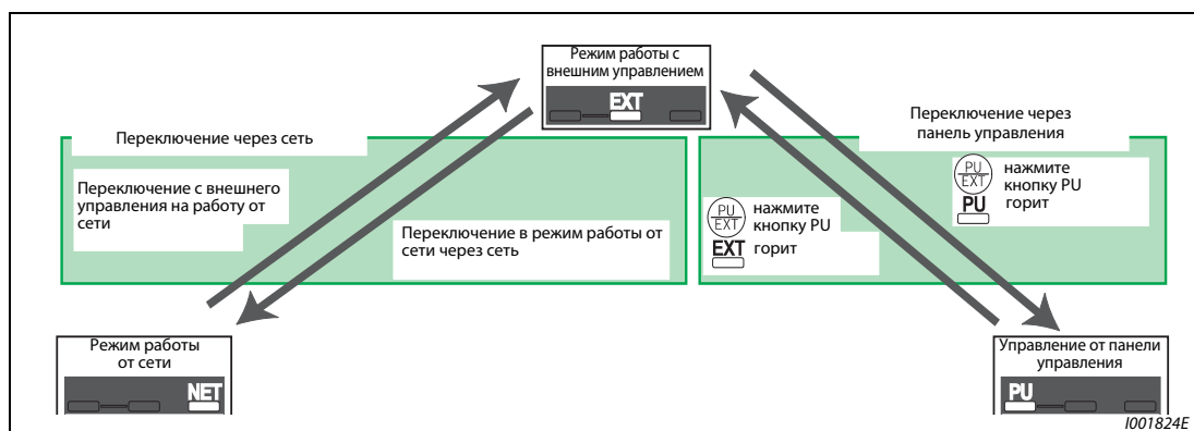
Рис. 6-103: Переключение режима работы при пар. 340 = 0, 1 или 2
