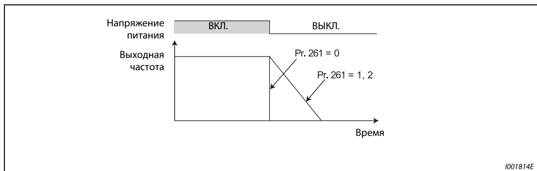
Рис. 6-82: Параметры для выбора способа останова при отказе сети питания
