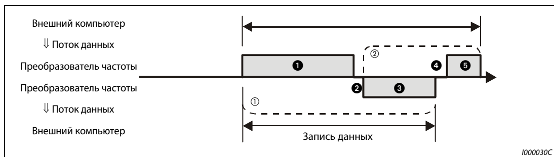
Рис. 6-122: Схематическое представление обмена данными
