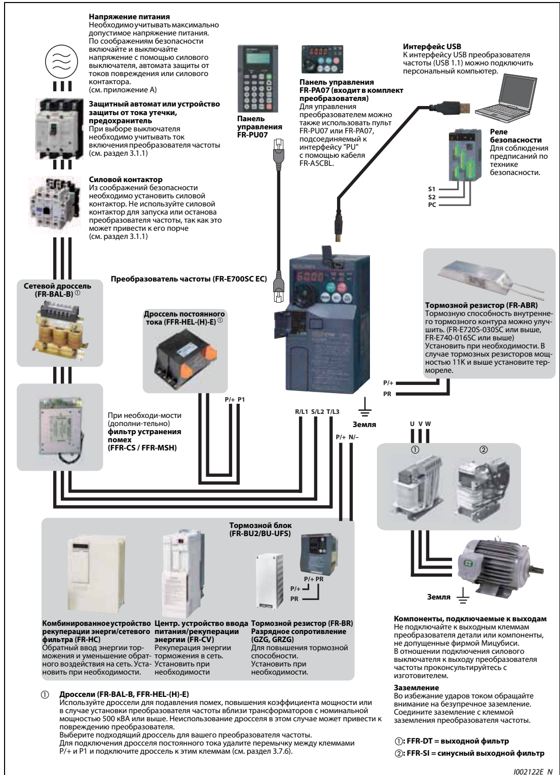
Рис. 3-1: Описание конфигурации системы
