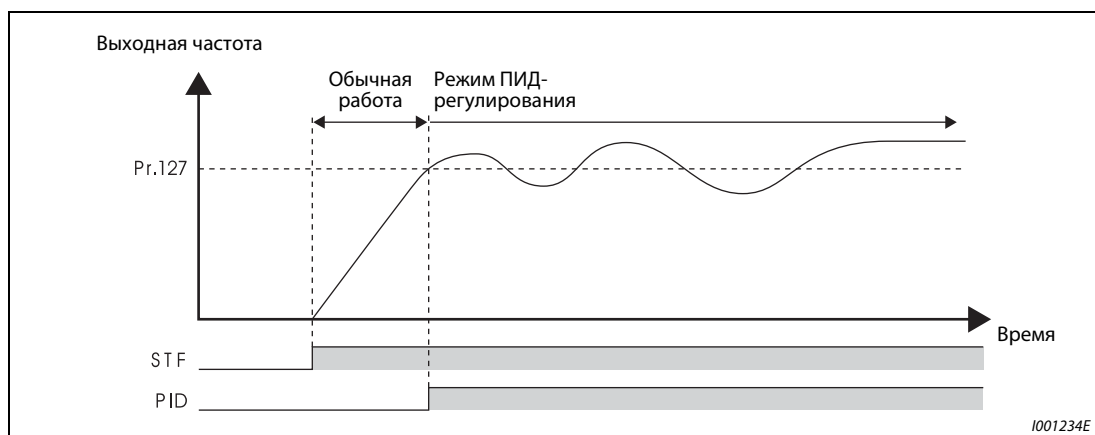
Рис. 6-140: Автоматическое переключение в режим ПИД-регулирования
