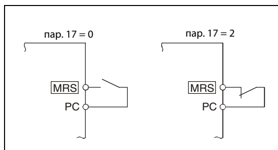
Рис. 6-52: Подключение сигнала MRS при положительной логике
