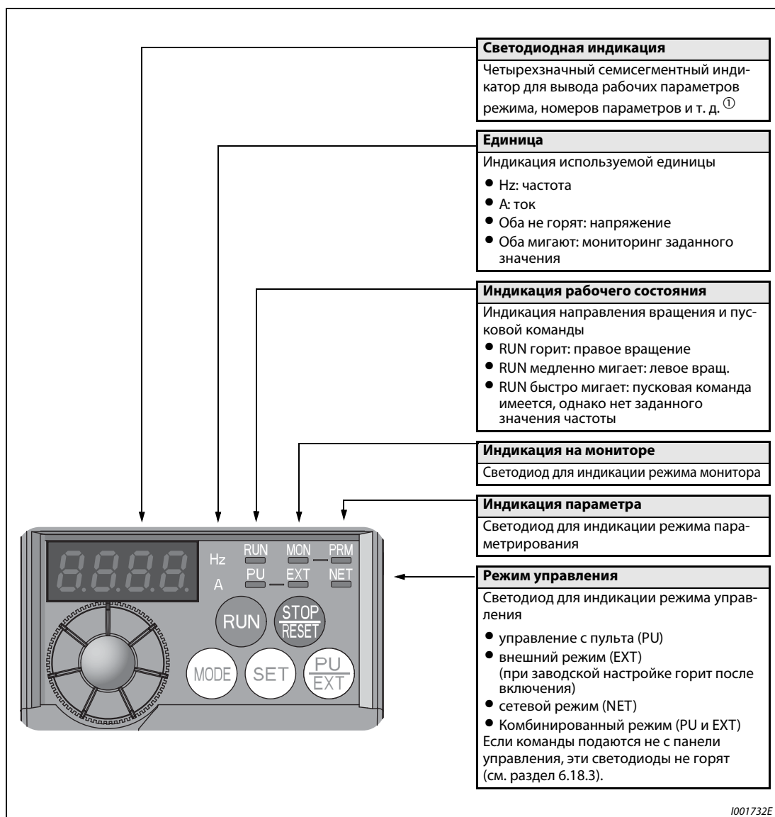
Рис. 4-6: Пульт управления преобразователя FR-E700SC
