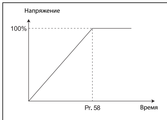
Рис. 6-81: Увеличение напряжения при автоматическом перезапуске
