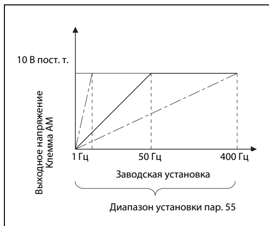
Рис. 6-73: Опорная величина для внешней индикации частоты
