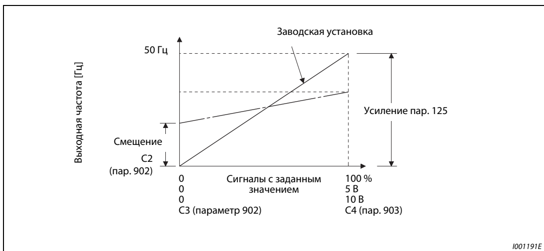
Рис. 6-94: Подгонка сигнала на клемме 2
