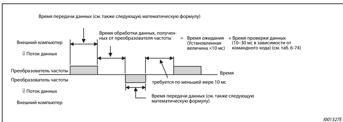
Рис. 6-125: Время передачи данных
