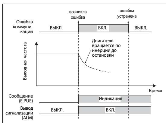
Рис. 6-119: Характер работы при пар. 502 = "0" (заводская настройка) или "3"
