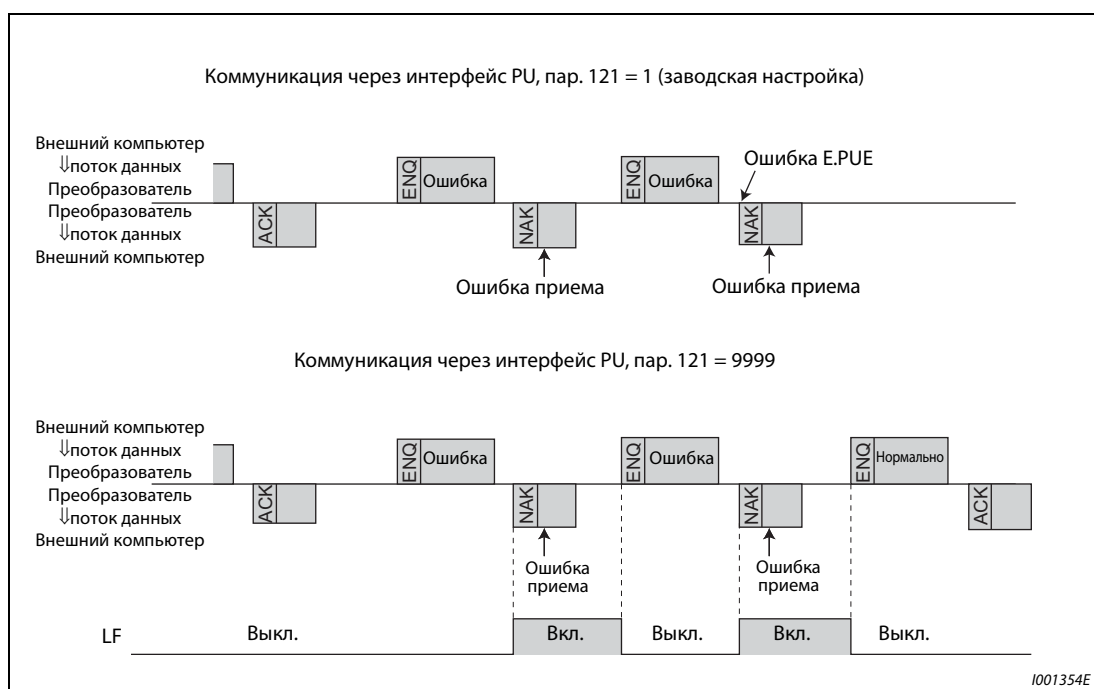
Рис. 6-117: Ошибки передачи данных
