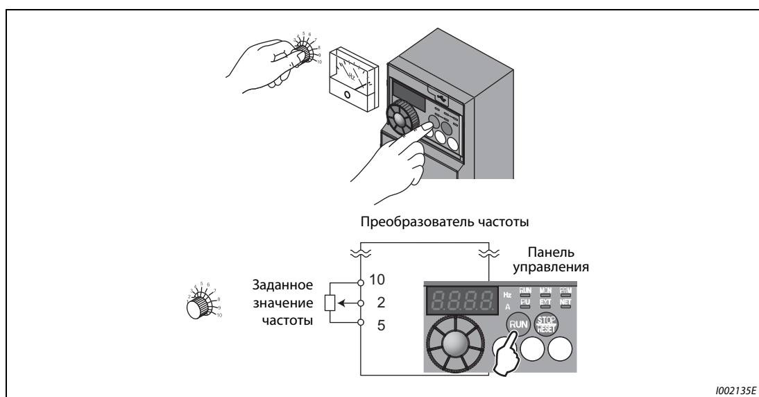
Рис. 6-108: Комбинированный режим работы 2
