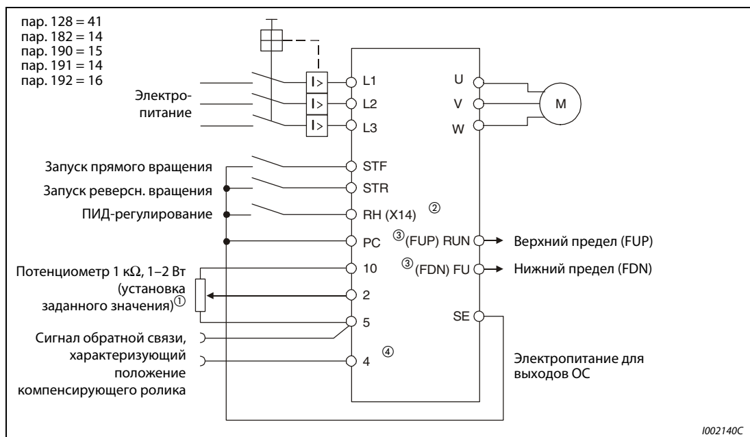
Рис. 6-146: Пример подключения при положительной логике
