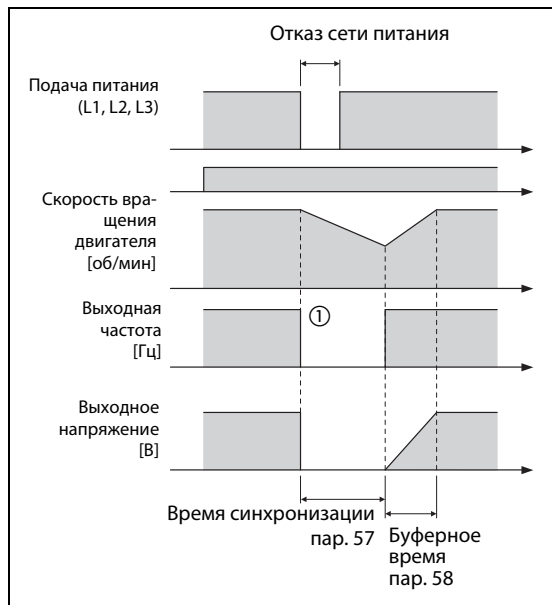
Рис. 6-79: Автоматический перезапуск без определения выходной частоты (пар. 162 = 1/11)
