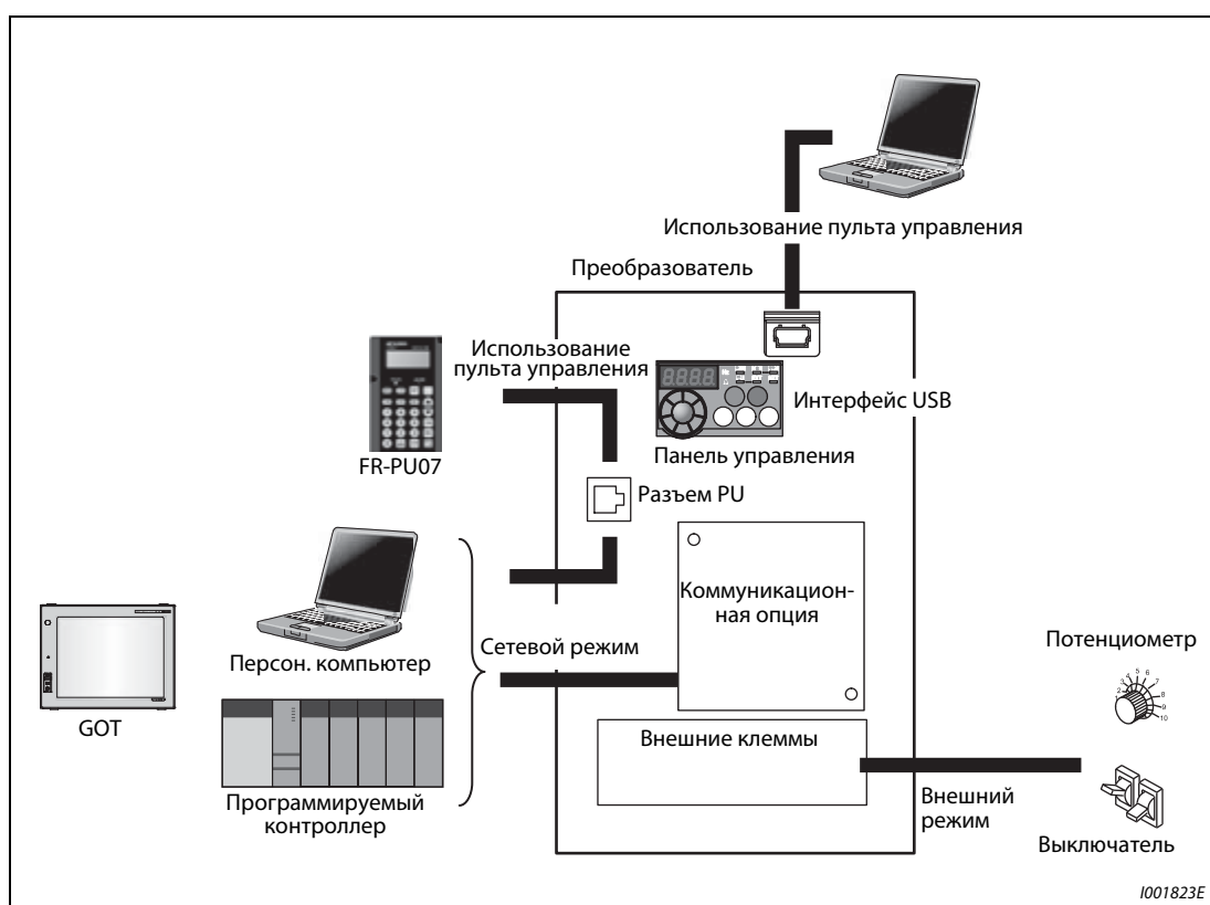
Рис. 6-102: Режимы работы преобразователя частоты
