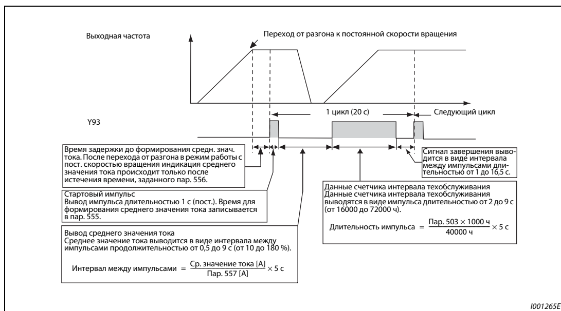
Рис. 6-156: Вывод импульсного сигнала Y93
