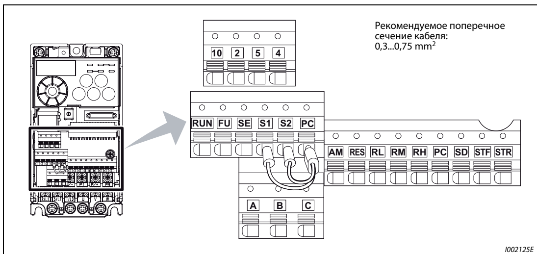
Рис. 3-6: Расположение клемм
