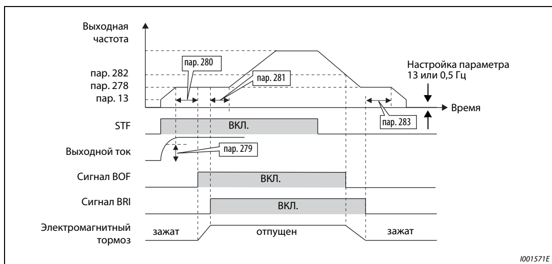
Рис. 6-49: Работа с параметром 292 = 7
