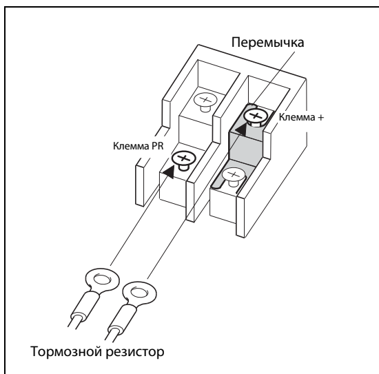
Рис. 3-25: Подключение тормозного резистора к клеммам + и PR преобразователя частоты FR-E720S-050SC ...FR-E720S-110SC
