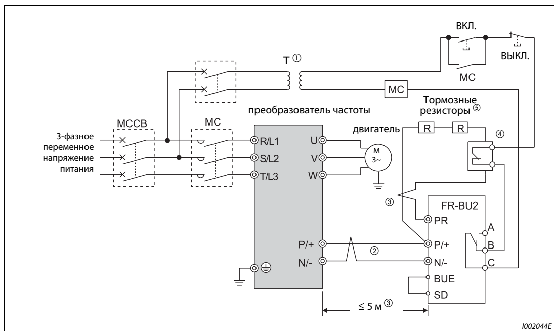
Рис. 3-30: Подключение тормозного устройства типа FR-BU2
