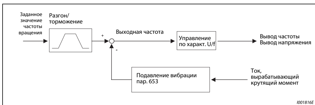
Рис. 6-89: Принцип подавления вибрации
