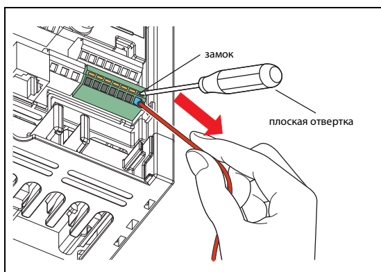
Рис. 3-12: Отсоединение провода
