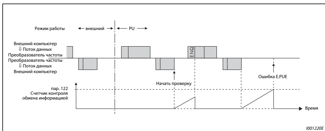
Рис. 6-118: Контроль кабеля на разрыв
