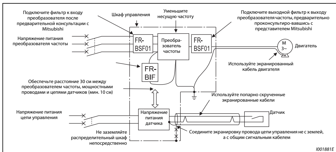
Рис. 3-40: Примеры подавления помех
