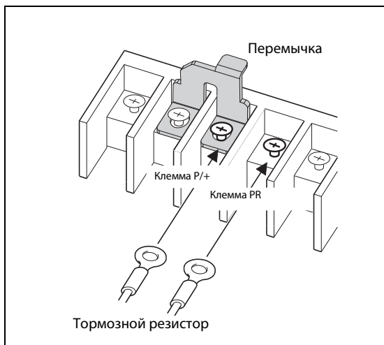
Рис. 3-27: Подключение тормозного резистора к клеммам P/+ и PR преобразователей частоты типов FR-E740-120SC...FR-E740-300SC
