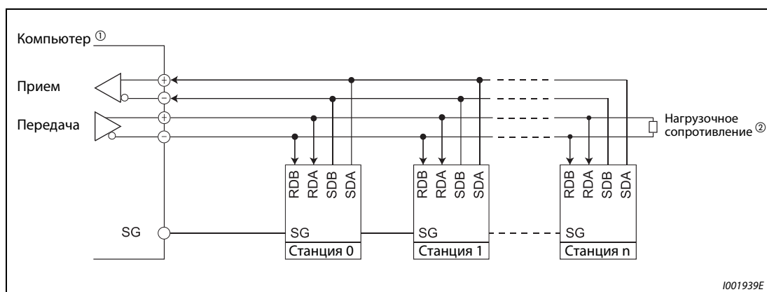
Рис. 6-115: Соединение с несколькими преобразователями частоты
