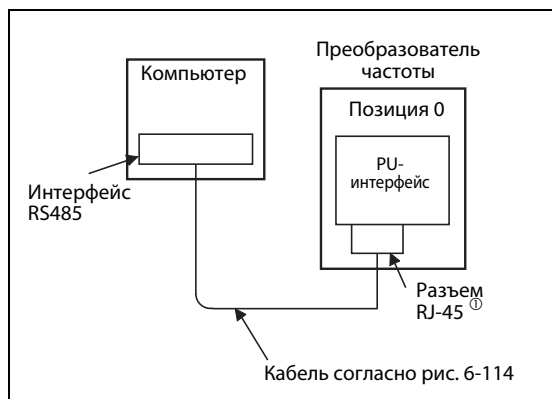
Рис. 6-111: Подключение компьютера с интерфейсом RS485 к интерфейсу PU
