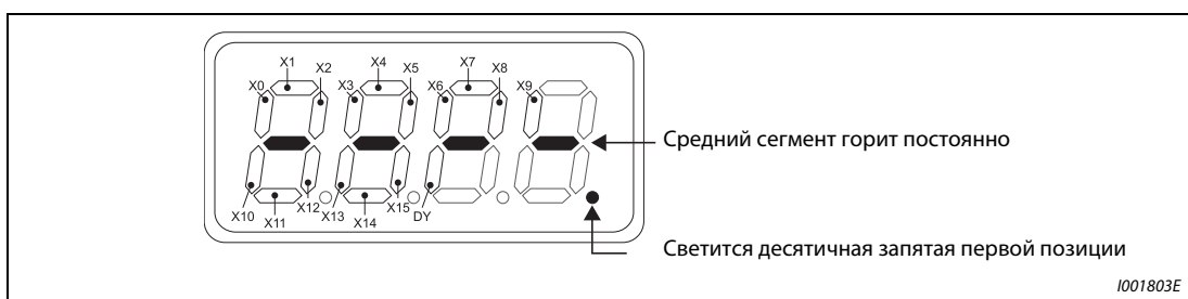
Рис. 6-71: Индикация при установленном дополнительном устройстве FR-A7AX-Ekit-SC-E
