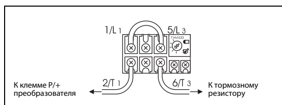
Рис. 3-29: Подключение Термореле
