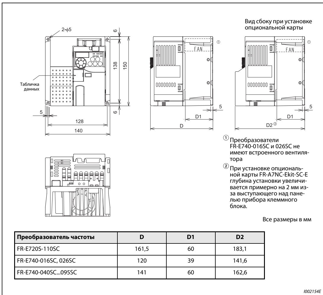
Рис. А-3: Размеры преобразователей частоты FR-E720S-110SC и FR-E740-016SC...095SC
