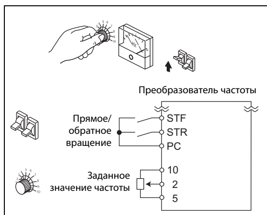
Рис. 6-105: Внешнее управление
