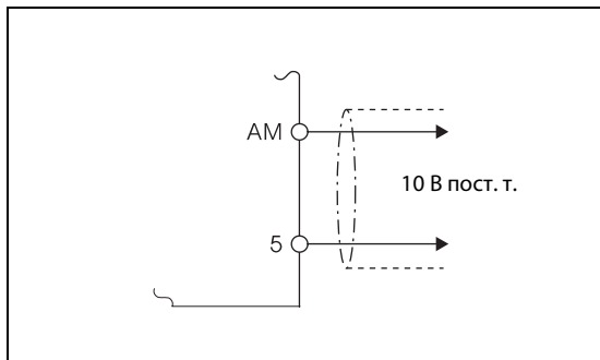
Рис. 6-76: Подключение аналогового индикатора к выходу АМ
