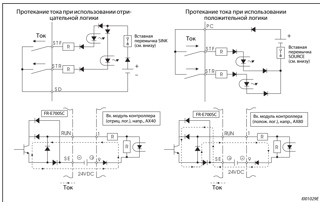
Рис. 3-16: Ток при отрицательной и положительной управляющей логике
