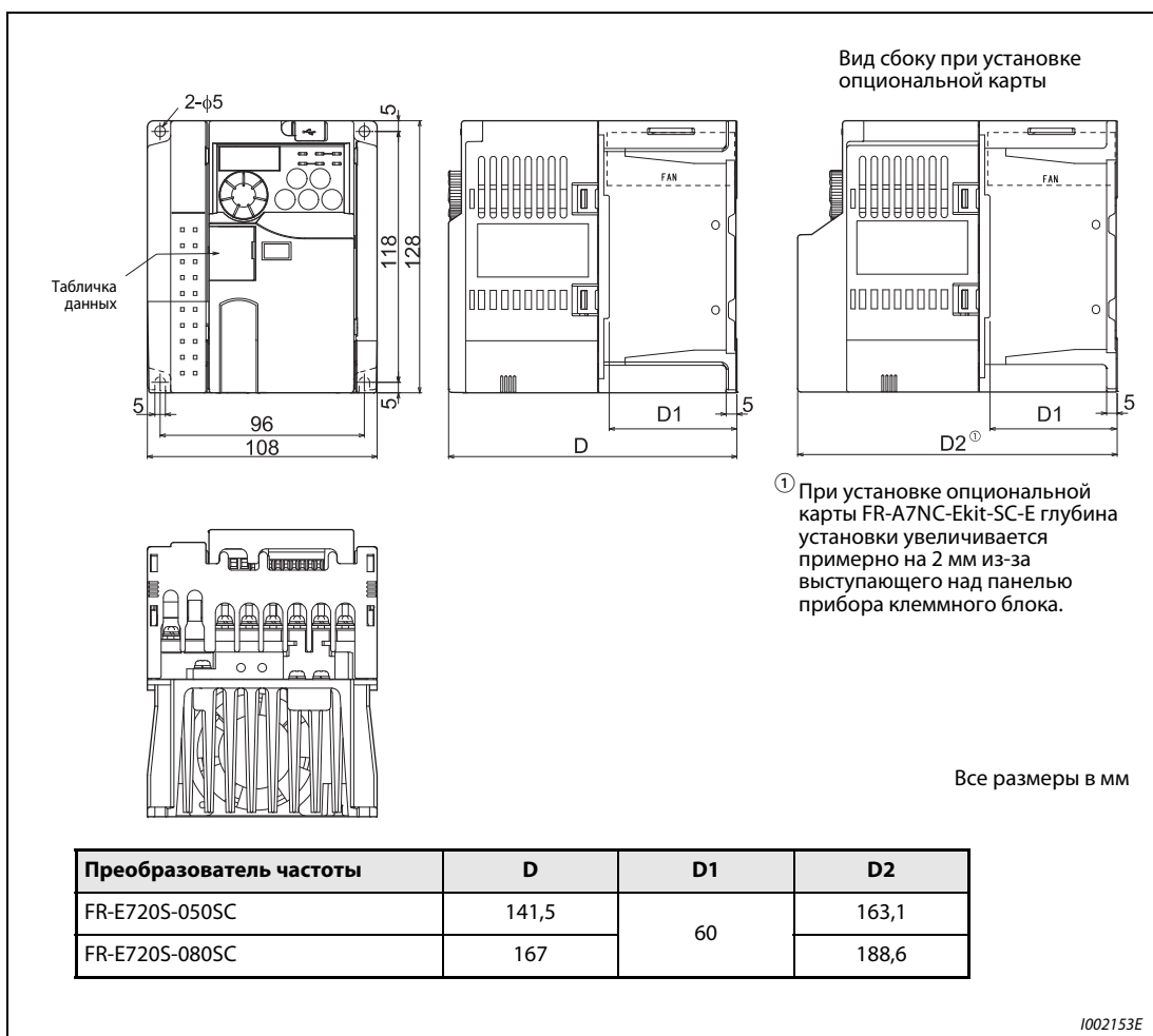
Рис. А-2: Размеры преобразователей частоты FR-E720S-050SC и 080SC
