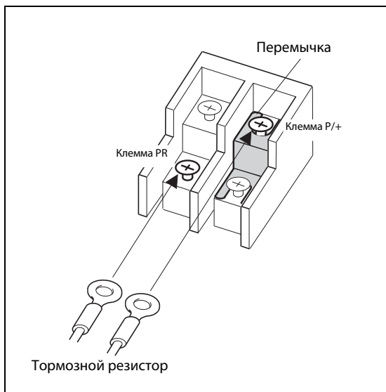
Рис. 3-26: Подключение тормозного резистора к клеммам P/+ и PR преобразователя частоты типа FR-E740-016SC... FR-E740-095SC
