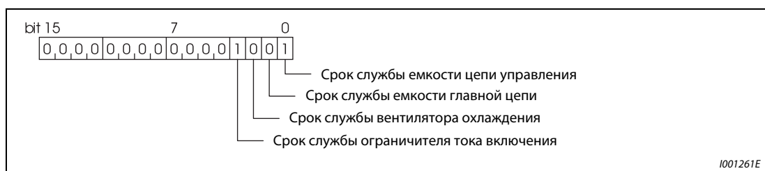
Рис. 6-153: Значение битов параметра 255
