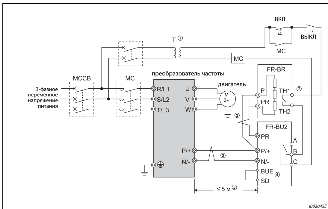
Рис. 3-31: Подключение тормозного блока типа FR-BU2
