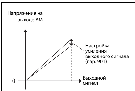
Рис. 6-77: Настройка усиления на выходе АМ
