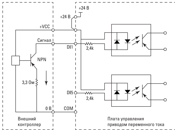
Рис. 3-8. Способ разводки при утечке тока
