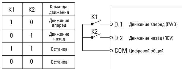
Рис. 6-6. Двухпроводной режим 1
