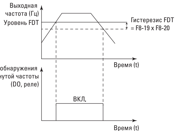
Рис. 6-16. Схема уровня FDT
