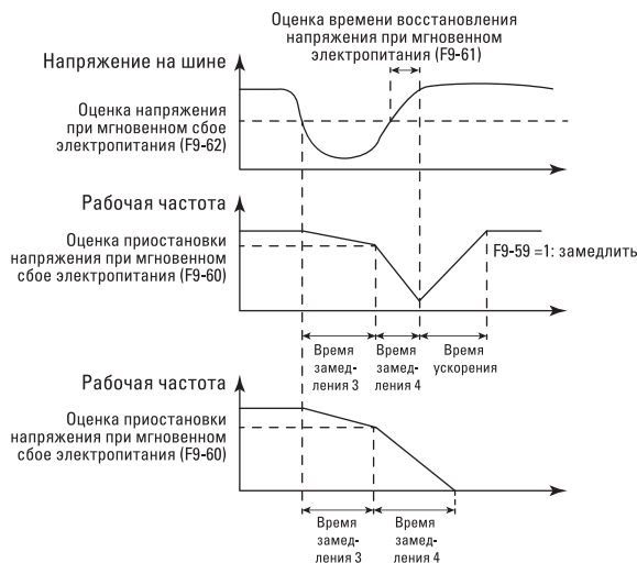
Рис. 6-25. Схема действия при мгновенном сбое электропитания
