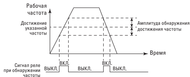
Рис. 6-20. Схема поиска произвольной достигнутой частоты
