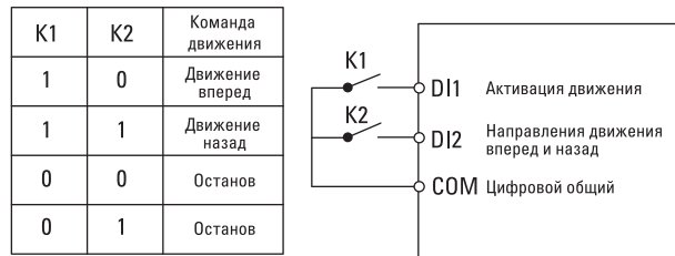
Рис. 6-7. Двухпроводной режим 2
