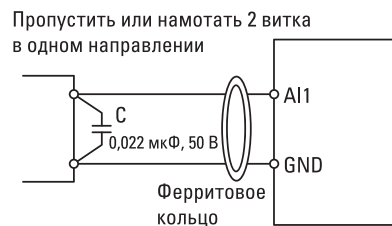
Рис. 3-7. Схема подключения обработки клеммы аналогового входа
