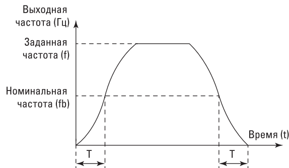
Рис. 6-12. Схема ускорения/замедления В для кривой S
