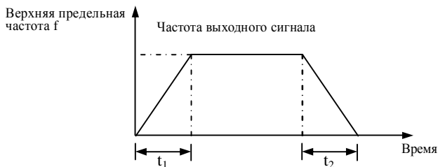
Рисунок 6-5. Время разгона/замедления
