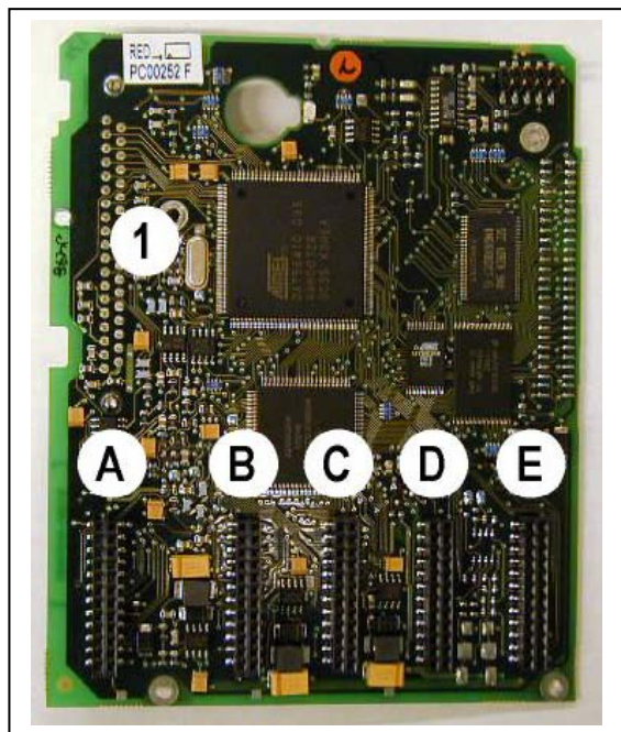
Рисунок 8-1. Плата управления NX
