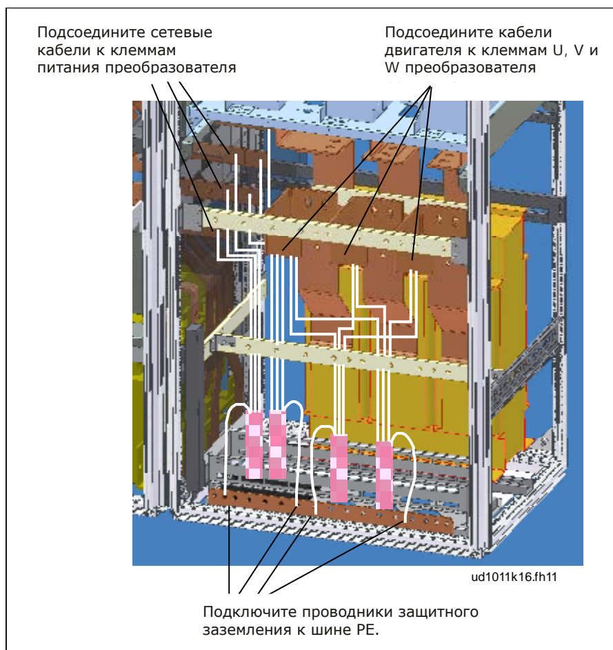
Рисунок 6-9. Разводка силовых кабелей, корпус типоразмера FR14 с подводом кабелей снизу
