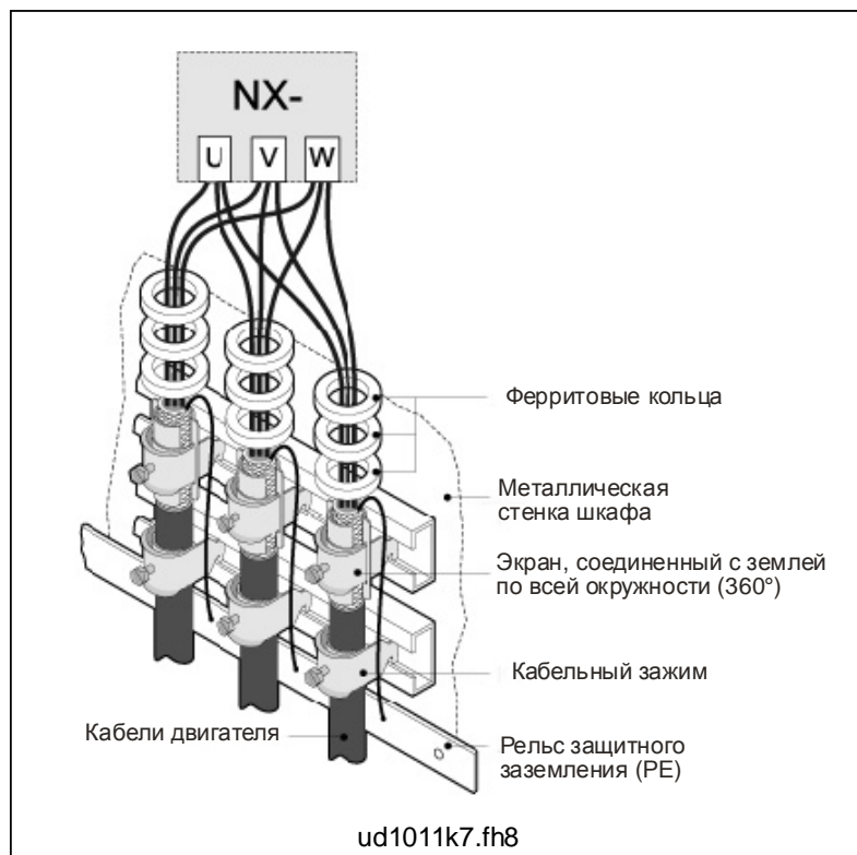
Рисунок 6-16. Установка ферритовых колец
