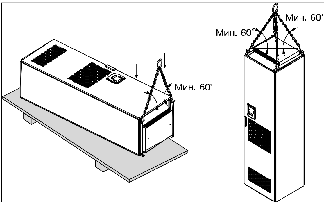
Рисунок 5-2. Подъем устройства
