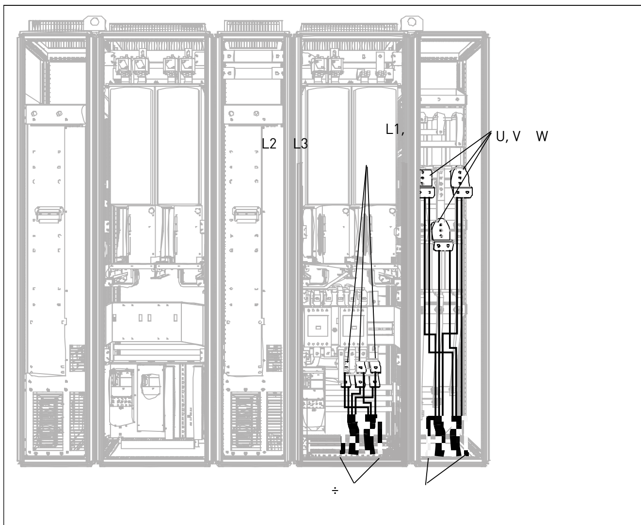
Рисунок 6-11. Разводка силовых кабелей, корпус типоразмера Fi12+ODU (на заказ) с подводом кабелей снизу
