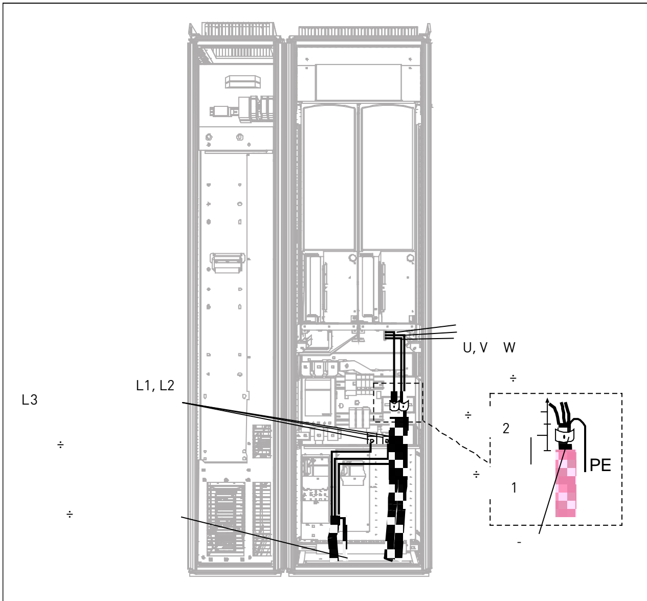
Рисунок 6-10. Разводка силовых кабелей, корпус типоразмера Fi10 с подводом кабелей снизу
