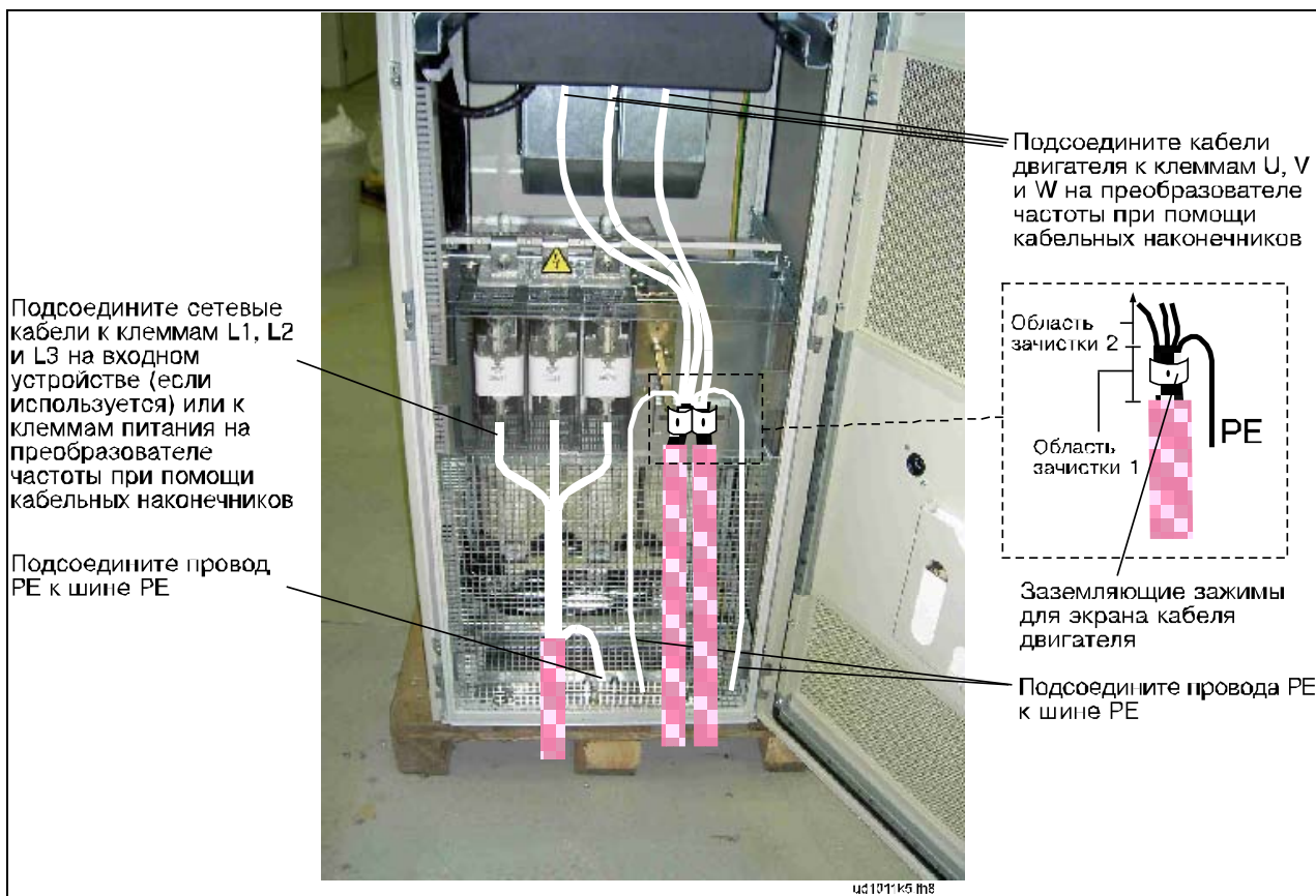
Рисунок 6-7. Прокладка кабелей питания, 6 и 12 пульсов, ввод кабеля снизу для типоразмеров FR10—FR12 (например, FR10+ILS)
