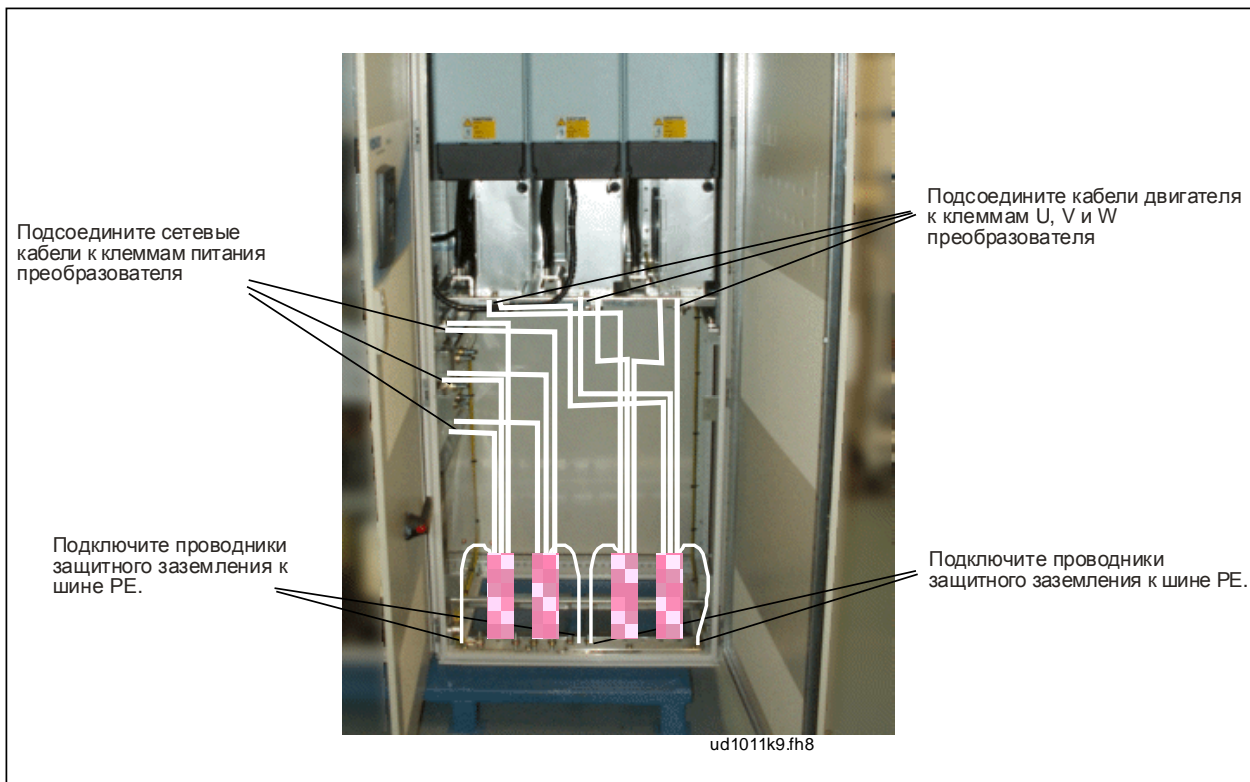
Рисунок 6-8. Прокладка кабелей питания, ввод кабеля снизу для типоразмера FR13
