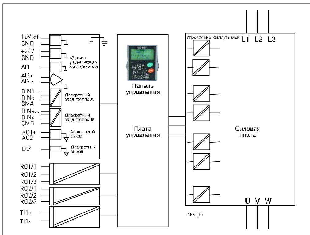
Рисунок 8-6. Гальваническая развязка
