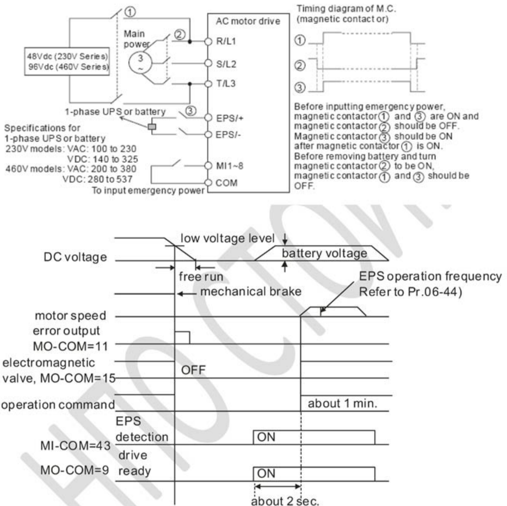
Рис. 2.2 Применение внешних источников напряжением ниже 230 В для питания ПЧ
