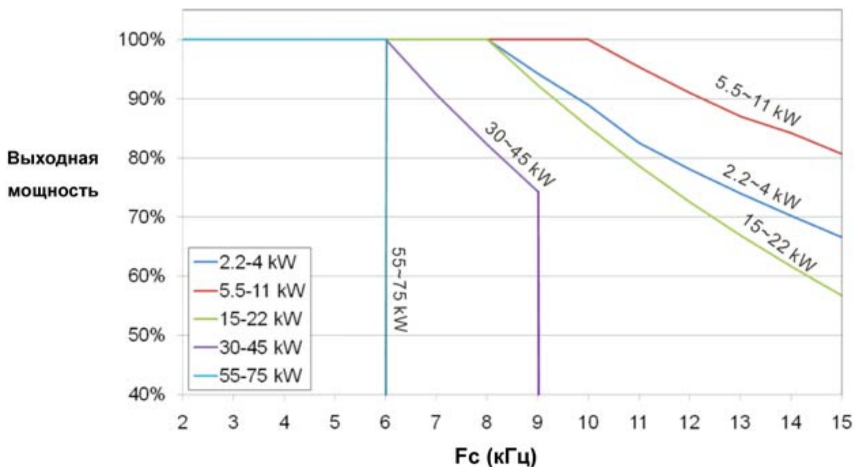
Кривая снижения мощности
