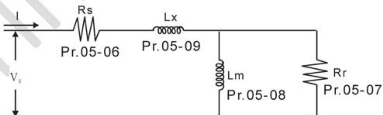
Эквивалентная схема для ПЧ серии VFD-ED
