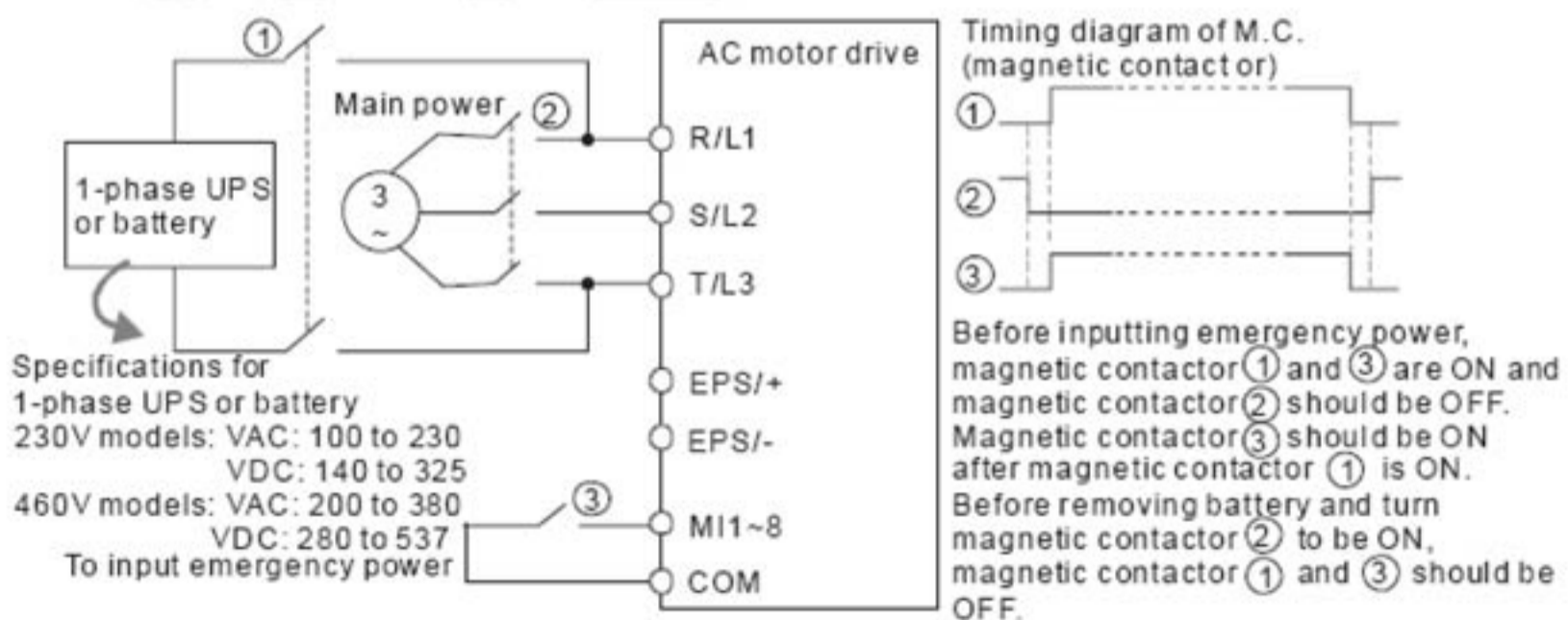
Рис. 2.1 Применение однофазного источника бесперебойного питания
