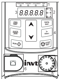
Рис. 6-1 Панель управления
